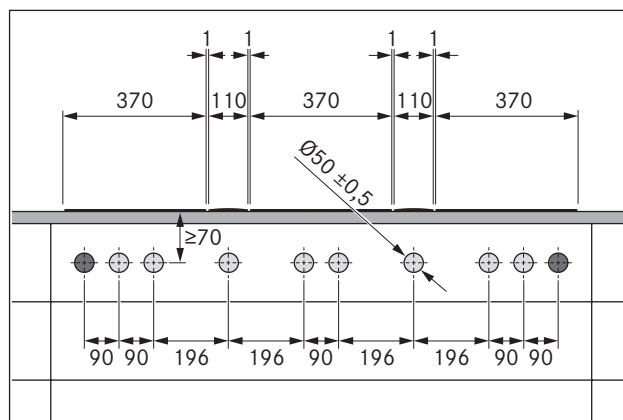
Fig. 5.11 Perfurações do painel em 3 placas de cozinha e 2 extratores
