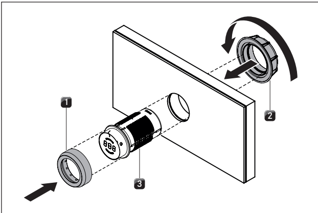
Afb. 5.9 Bedieningsknop monteren
