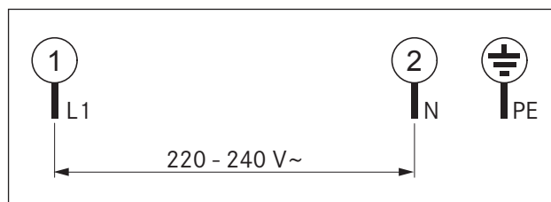
Afb. 5.21 Aansluitschema 1-fasig
