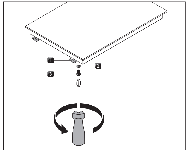
Kuva 5.16 Asennuskannakkeet
