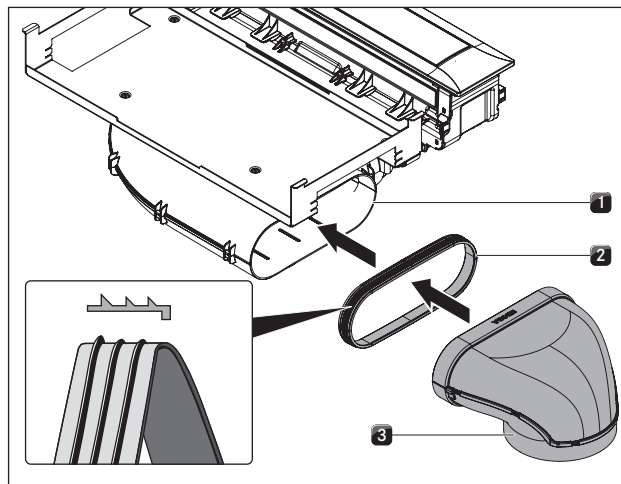
Ilustracja 6.33 Przyłącze systemu kanału
