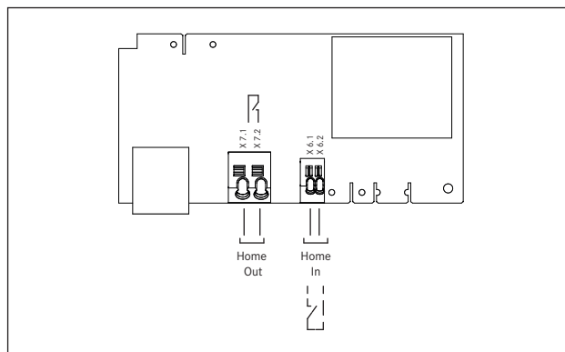
Ilustracja 6.41 Schemat połączeń dla zewnętrznych styków
