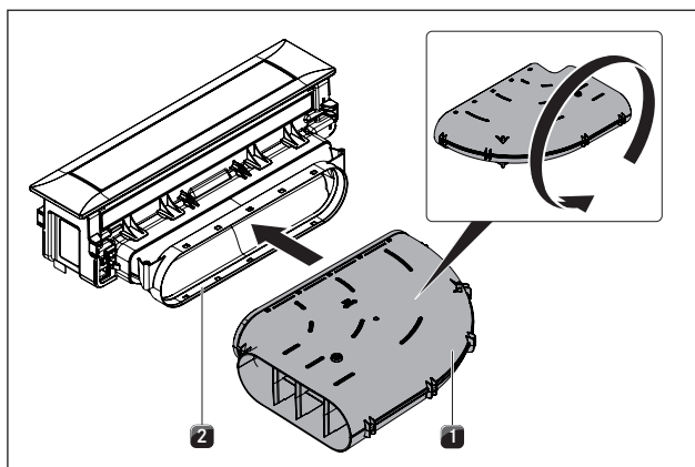
Ilustracja 6.27 Obracanie kształtki wygiętej kanału
