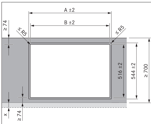
Ilustracja 6.3 Wymiary wycięcia - montaż zlicowany z powierzchnią
