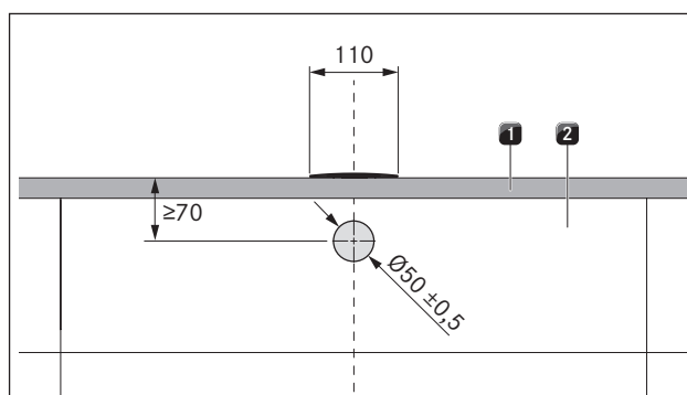
Ilustracja 6.19 Szkic wykonania otworu
