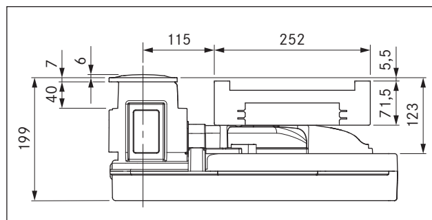
Ilustracja 3.6 PKAS, PKASAB, wymiary urządzenia, widok z przodu
