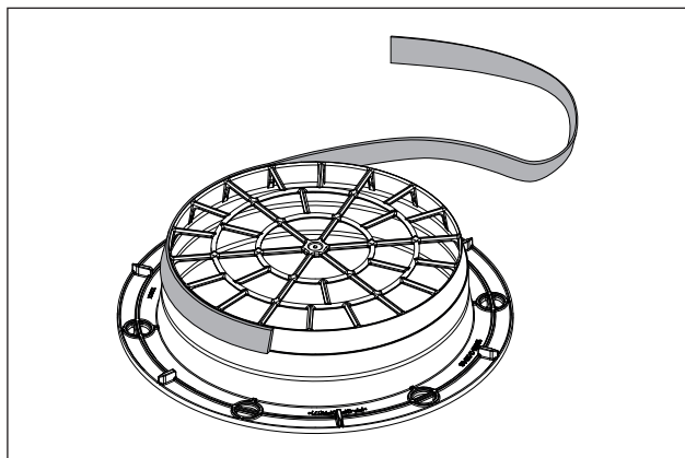
Ilustracja 6.31 Położenie taśmy uszczelniającej przy montażu rury o przekroju okrągłym
