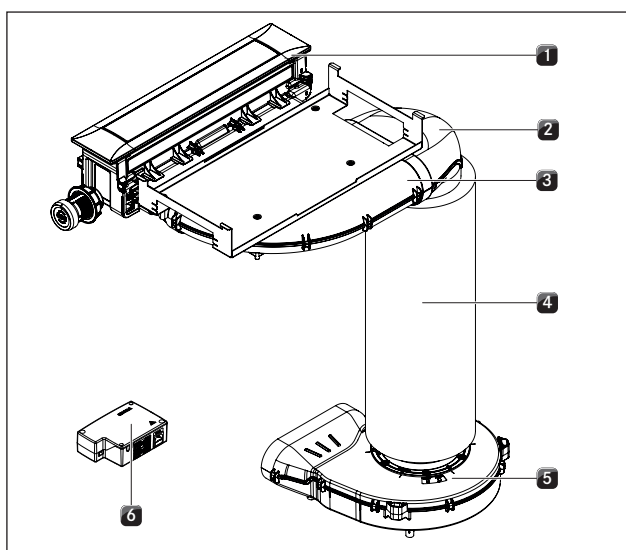
Ilustracja 6.34 Standardowy układ PKA
