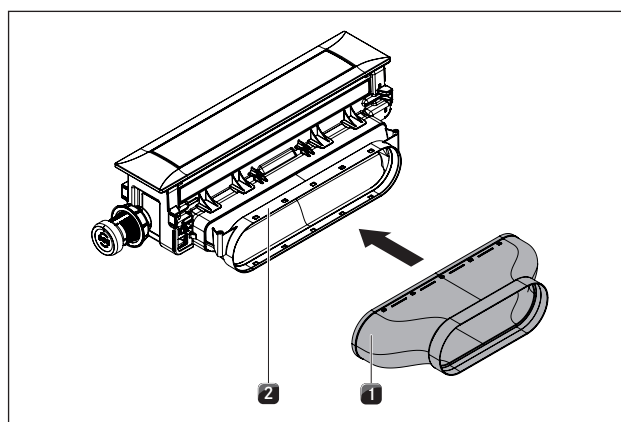
Ilustracja 6.26 Montaż kształtki prostej
