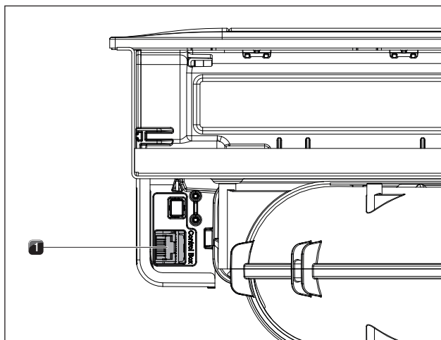
Ilustracja 6.46 Boczne przyłącze na wyciągu oparów PKA do przyłączenia modułu sterowania
