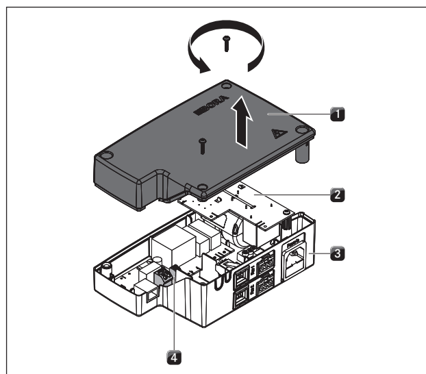
Ilustracja 6.38 Otwieranie pokrywy uniwersalnego modułu sterowania
