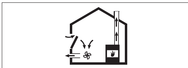
Ilustracja 6.36 Odprowadzenie powietrza – prawidłowe
