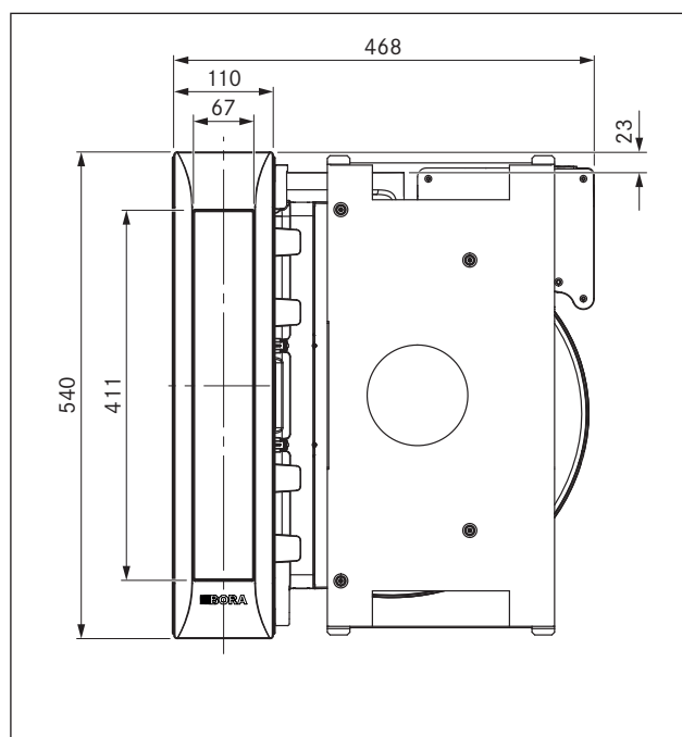
Ilustracja 3.5 PKAS, PKASAB, wymiary urządzenia, rzut
