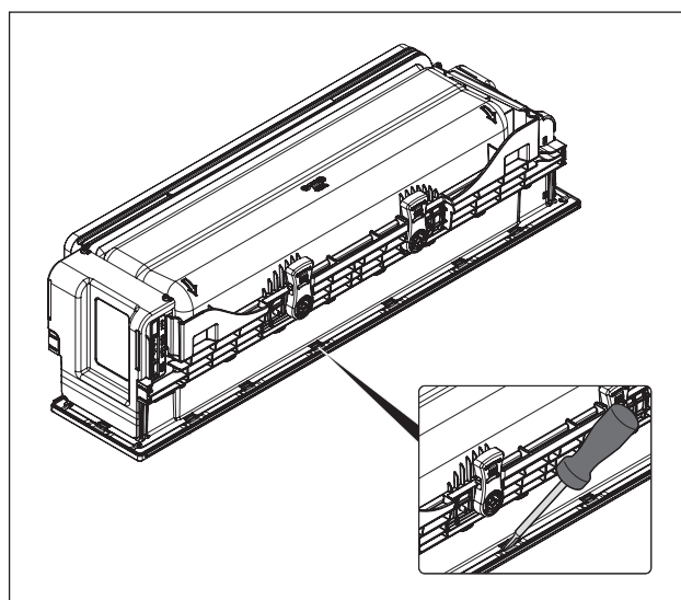
Ilustracja 6.29 Demontaż ramki przykrywającej
