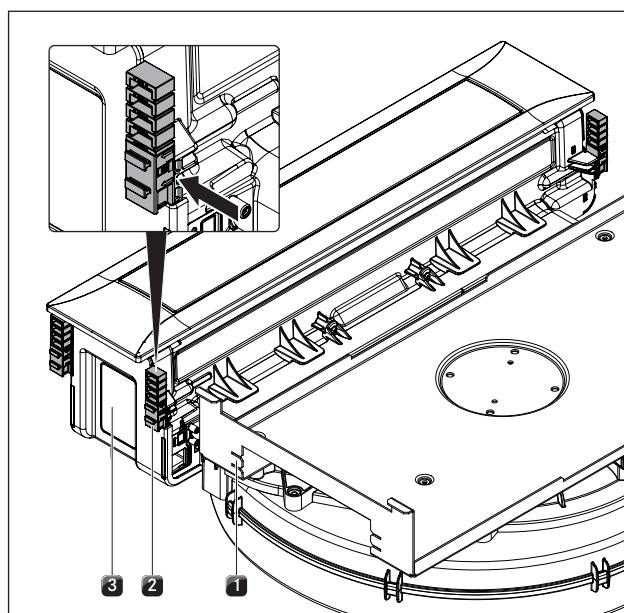
Ilustracja 6.13 Nasuwanie zacisków montażowych
