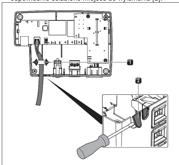
Ilustracja 6.42 Połączenie Home-Out z klamrą zabezpieczającą przed naprężaniem
