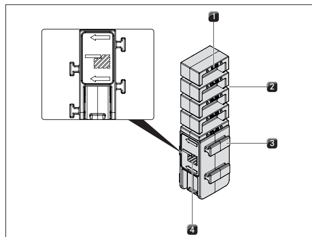
Fig. 6.11 Monteringsklemme høyre side (planlimt montering)
