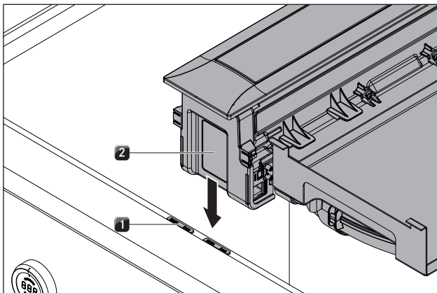
Fig. 6.9 Høydejusteringsplater
