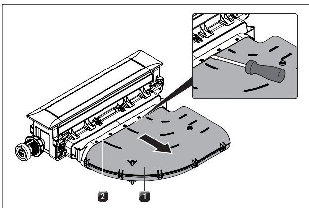
Fig. 6.25 Demontere kanalstykke bøye
