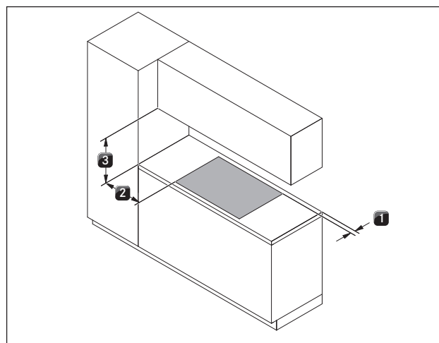
Fig. 6.1 Anbefalte minimumsavstander
