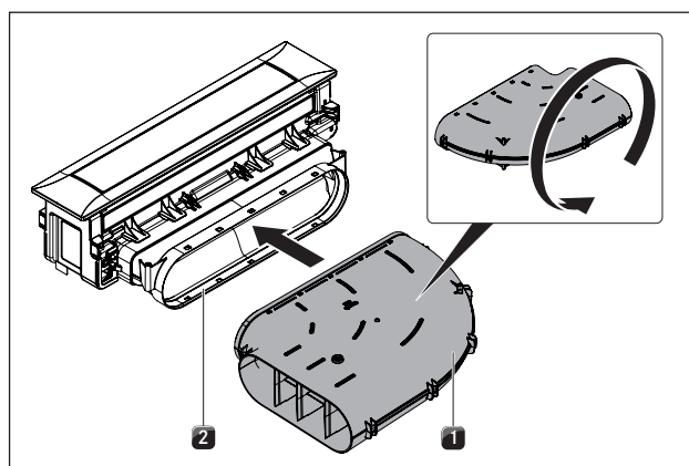
Fig. 6.27 Snu kanalstykke bøye
