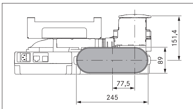
Fig. 6.18 Kanaltilslutningsmål PKAS, PKASAB
