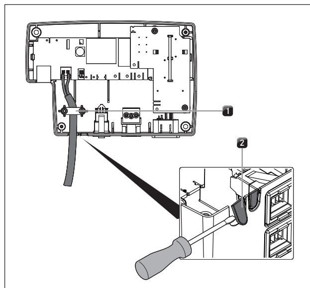
Fig. 6.42 Kontakt Home Out med trækaflastning
