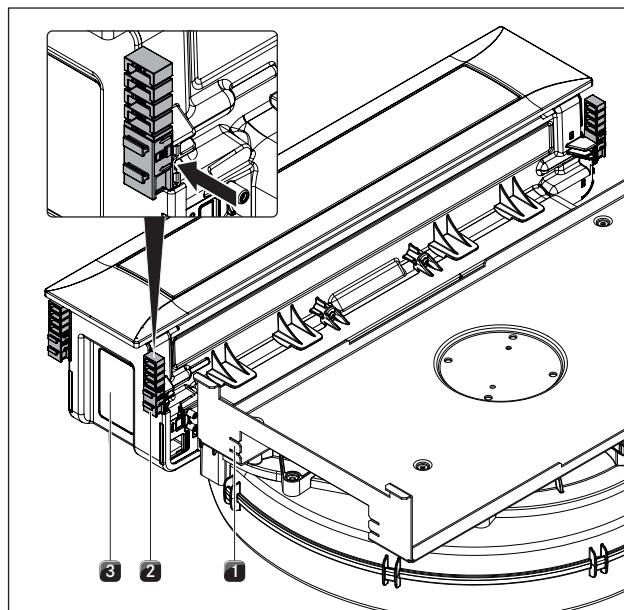
Fig. 6.13 Sådan skubbes monteringsclipsene på
