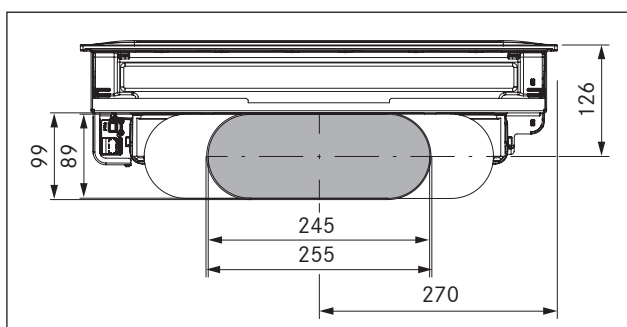
Fig. 6.16 Kanaltilslutningsmål PKA med lige kanalstykke
