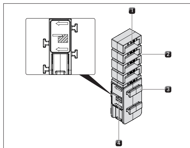
Fig. 6.11 Monteringsclips i højre side (planlimet montering)
