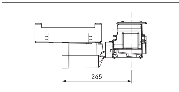
Fig. 6.17 Kanaltilslutningsmål PKA med lige kanalstykke
