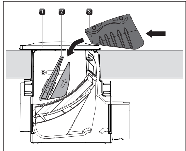
Fig. 8.4 Sådan sættes dækslet i
