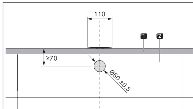
Fig. 6.19 Borebillede
