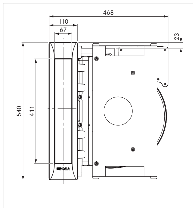
Fig. 3.5 PKAS, PKASAB apparatmål set fra oven
