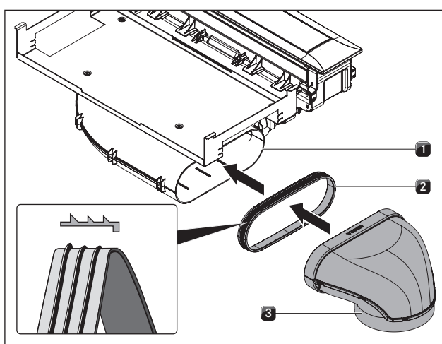
Fig. 6.33 Tilslutning til kanalsystem
