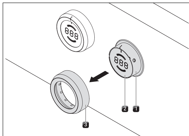
Fig. 8.7 Afmontering af drejeknap
