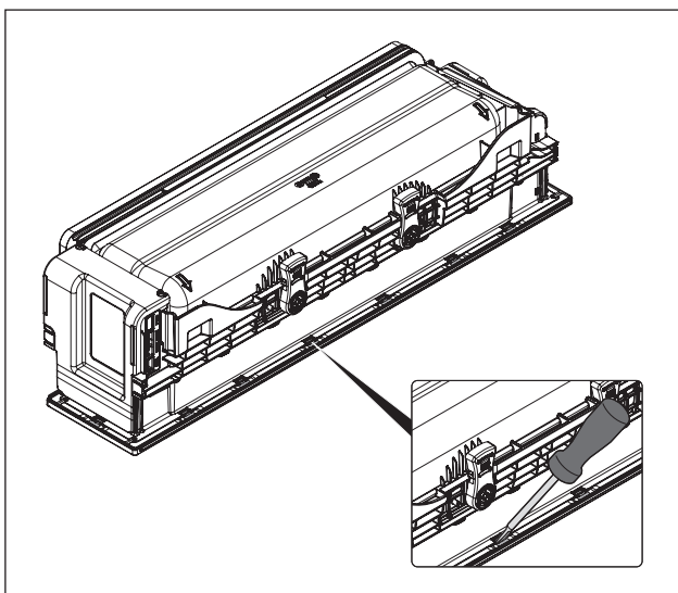
Fig. 6.29 Afmontering af afdækningsramme
