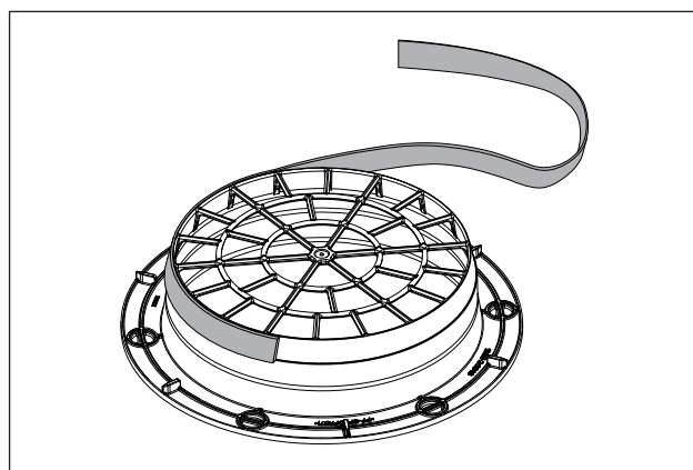
Fig. 6.31 Position på forseglingsstapen til montering med rundrør
