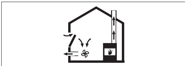
Fig. 6.36 Montering med udsugningsluft – korrekt
