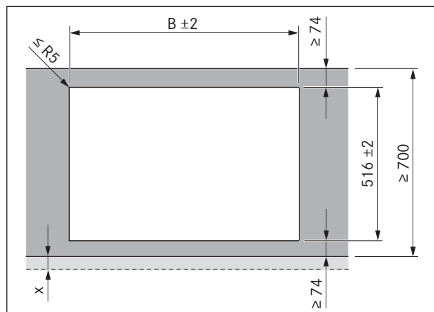
Fig. 6.5 Udskæringsmål overflademontage
