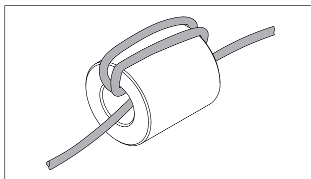
Fig. 6.39 Tilslutningsledningen vikles 3 gange omkring ferritmanchetten
