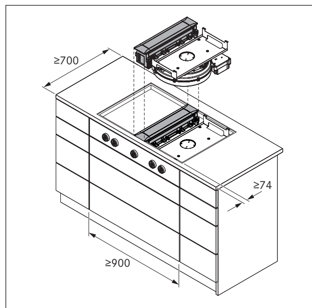
Fig. 6.7 Monteringsmål for apparater PKA og PKAS, PKASAB
