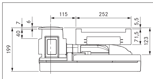
Fig. 3.6 PKAS, PKASAB apparatmål set forfra
