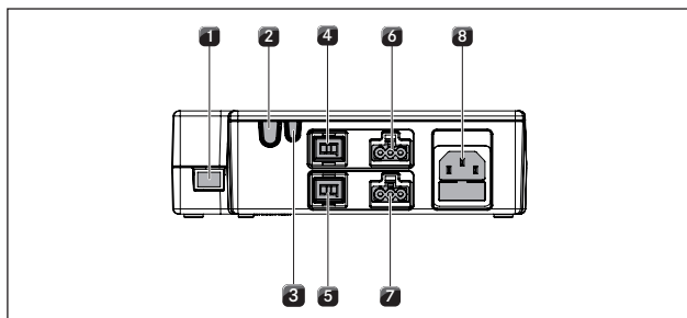
Fig. 6.47 Tilslutninger til universal-styringsenheden
