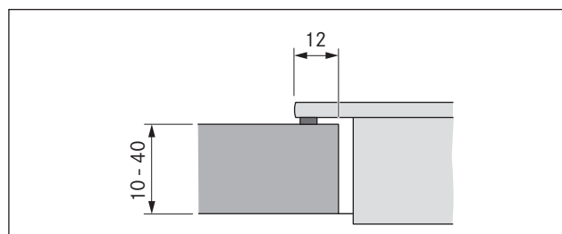
Fig. 6.6 Snit, overflademontage
