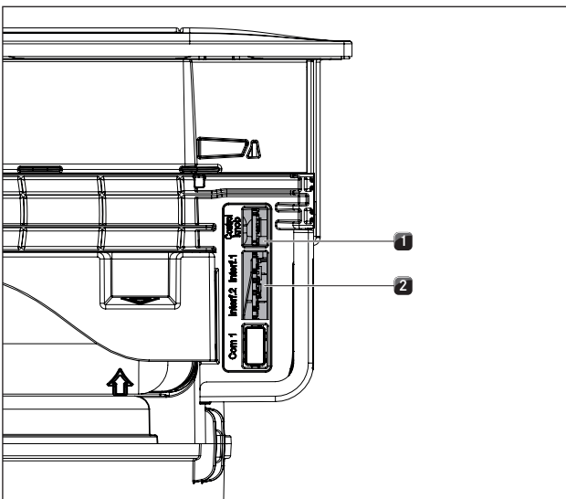
Fig. 6.44 Tilslutninger i siden på emfang
