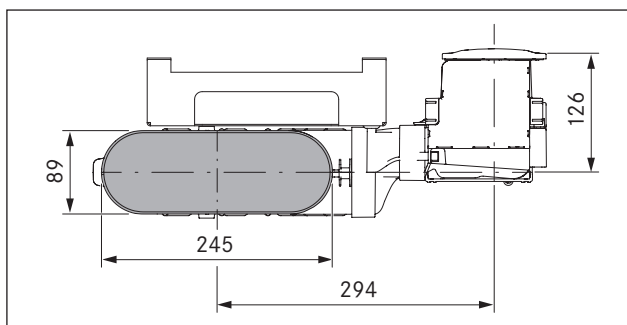
Fig. 6.15 Kanaltilslutningsmål PKA med buet kanalstykke
