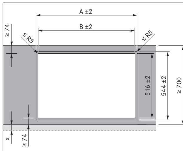
Fig. 6.3 Udkæringsmål planlimet montering
