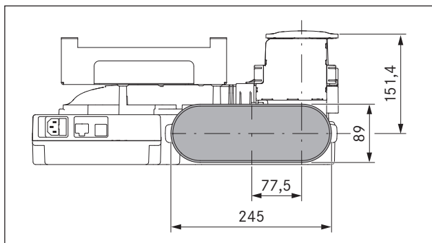
рис. 6.18 Подсоединение канала PKAS, PKASAB
