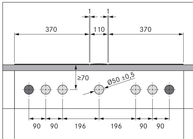
рис. 6.20 Отверстия в передней панели для 2 варочных панелей, 2 розеток и 1 вытяжки
