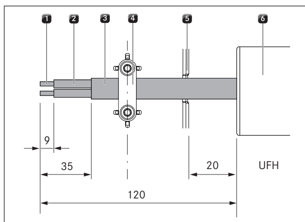
рис. 6.40 Длина изоляции и положение соединительного кабеля при монтаже
