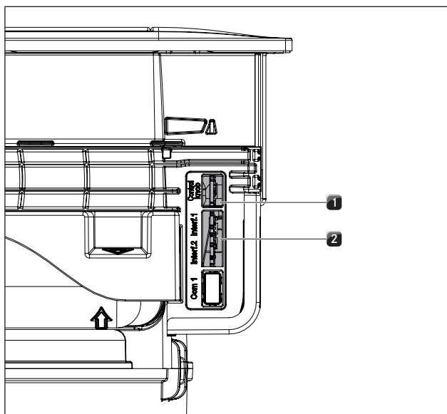
рис. 6.44 Боковые разъемы на вытяжке
