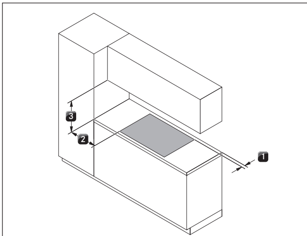
рис. 6.1 Рекомендуемые минимальные расстояния
