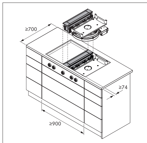
рис. 6.7 Монтажные размеры устройств PKA и PKAS, PKASAB
