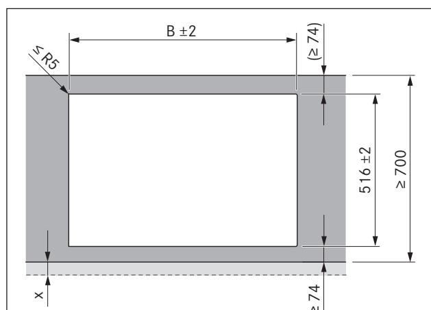
Ilustracja 6.5 Wymiary wycięcia – montaż nakładkowy
