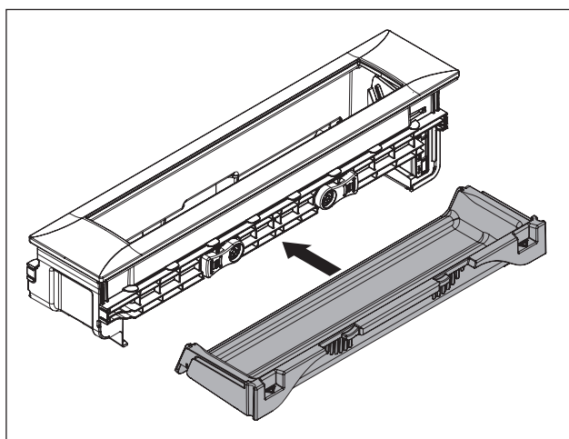
Ilustracja 8.6 Montaż wanienki konserwacyjnej
