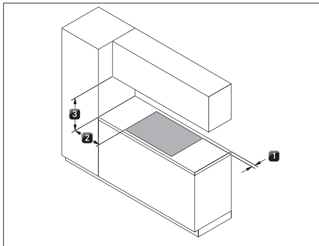
Fig. 6.1 Distanze minime consigliate
