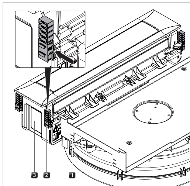
Fig. 6.13 Applicare i morsetti di montaggio
