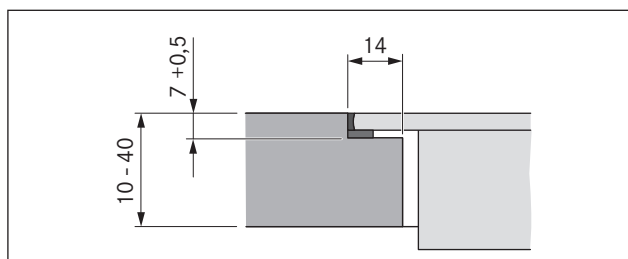
Fig. 6.4 Dimensione dell'incassatura per montaggio a filo piano
