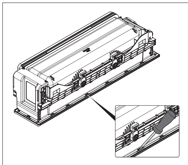
Fig. 6.29 Smontaggio del telaio di copertura
