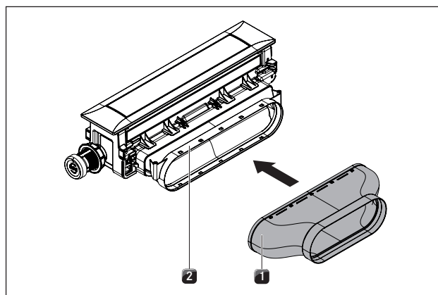
Fig. 6.26 Montare l'elemento canale diritto
