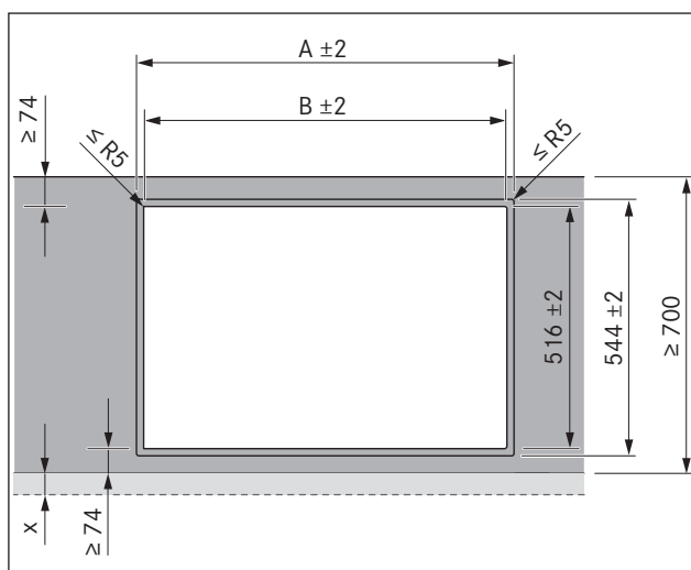
Fig. 6.3 Dimensioni d'intaglio per montaggio a filo piano
