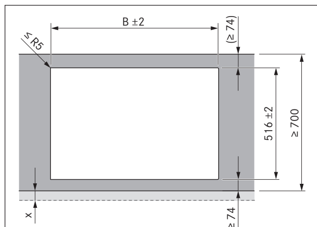
Prikaz 6.5 Dimenzije izreza nadogradnje
