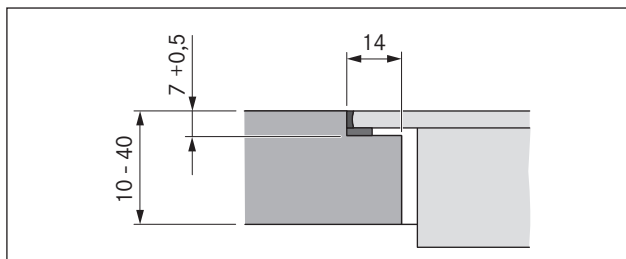
Prikaz 6.4 Dimenzije pregiba za instalaciju u ravni s površinom
