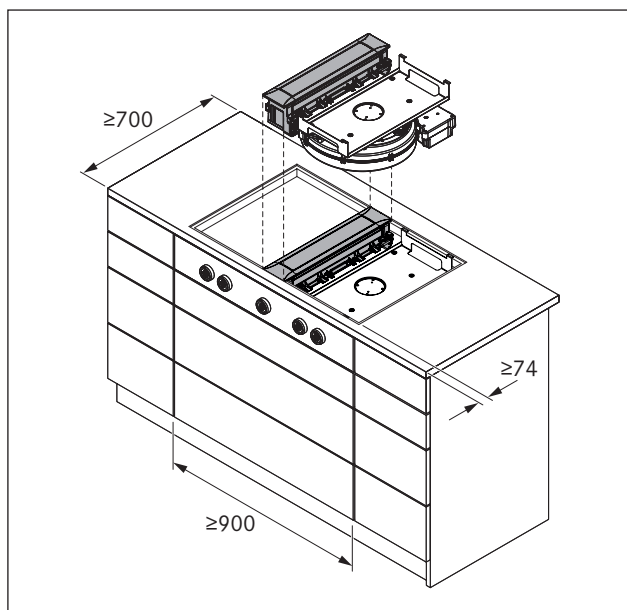
Prikaz 6.7 Dimenzije za ugradnju uređaja PKA i PKAS, PKASAB
