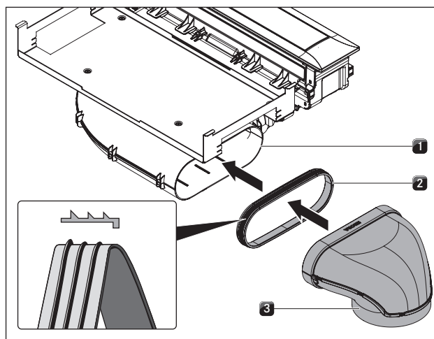
Prikaz 6.33 Priklučivanje na sustav kanala
