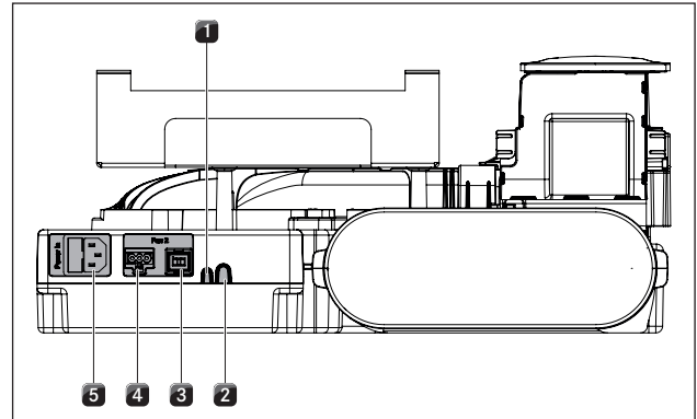
Kuva 6.45 Takaosan liitännät PKAS, PKASAB
