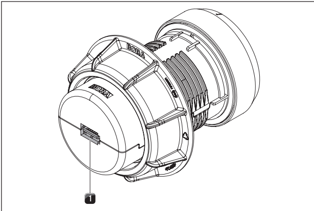
Kuva 6.43 Säätimen takaosan liitäntä
