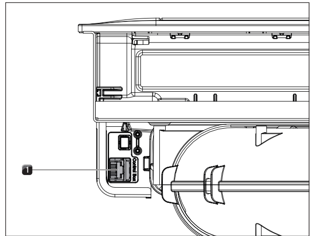
Kuva 6.46 Keittotason höyrynpöiston PKA sivulla sijaitseva ohjausyksikön liitäntä
