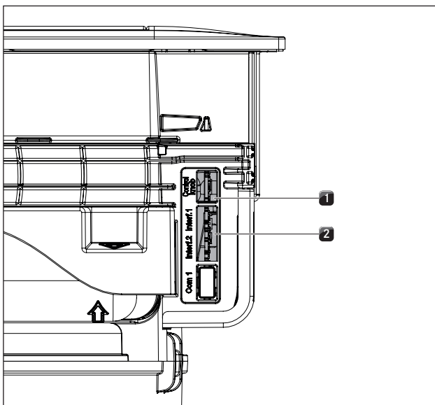
Abb. 6.44 Seitliche Anschlüsse am Kochfeldabzug
