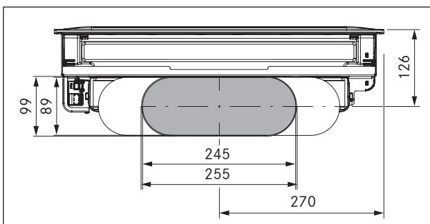
Abb. 6.16 Kanalanschlussmaße PKA mit dem Kanalstück gerade
