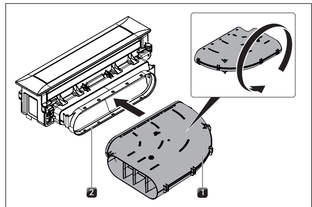
Abb. 6.27 Kanalstück Bogen wenden
