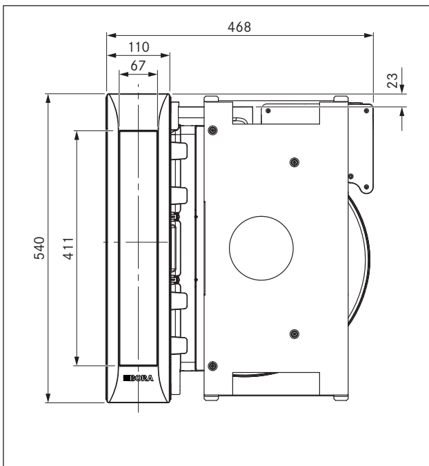
Abb. 3.5 PKAS, PKASAB Gerätemaße Draufsicht
