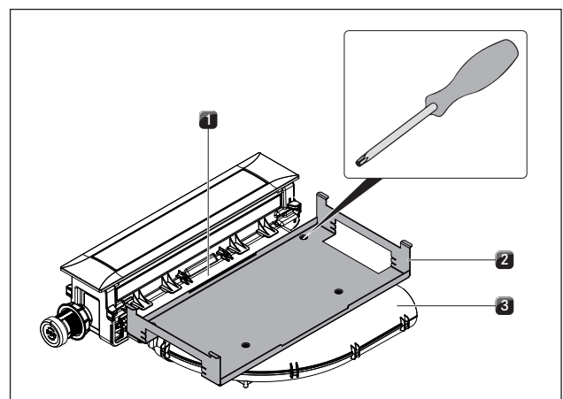
Abb. 6.24 Halblech entfernen
