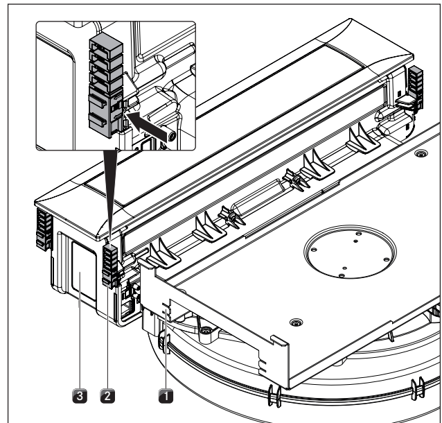
Abb. 6.13 Montageklemmen aufschieben
