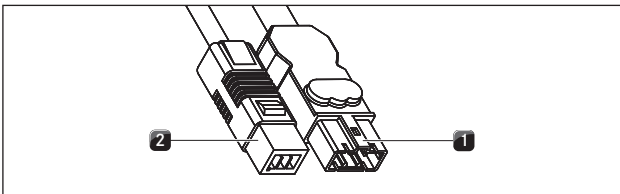
Abb. 6.48 Anschlussstecker des Sockellüfters
