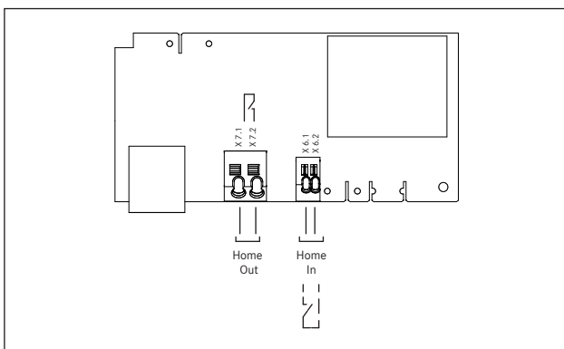
Abb. 6.41 Anschlussschema für externe Schaltkontakte
