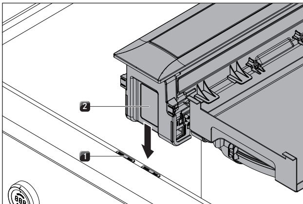
Abb. 6.9 Höhenausgleichsplatten
