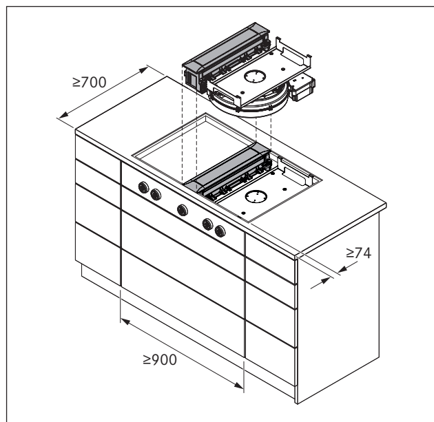
Abb. 6.7 Geräteeinbaumaße PKA ,PKAS und PKASAB
