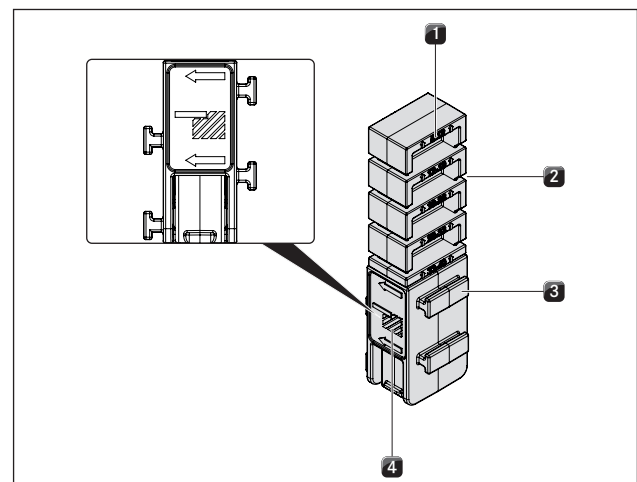
Abb. 6.11 Montageklemme rechte Seite (flächenbündige Montage)
