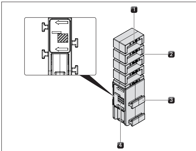
Abb. 6.12 Montageklemme linke Seite (Aufsatzmontage)
