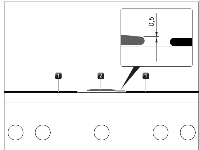
Abb. 6.10 Kochfeldabzug montieren
