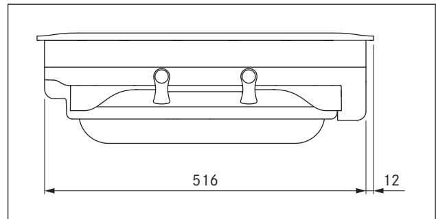
Abb. 3.3 PKA Gerätemaße Seitenansicht
