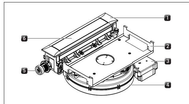
Abb. 5.2 Kochfeldabzugssystem PKAS, PKASAB
