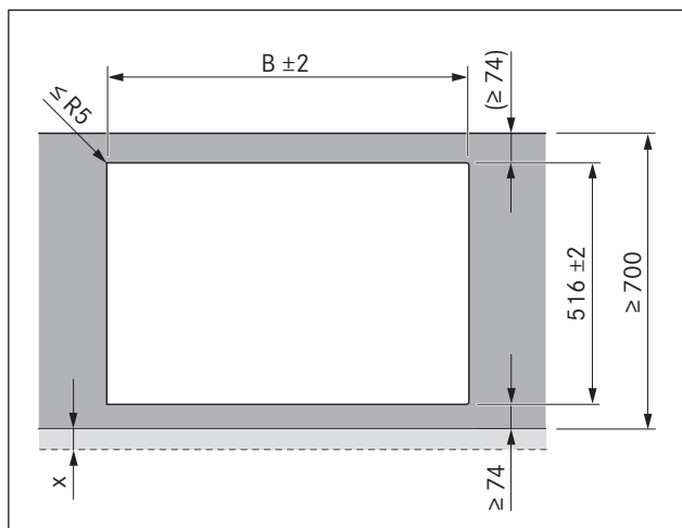
Abb. 6.5 Ausschnittsmaße Aufsatzmontage
