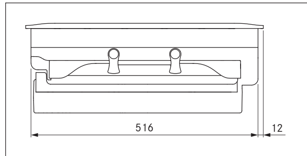
Abb. 3.7 PKAS, PKASAB Gerätemaße Seitenansicht
