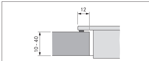
Abb. 6.6 Schnitt Aufsatzmontage
