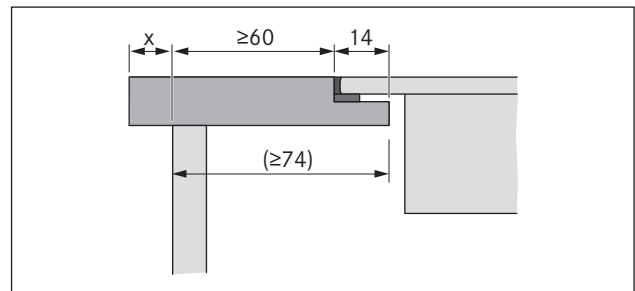
Abb. 6.2 Arbeitsplattenüberstand
