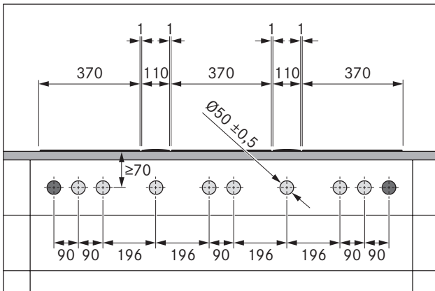
Abb. 6.21 Blendenbohrungen für 3 Kochfelder, 2 Steckdosen und 2 Kochfeldabzüge
