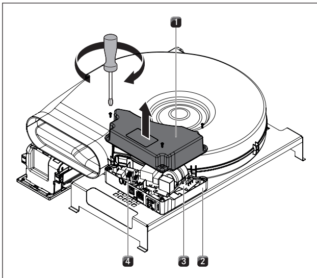
Abb. 6.37 Deckel der Steuerungseinheit öffnen
