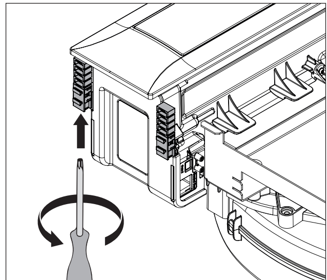
Abb. 6.14 Montageklemmen festziehen
