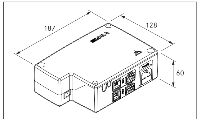
Abb. 3.4 Gerätemaße Universal Steuerungseinheit
