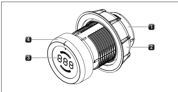
Abb. 5.4 Bedienknebel
