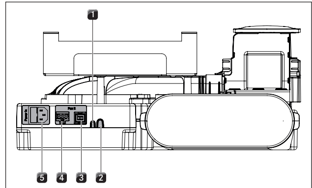
Abb. 6.45 Rückseitige Anschlüsse PKAS und PKASAB
