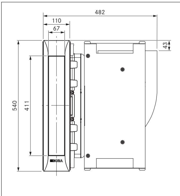
Abb. 3.1 PKA Gerätemaße Draufsicht
