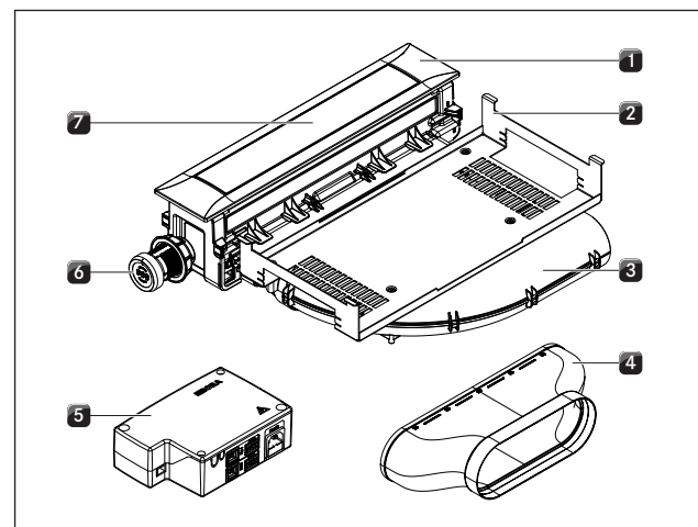
Abb. 5.1 Kochfeldabzug PKA
