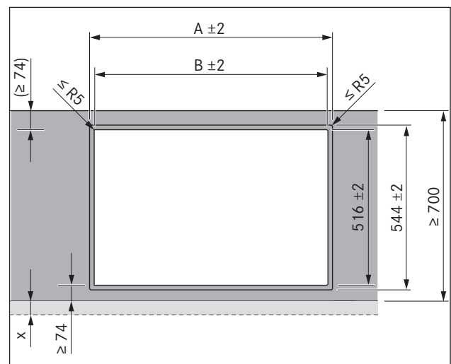
Abb. 6.3 Ausschnittsmaße flächenbündige Montage
