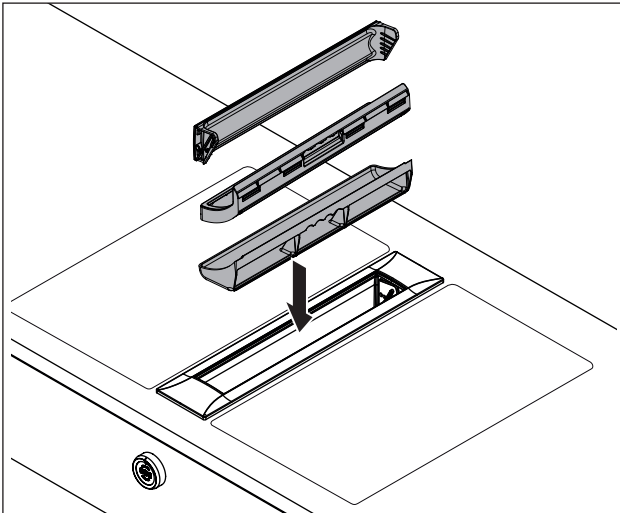
Abb. 8.3 Einbau der Komponenten
