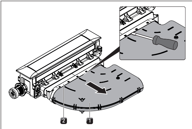
Abb. 6.25 Kanalstück Bogen demontieren
