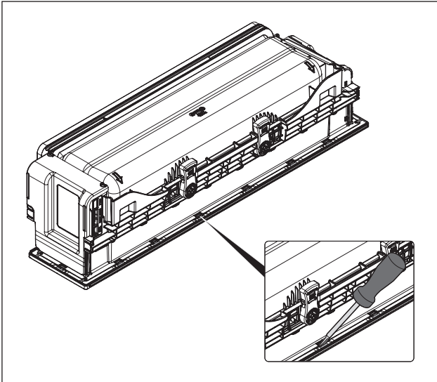
Abb. 6.29 Abdeckrahmen demontieren
