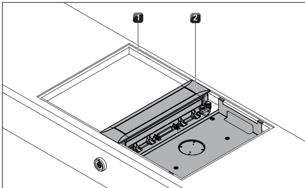
Abb. 6.8 Kochfeldabzug einpassen
