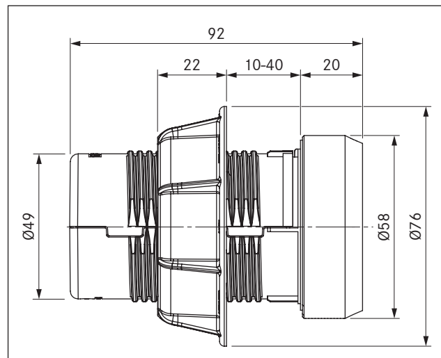
Abb. 3.8 Gerätemaße Bedienknebel
