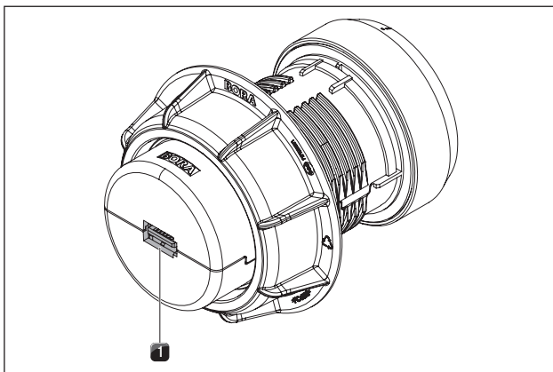
Abb. 6.43 Rückseite Bedienknebel mit Anschluss
