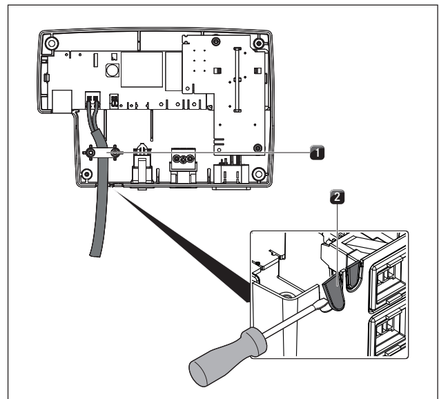
Abb. 6.42 Kontaktierung Home-Out mit Zugentlastung
