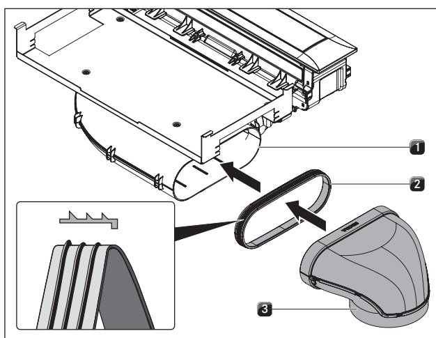
Abb. 6.33 Anschluss an Kanalsystem
