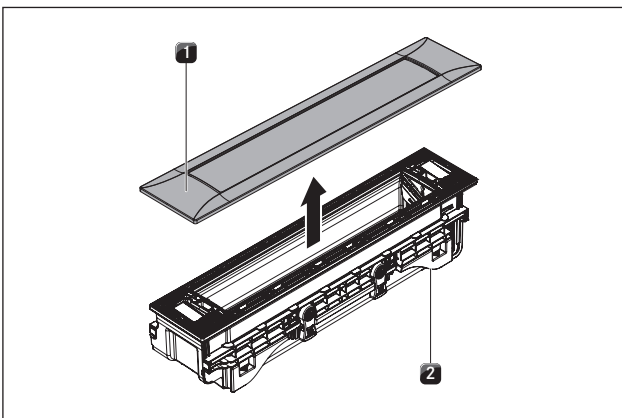
Abb. 6.30 Abdeckrahmen demontieren
