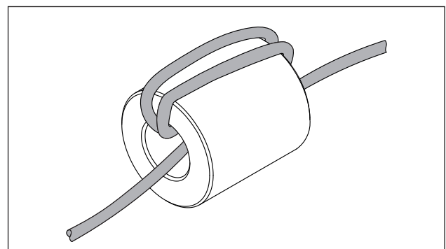
Abb. 6.39 Ferrithülse mit Anschlussleitung 3-fach umwickeln
