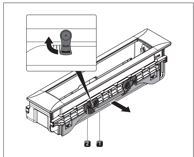
Abb. 8.5 Ausbau der Wartungswanne
