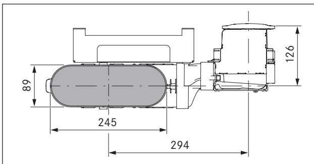
Abb. 6.15 Kanalanschlussmaße PKA mit dem Kanalstück Bogen
