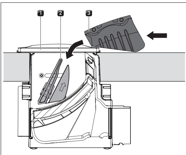
Abb. 8.4 Einsetzen der Verschlussklappe
