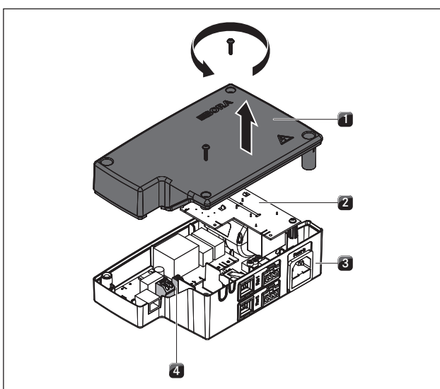
Abb. 6.38 Deckel der Universal Steuerungseinheit öffnen
