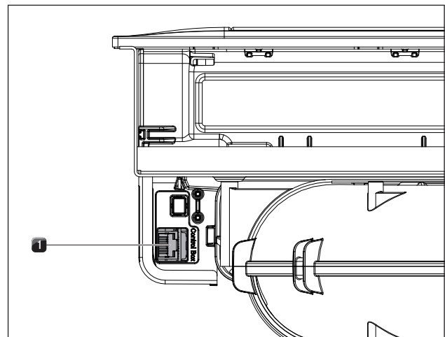
Abb. 6.46 Seitlicher Anschluss für die Steuerungseinheit am Kochfeldabzug PKA
