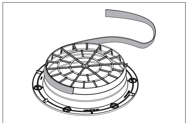
Abb. 6.31 Position des Dichtungsbands für Montage mit Rundrohr
