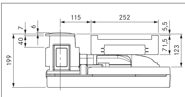
Abb. 3.6 PKAS, PKASAB Gerätemaße Vorderansicht
