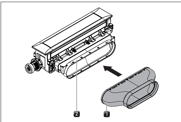
Abb. 6.26 Kanalstück gerade montieren
