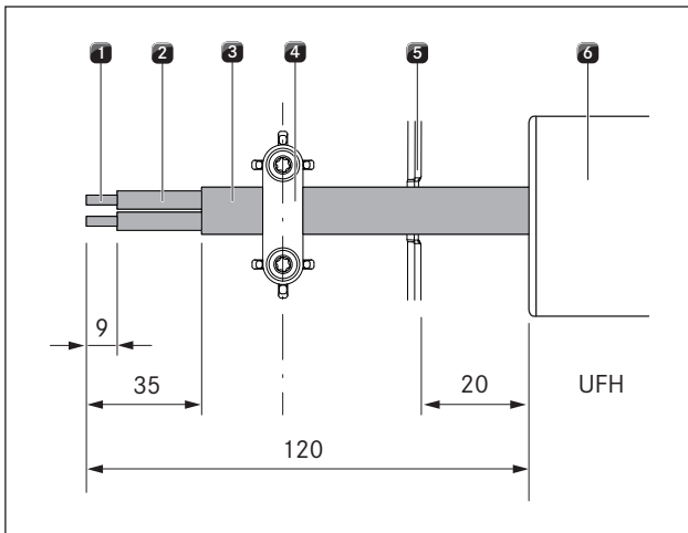
Abb. 6.40 Abisolierlängen und Montageposition der Anschlussleitung
