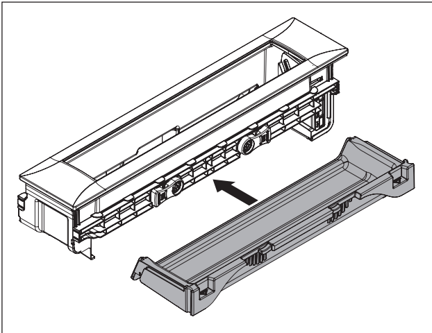
Abb. 8.6 Einbau der Wartungswanne
