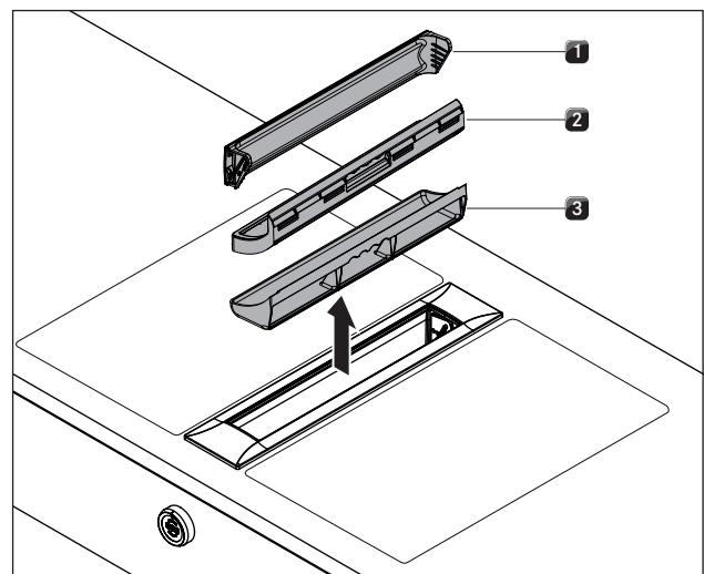
Abb. 8.2 Ausbau der Fettfilter-Komponenten
