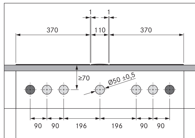
Abb. 6.20 Blendenbohrungen für 2 Kochfelder, 2 Steckdosen und 1 Kochfeldabzug
