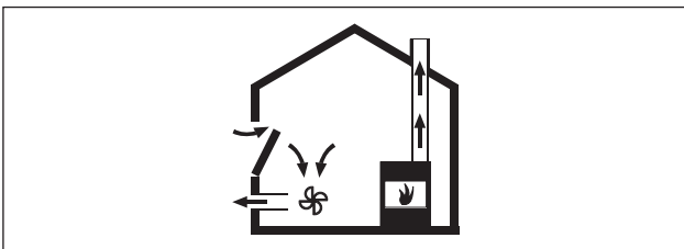
Abb. 6.36 Abluftmontage – korrekt
