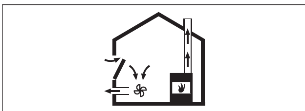
Fig. 6.36 Montering med udsugningsluft – korrekt
