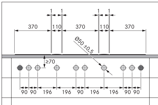
Fig. 6.21 Pladeborehuller til 3 kogeplader, 2 stikdåser og 2 emfang
