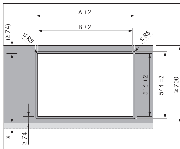
Fig. 6.3 Udskæringsmål planlimet montering
