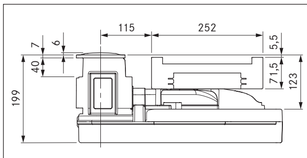
Fig. 3.6 PKAS, PKASAB apparatmål set forfra
