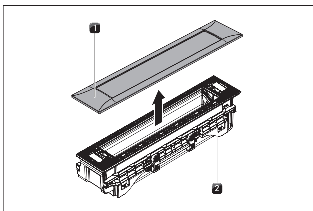
Fig. 6.31 Démontez le cadre de recouvrement
