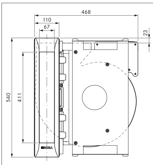
Fig. 3.5 Dimensions PKAS, PKASAB vue du dessus
