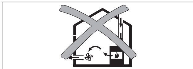
Fig. 6.36 Le montage du circuit - non autorisé
