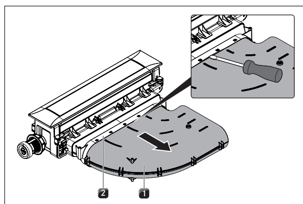
Fig. 6.26 Démontez le coude de section
