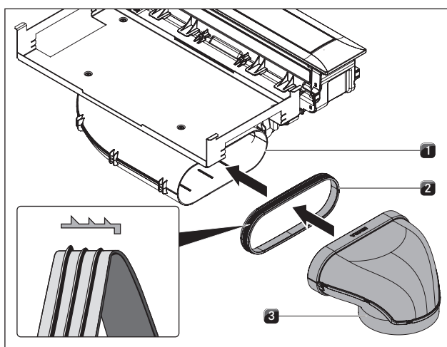
Fig. 6.34 Raccordement au système de canaux
