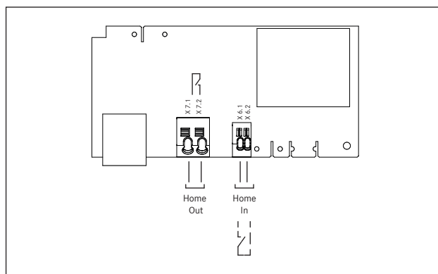
Fig. 6.42 Schéma de raccordement pour contacts de commutation externes
