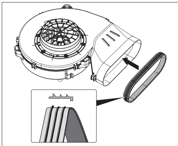
Fig. 6.33 Mettez en place les joints des manchons de sortie du ventilateur de socle
