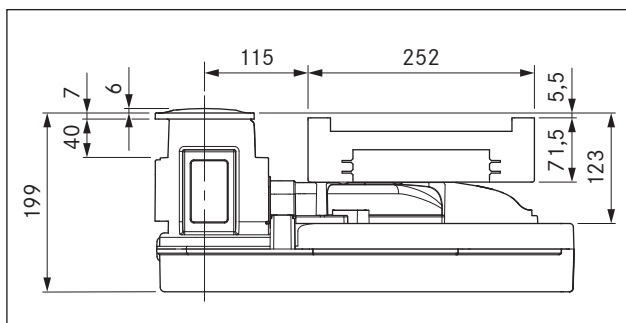
Fig. 3.6 Dimensions PKAS, PKASAB vue de face
