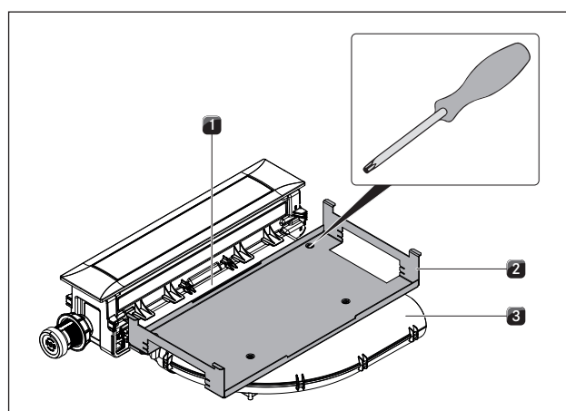
Fig. 6.25 Retirez la plaque de maintien
