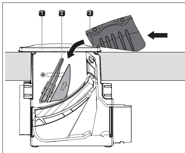
Fig. 8.4 Ouverture d'aspiration
