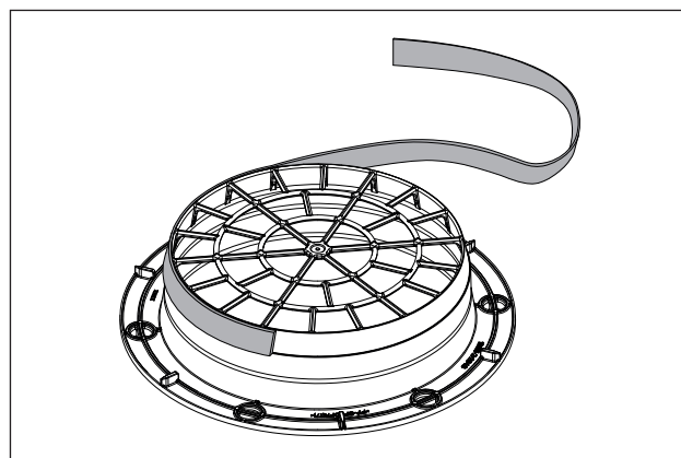
Fig. 6.32 Position du joint pour montage avec tube rond
