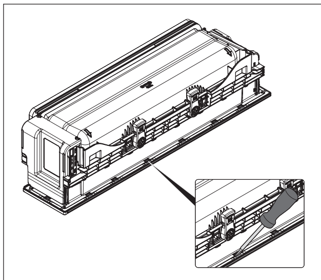
Fig. 6.30 Démontez le cadre de recouvrement
