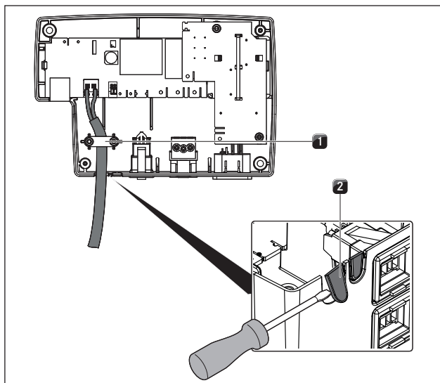
Fig. 6.43 Connexion « Home Out » avec serre-câble
