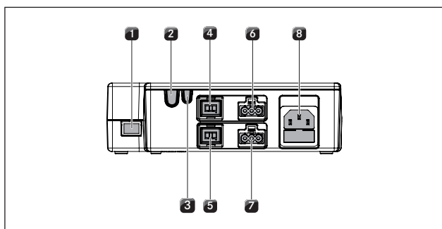
Fig. 6.48 Raccordement de l'unité de commande universelle
