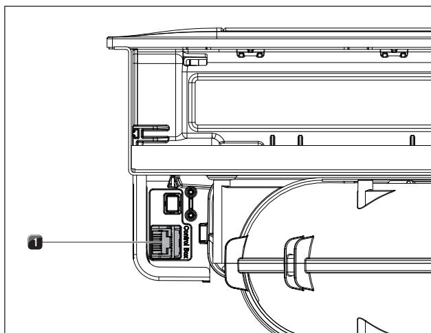
Fig. 6.47 Raccordements latéraux pour l'unité de commande universelle du dispositif d'aspiration PKA
