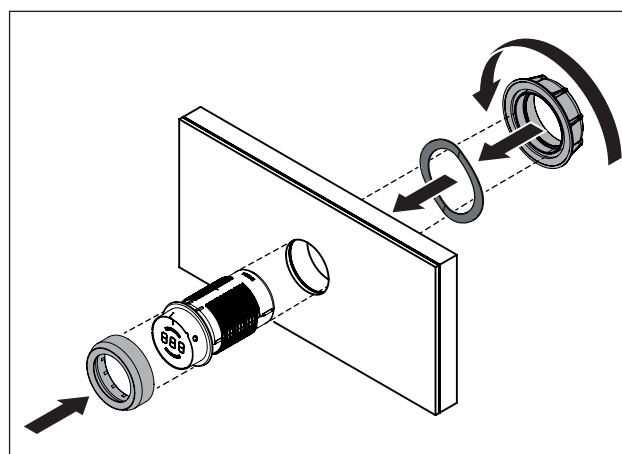
Fig. 6.23 Montez le bouton de commande
