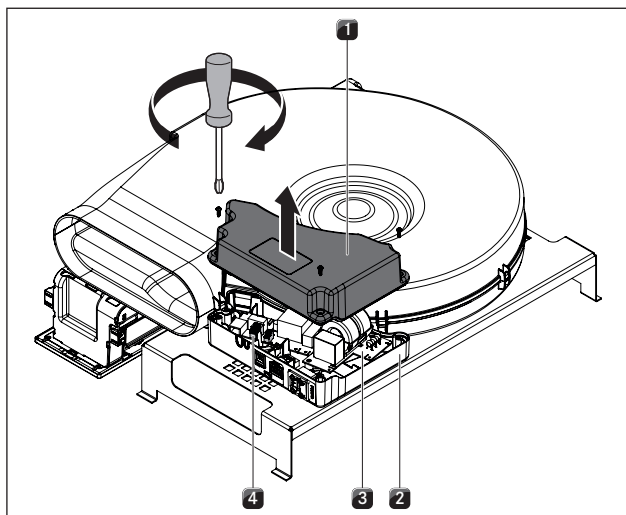
Fig. 6.38 Ouvrez le couvercle de l'unité de commande
