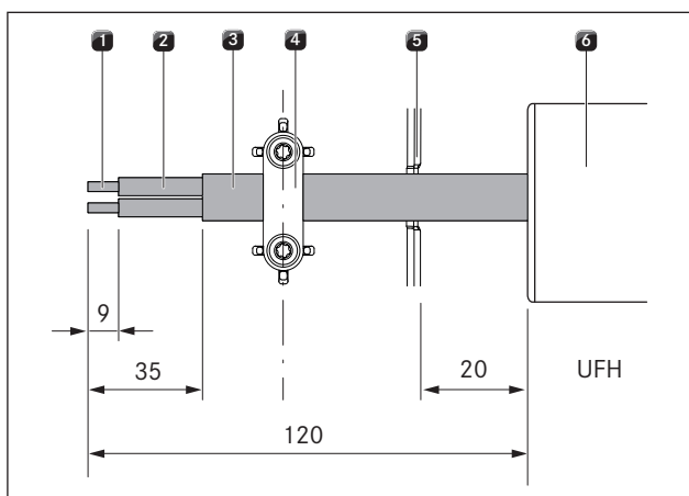
Fig. 6.41 Longueurs de dénudage et position de montage de la fiche de raccordement
