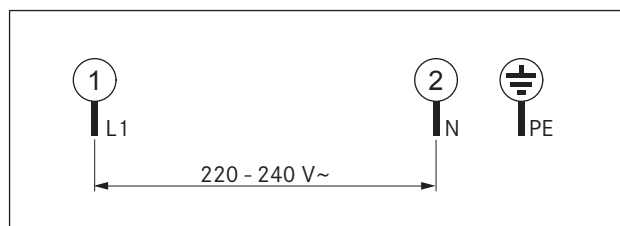
Fig. 5.17 Tilslutningsskema, 1-faset
