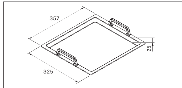
Sl. 1.1 Dimenzije (brez ročajev)
