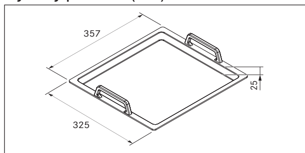
Ilustracja 1.1 Wymiary (bez uchwytów)
