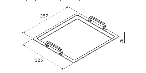
Obr. 1.1 Rozměry (bez držadel)
