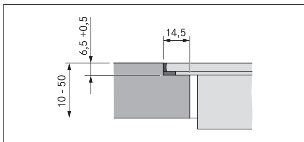
bild 6.3 Falsmått för planmonteringen
