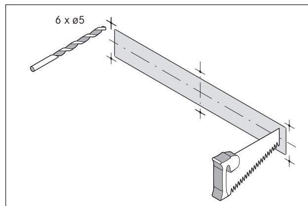
bild 6.10 Utskärning och anslutningshål
