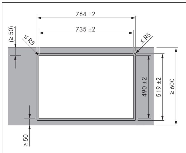
bild 6.2 Utskärningsmått för planmonteringen
