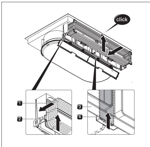
bild 6.14 Haka i flexkanalens ram
