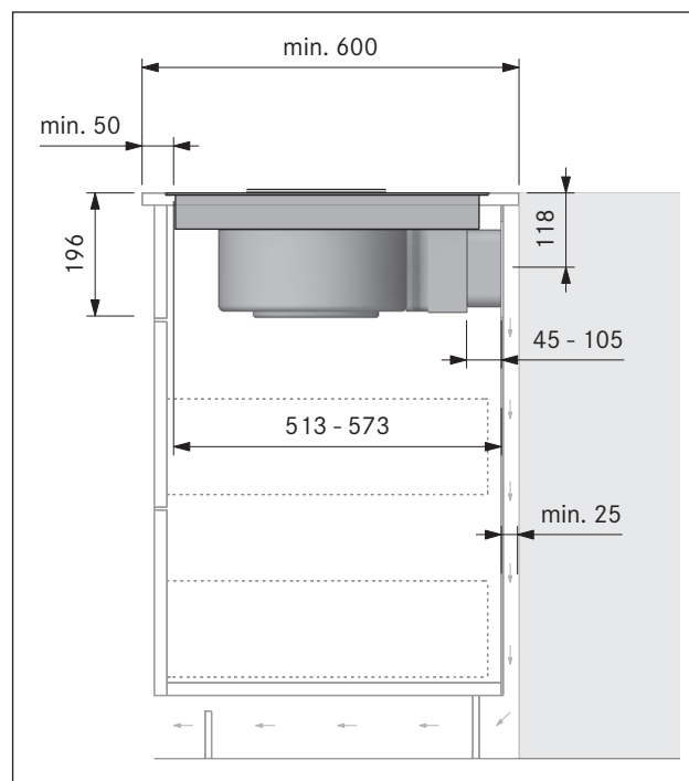
bild 6.9 Inbyggnadsmått vid luftcirkulation, bänkskivans djup 600mm
