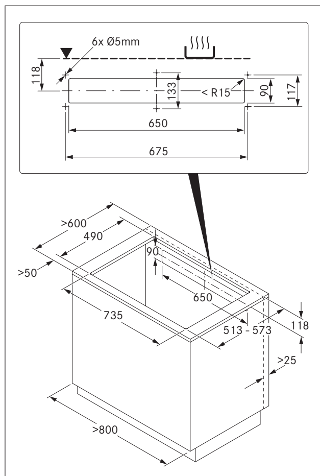
bild 6.8 Möbelmått vid luftcirkulation
