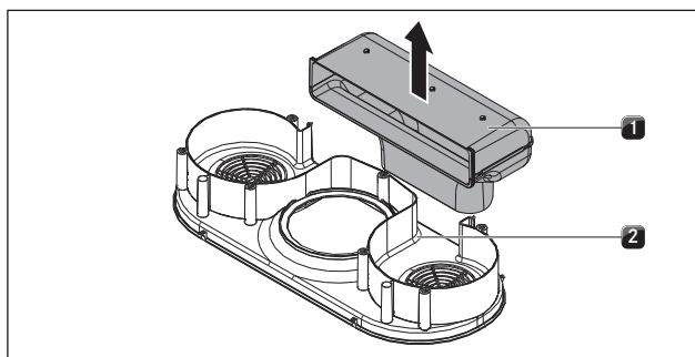
bild 6.27 Ta av utsugsbågen
