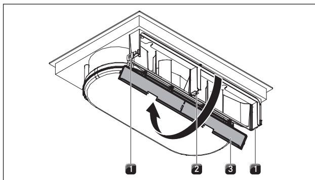
bild 6.13 Öppna kåpans lock
