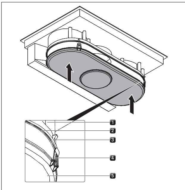
Fig. 8.4 Luk luftføringskabinettet
