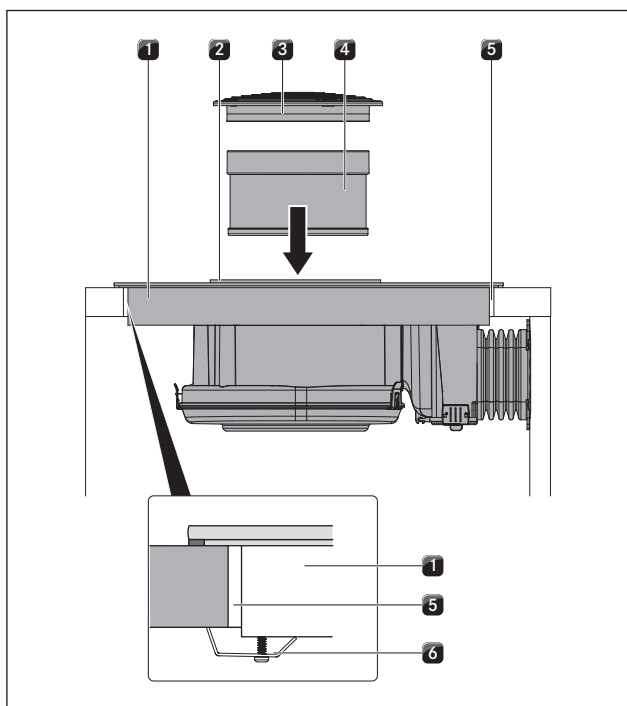
Fig. 6.16 Fastgør kogepladen i midten
