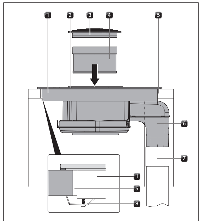
Fig. 6.34 Tilslutning af udsugningskanalen + Fastmontering
