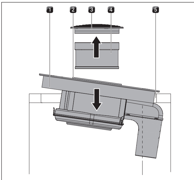
Fig. 6.32 Indsæt kogeplade
