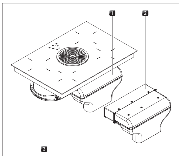
Obr. 5.3 Digestoř s odvodem vzduchu (BHA)
