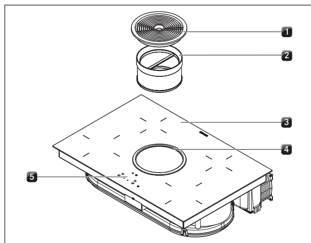
Obr. 5.1 Varná deska
