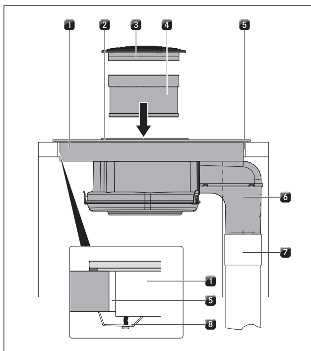
Obr. 6.34 Připojení odtahového kanálu + upevnění
