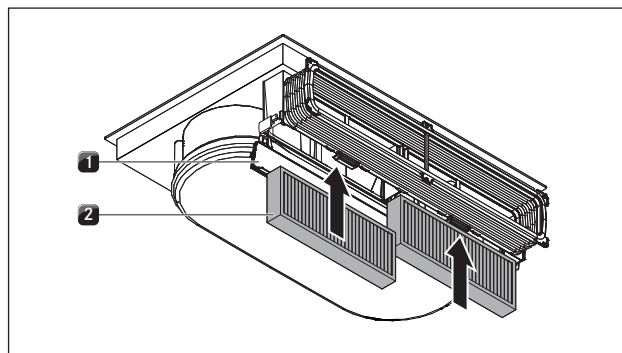
Kuva 6.16 Aktiivihiiisuodatintimen asettaminen paikalleen
