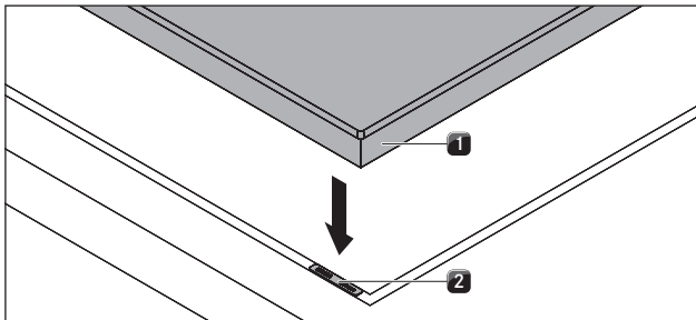
Kuva 6.18 Korkeussäätölevyt
