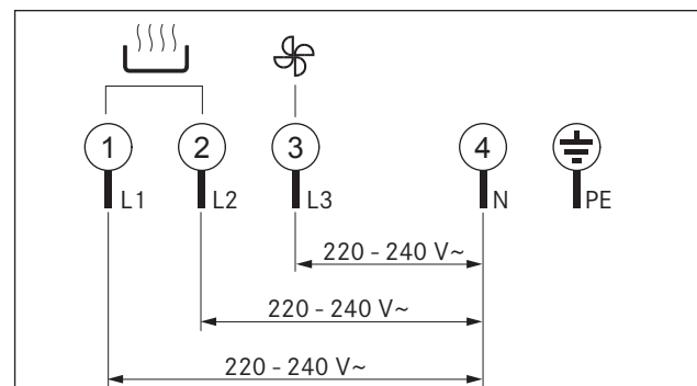
Kuva 6.36 Liitäntäkaavio - 3-vaiheiliitäntä
