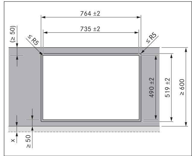
Kuva 6.3 Asennusaukkojen mitat upotusasennusta varten
