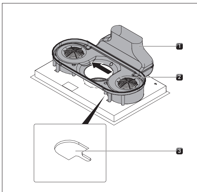
Kuva 6.26 Ilmanohjauksotelon siirtäminen
