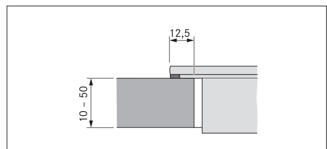
Kuva 6.6 Alustan mitat pinta-asennusta varten
