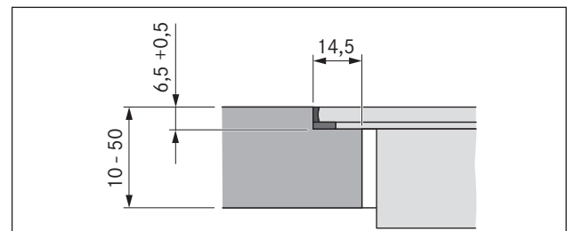
Kuva 6.4 Saumamitta upotusasennusta varten
