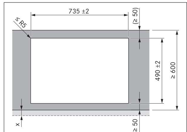
Kuva 6.5 Asennusaukkojen mitat pinta-asennusta varten
