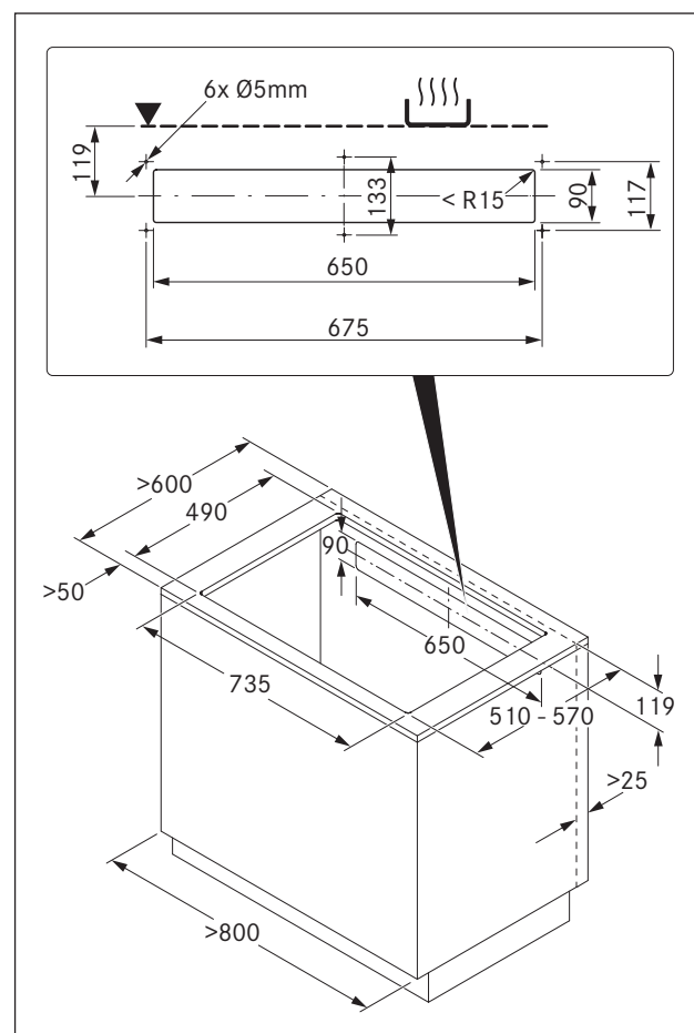
Kuva 6.9 Kalustemitat kiertoilmakäytössä
