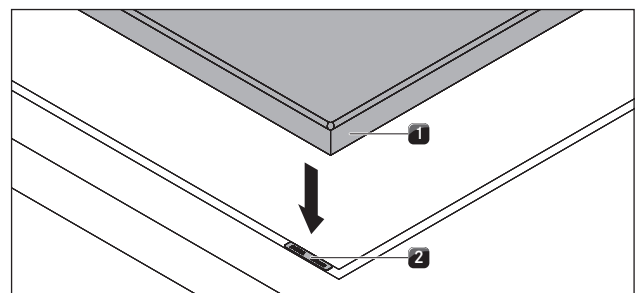
Kuva 6.17 Korkeussäätölevyt
