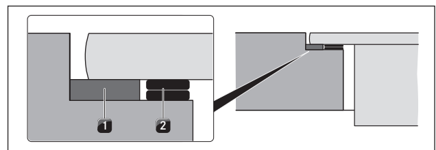
Fig. 6.38 Placas de compensación de altura
