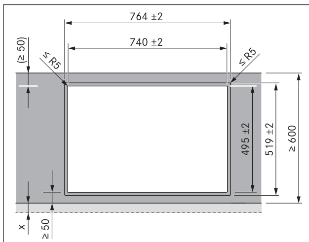
Fig. 6.11 Medidas del recorte para montaje enrasado
