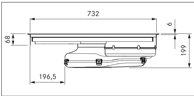
Fig. 3.8 PURA dimensiones, vista frontal
