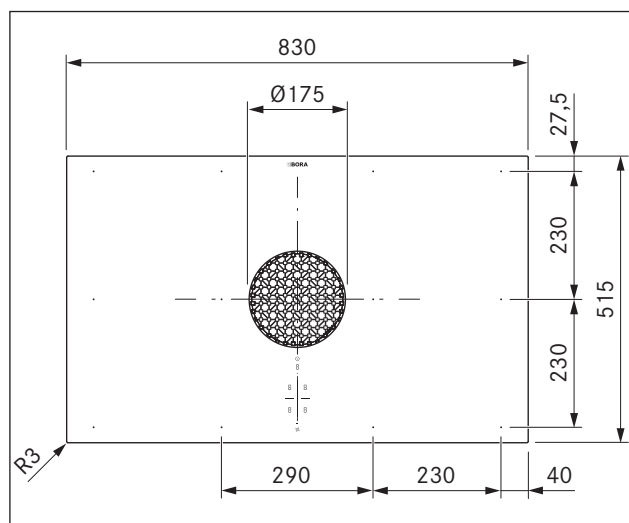
Fig. 3.4 PUXU dimensiones, vista superior
