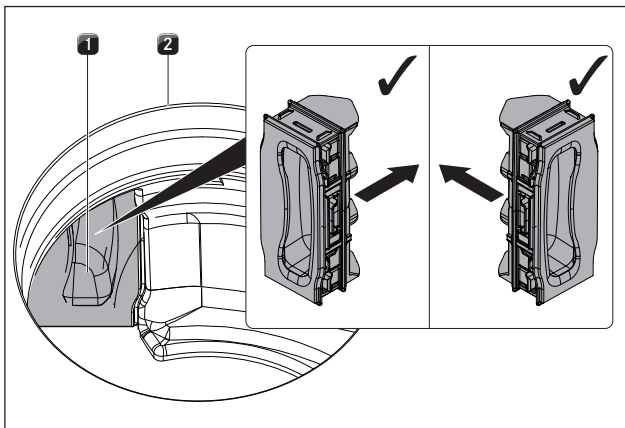
Fig. 6.45 Colocación de la trampilla para el cambio del filtro
