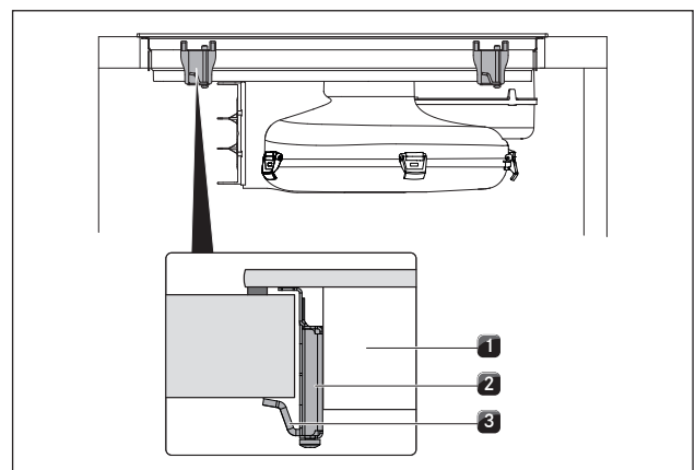
Fig. 6.39 Fijación de la placa de cocción
