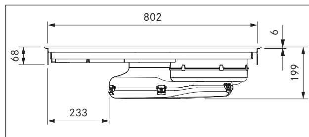
Fig. 3.2 PUXA dimensiones, vista frontal
