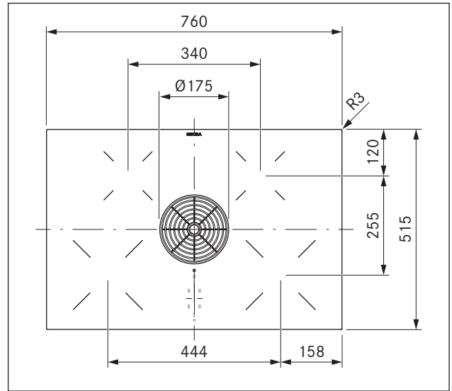
Fig. 3.10 PURU dimensiones, vista superior
