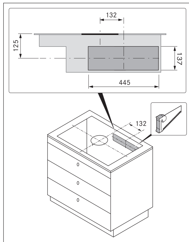
Fig. 6.28 Recorte de la abertura de flujo de retorno
