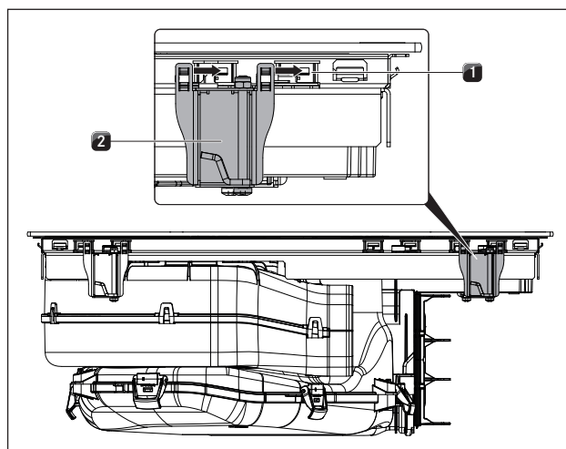
Fig. 6.33 Colocación de las abrazaderas de montaje
