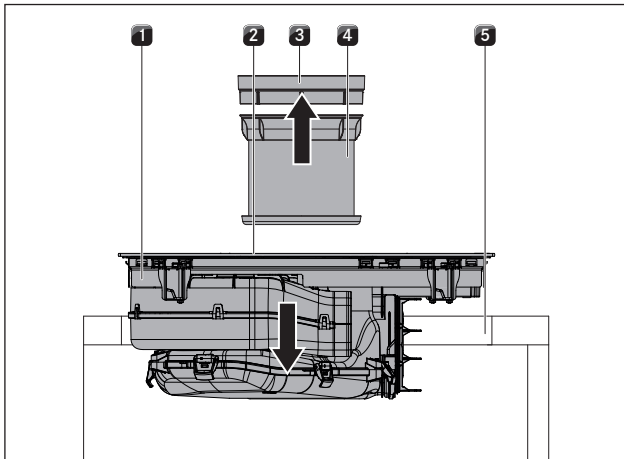
Fig. 6.19 Colocación de la placa de cocción
