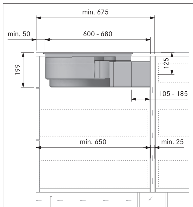
Fig. 6.34 Medidas de montaje para la variante de recirculación A, profundidad de la encimera 675 mm o más
