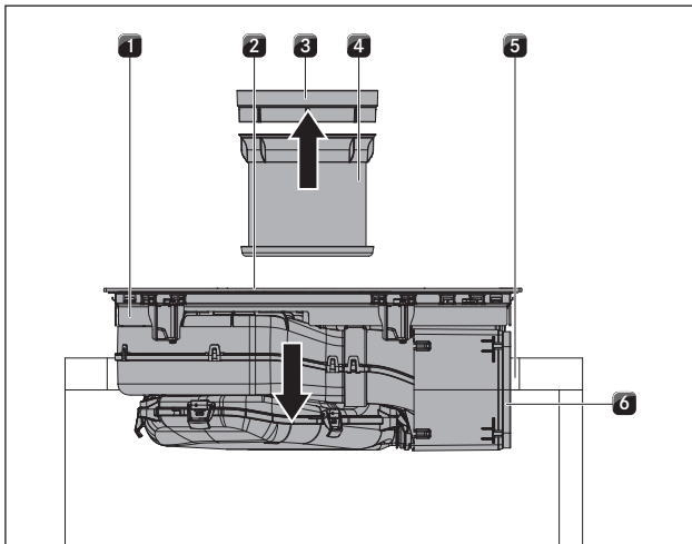
Fig. 6.36 Colocación de la placa de cocción en posición centrada
