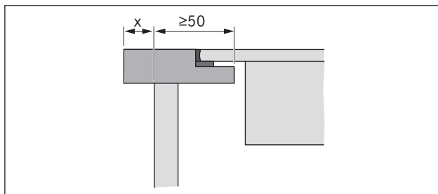
Fig. 6.6 Saliente de la encimera
