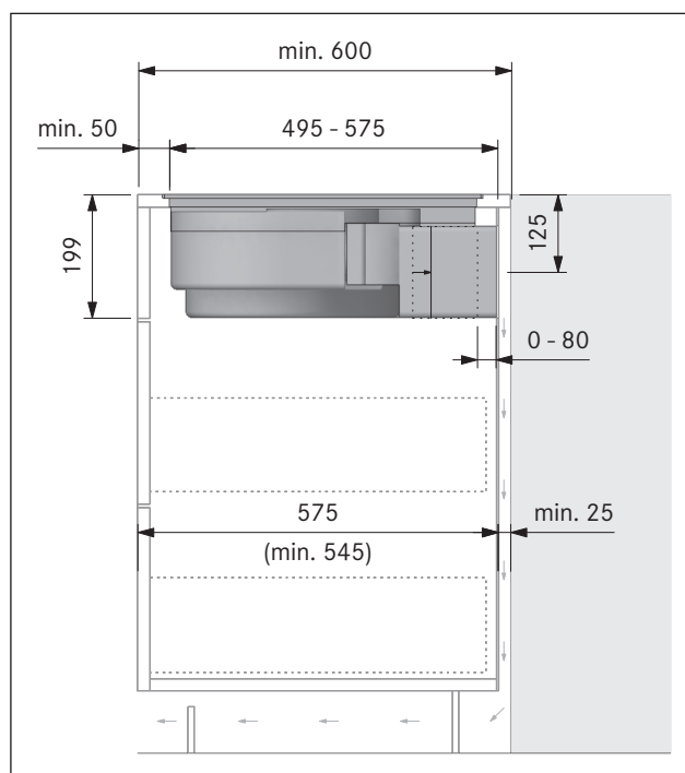
Fig. 6.27 Medidas de montaje con recirculación, variante de montaje A
