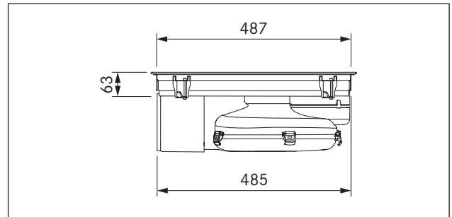
Fig. 3.12 PURU dimensiones, vista lateral
