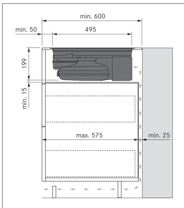
Fig. 6.30 Medidas de montaje para la variante de recirculación B, profundidad de la encimera 600 mm
