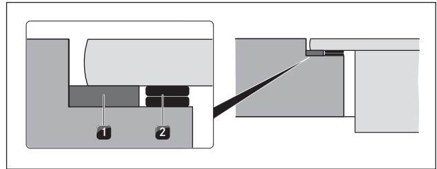
Fig. 6.21 Placas de compensación de altura
