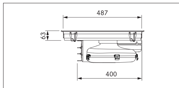
Fig. 3.3 PUXA dimensiones, vista lateral
