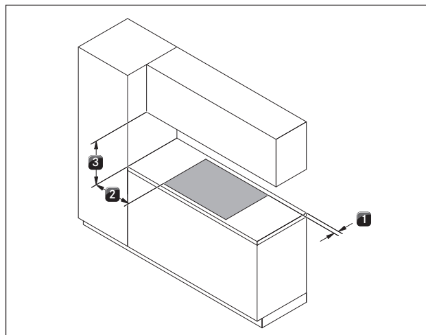
Fig. 6.3 Especificación de distancias de seguridad
