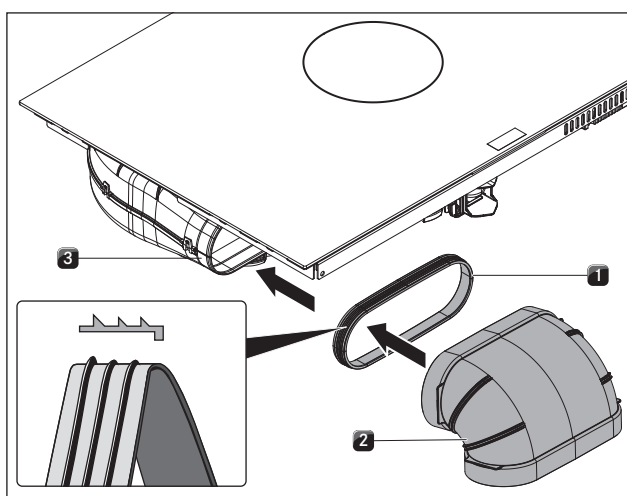
Fig. 6.23 Conexión al sistema de conductos
