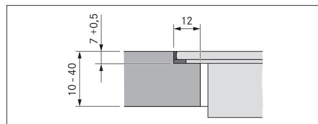
Fig. 6.8 Medida del pliegue para un montaje enrasado
