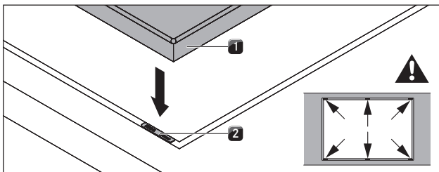
Fig. 6.20 Colocación de placas de compensación de altura
