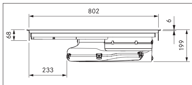
Fig. 3.5 PUXU dimensiones, vista frontal
