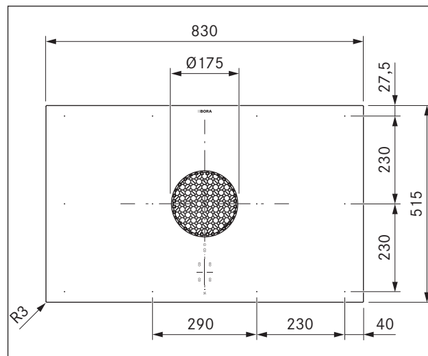
Fig. 3.1 PUXA dimensiones, vista superior
