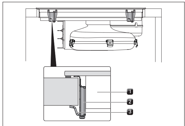
Fig. 6.22 Fijación de la placa de cocción en posición centrada
