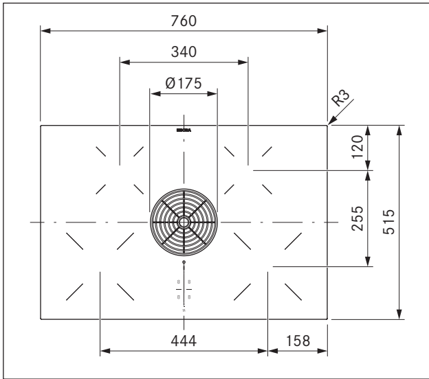
Fig. 3.7 PURA dimensiones, vista superior
