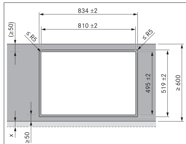
Fig. 6.7 Medidas del recorte para montaje enrasado
