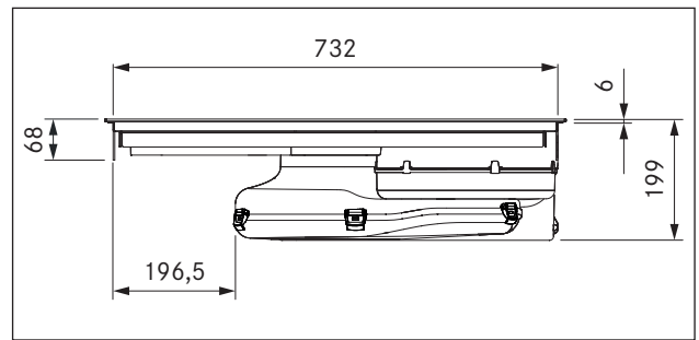
Fig. 3.11 PURU dimensiones, vista frontal
