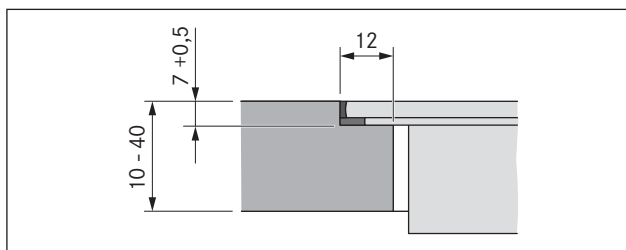
Fig. 6.12 Medida del pliegue para un montaje enrasado
