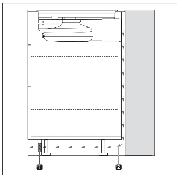
Fig. 6.24 Abertura de flujo de retorno en la zona del zócalo
