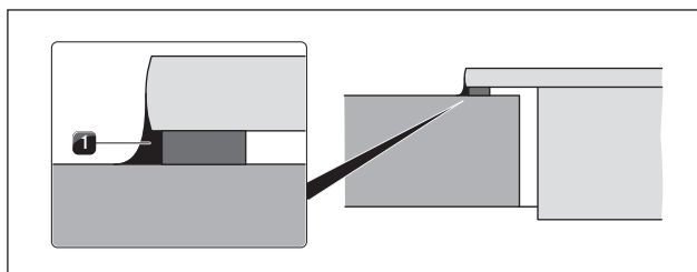
Fig. 6.55 Silicona de sellado para montaje superpuesto
