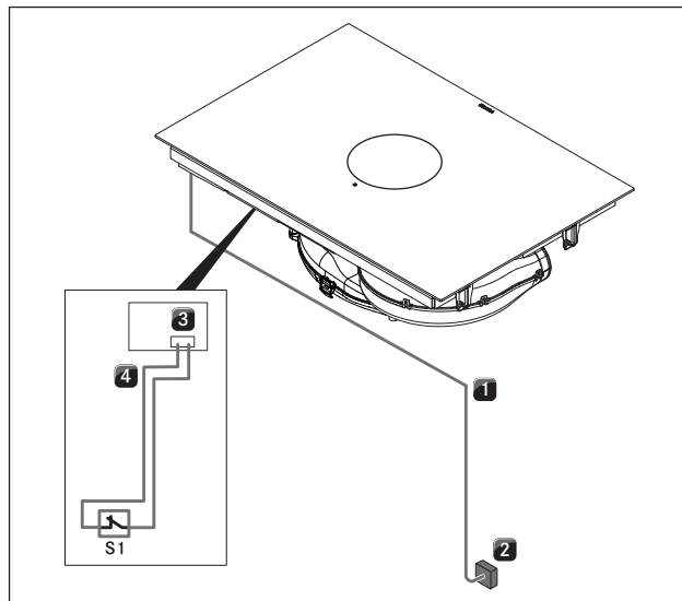
Fig. 6.46 Esquema de conexiones con el módulo opcional Home In
