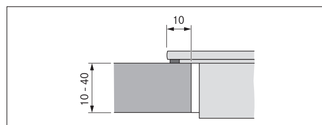
Fig. 6.10 Dimensiones para montaje superpuesto
