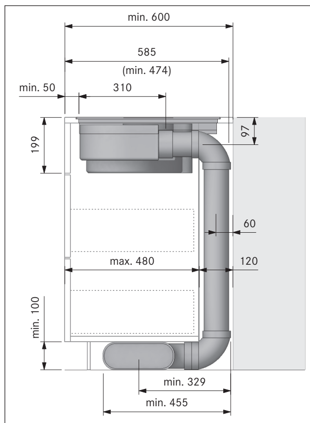
Fig. 6.15 Medidas de montaje para extracción al exterior, profundidad de la encimera 600 mm
