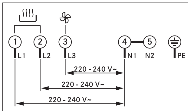
Fig. 6.47 Esquema de conexiones, conexión trifásica
