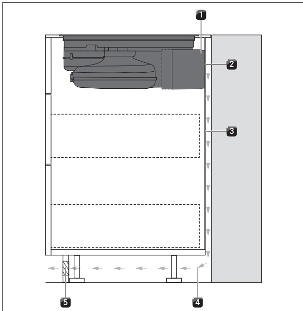
Fig. 6.25 Variante de montaje con panel trasero continuo
