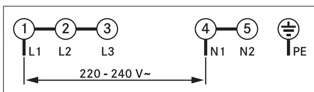
Fig. 6.49 Esquema de conexiones conexión monofásica
