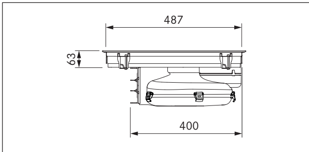
Fig. 3.9 PURA dimensiones, vista lateral
