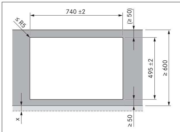
Fig. 6.13 Medidas del recorte para montaje superpuesto
