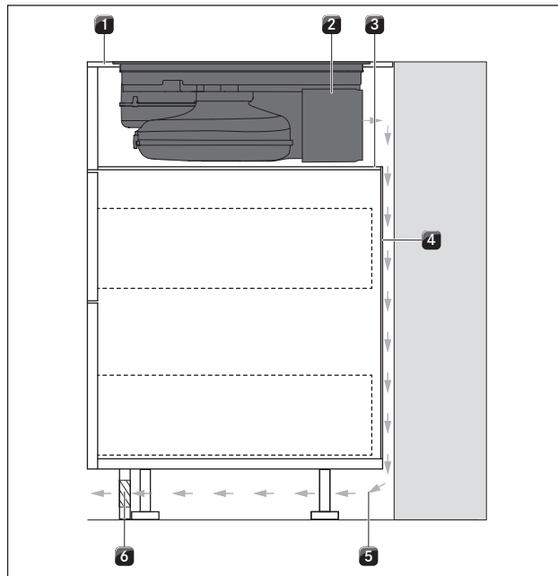
Fig. 6.26 Variante de montaje con base intermedia
