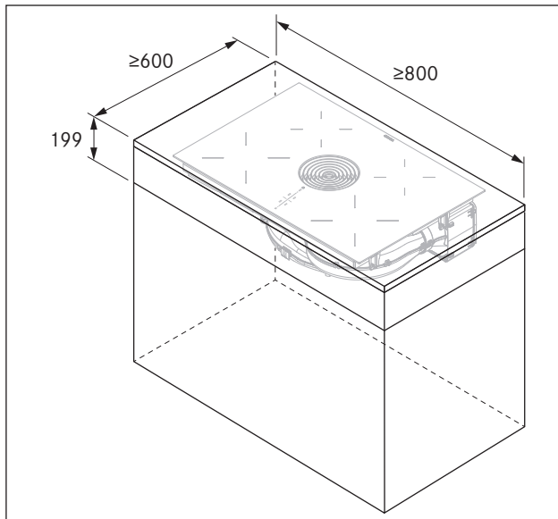
Fig. 6.5 Medidas mínimas de los muebles Pure
