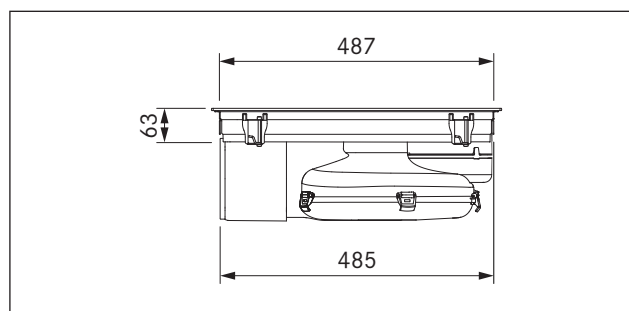
Fig. 3.6 PUXU dimensiones, vista lateral
