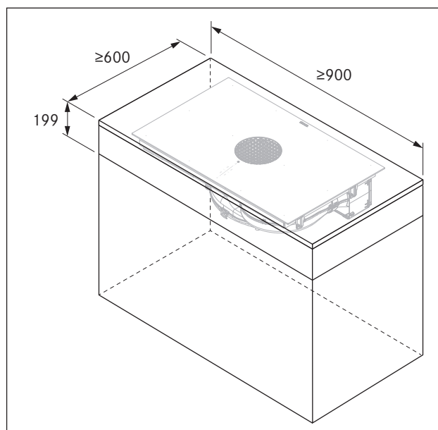
Fig. 6.4 Medidas mínimas de los muebles X Pure
