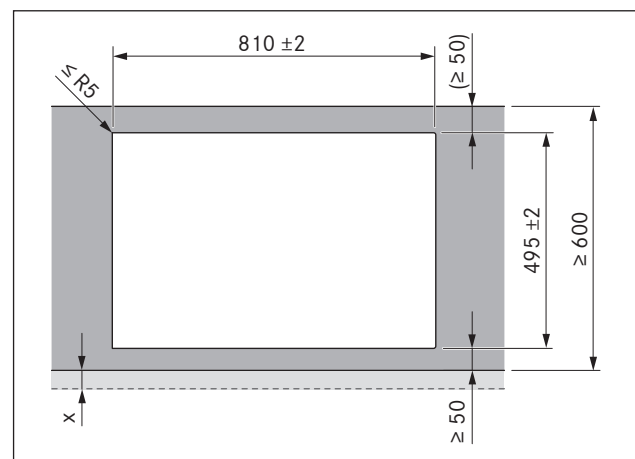
Fig. 6.9 Medidas del recorte para montaje superpuesto
