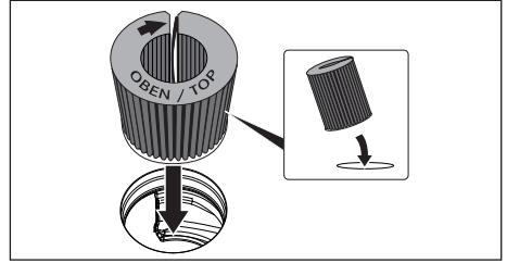
Kuva 10.42 Aktiivihiiisuodattimen asettaminen tuloaukkoon
