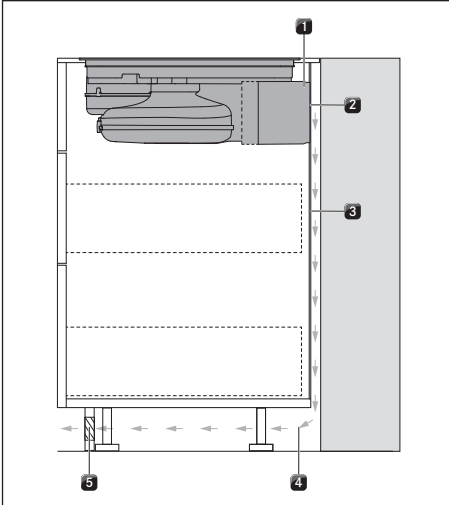
Kuva 10.24 Asennusvaihtoehto, jossa yhtenäinen takaseinä
