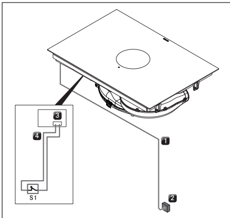
Kuva 10.45 Liitäntäkaavio, valinnainen home in -moduuli
