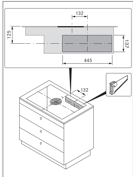
Kuva 10.27 Takaseinän aukkoa
