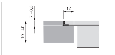
Kuva 10.11 Saumamitta uppoasennusta varten
