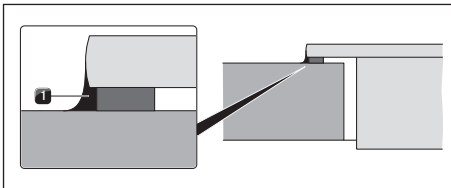
Kuva 10.54 Silikonitiivistysmassassa pinta-asennuksessa
