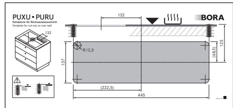
Kuva 10.28 Sapluna takaseinän aukkoa varten
