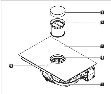
Kuva 5.1 Keittotaso
