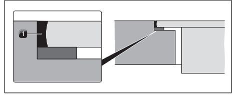
Kuva 10.55 Silikonitiivistysmassassa uppoasennuksessa
