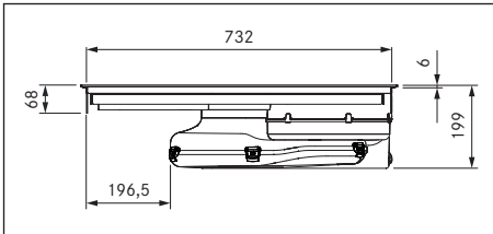
Kuva 3.5 Laitemitat PURU kuva edestä
