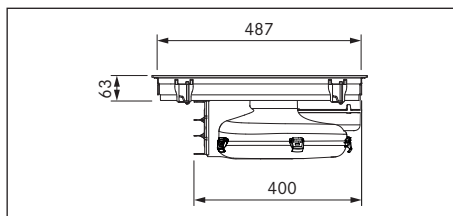
Kuva 3.3 Laitemitat PURA sivukuva
