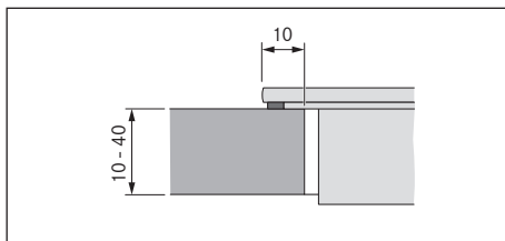
Kuva 10.9 Alustan mitat pinta-asennusta varten
