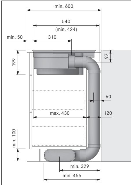
Kuva 10.14 Asennusmitat poistoilmakäytössä, työtason syvyys 600 mm
