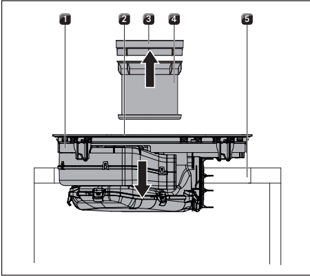
Kuva 10.18 Keittotason asettaminen paikalleen
