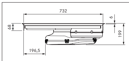
Kuva 3.2 Laitemitat PURA kuva edestä
