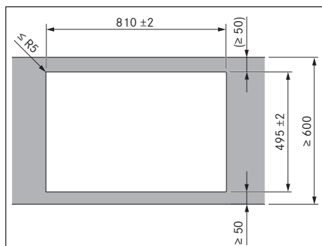
Kuva 10.8 Asennusaukkojen mitat pinta-asennusta varten
