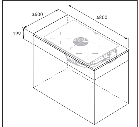
Kuva 10.5 Kalusteen vähimmäismitat Pure
