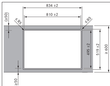
Kuva 10.6 Asennusaukkojen mitat uppoasennusta varten
