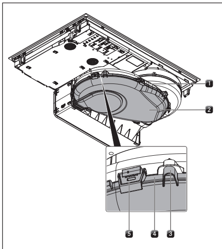
Kuva 8.4 Ilmanohjaukotelon
