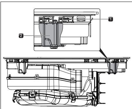
Kuva 10.32 Kiinnittimien kiinnittäminen
