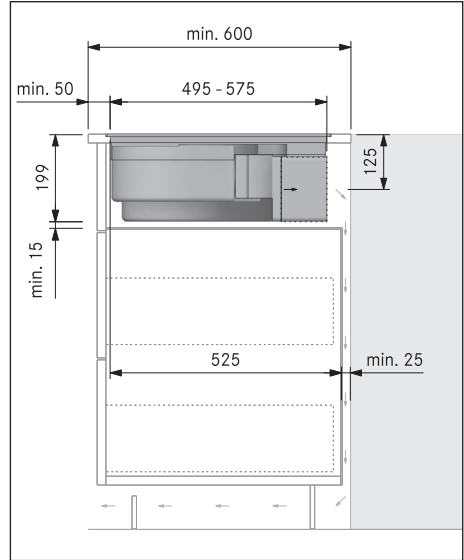
Kuva 10.29 Asennusmitat kiertoilma-asennuksessa B, työtason syvyys 600 mm
