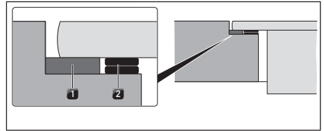
Kuva 10.20 Korkeussäätölevyt
