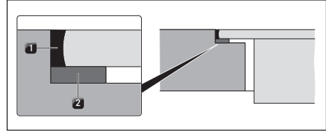
Kuva 10.16 Tiivistenauha uppoasennuksessa
