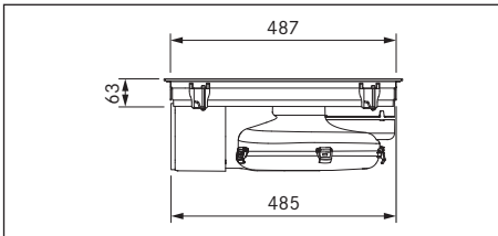
Kuva 3.6 Laitemitat PURU sivukuva
