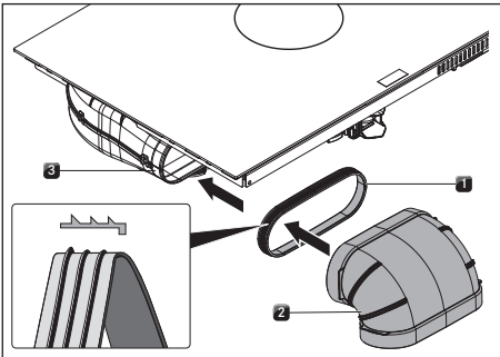
Kuva 10.22 Liittäminen kanavajärjestelmään
