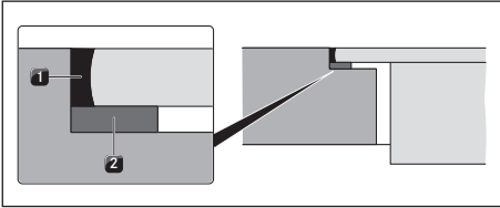
Kuva 10.31 Tiivistenauha uppoasennuksessa
