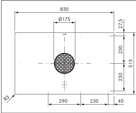
Kuva 3.1 Laitemitat PUXA kuva ylhäältä
