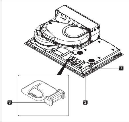
Kuva 10.49 Keittotason sähköliitännät
