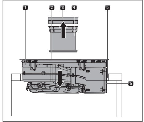
Kuva 10.35 Keittotason asettaminen keskelle
