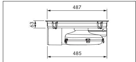
Kuva 3.6 Laitemitat PUXU sivukuva
