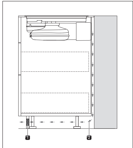
Kuva 10.23 Paluuilman aukko sokkelialueella
