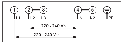
Kuva 10.47 Liitäntäkaavio - 2-vaiheiliitäntä
