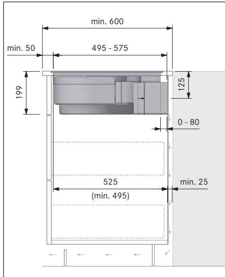
Kuva 10.26 Asennusmitat kiertoilmakäytössä, asennusvaihtoehto A
