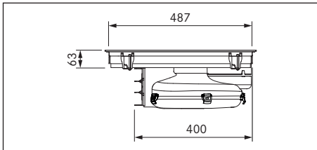
Kuva 3.3 Laitemitat PUXA sivukuva
