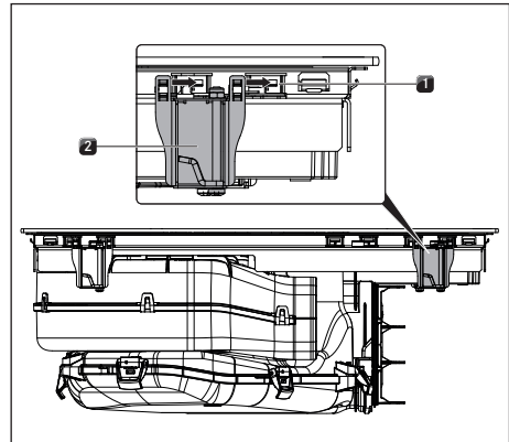
Kuva 10.17 Kiinnittimien kiinnittäminen
