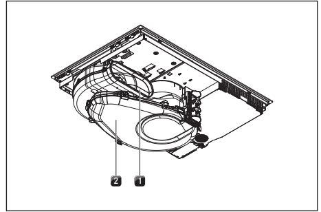
Kuva 5.2 Näkymä takaa PUXA, PURA
