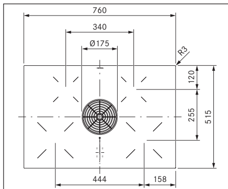
Kuva 3.1 Laitemitat PURA kuva ylhäältä
