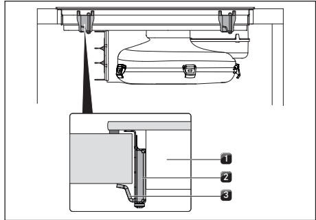
Kuva 10.38 Keittotason kiinnittäminen
