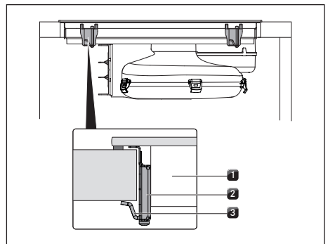
Kuva 10.21 Keittotason kiinnittäminen keskelle
