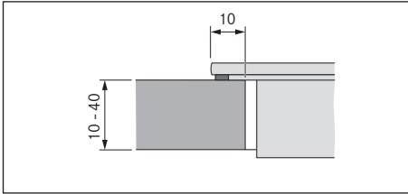
Kuva 10.13 Alustan mitat pinta-asennusta varten
