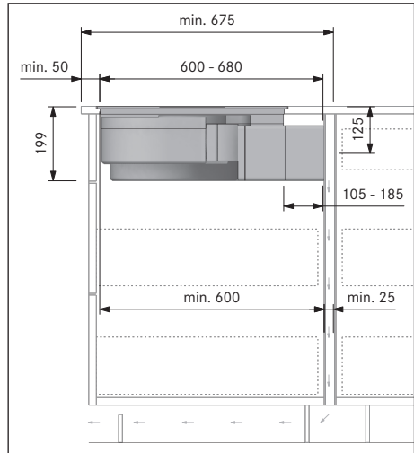
Kuva 10.33 Asennusmitat kiertoilma-asennuksessa A, työtason syvyys yli 675 mm
