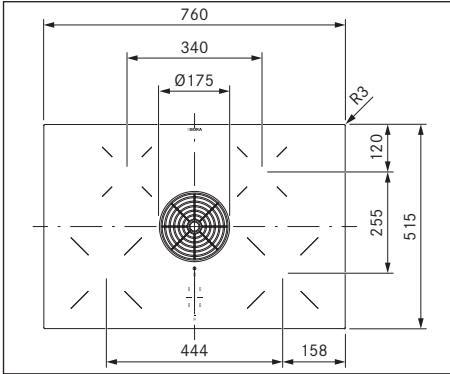
Kuva 3.4 Laitemitat PURU kuva ylhäältä
