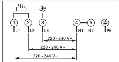
Kuva 10.46 Liitäntäkaavio - 3-vaiheiliitäntä
