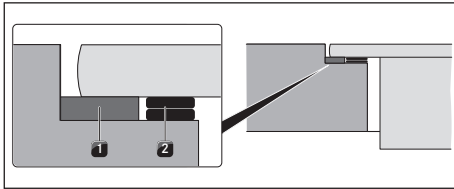
Kuva 10.37 Korkeussäätölevyt
