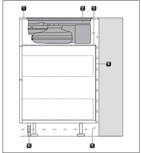
Kuva 10.25 Asennusvaihtoehto, jossa välipohja
