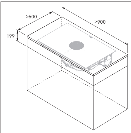
Kuva 10.4 Kalusteen vähimmäismitat X Pure
