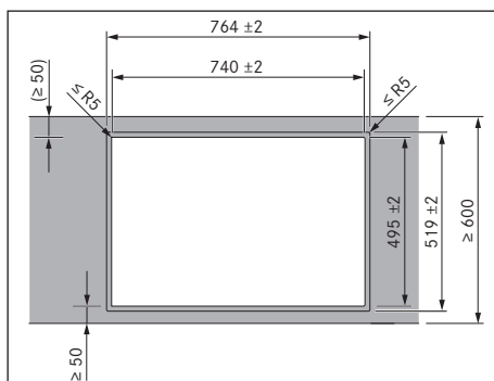
Kuva 10.10 Asennusaukkojen mitat uppoasennusta varten
