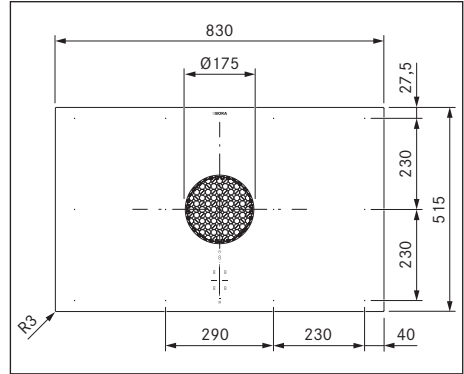
Kuva 3.4 Laitemitat PUXU kuva ylhäältä
