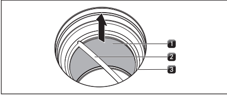
Kuva 8.3 Ruostumattomasta teräksestä valmistetun rasvasuodattimen irrottaminen
