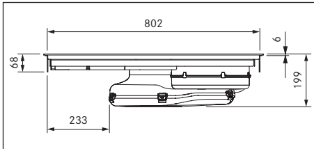
Kuva 3.2 Laitemitat PUXA kuva edestä
