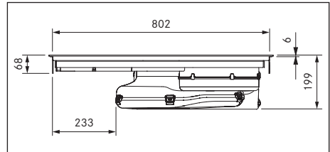
Kuva 3.5 Laitemitat PUXU kuva edestä
