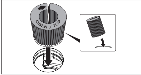
Kuva 8.9 Aktiivihiilisuodattimen asettaminen tuloaukkoon
