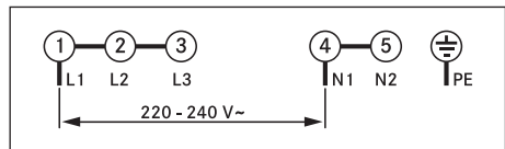
Kuva 10.48 Liitäntäkaavio - 1-vaiheiliitäntä
