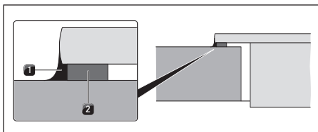
Kuva 10.15 Tiivistenauha pinta-asennuksessa
