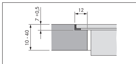
Kuva 10.7 Saumamitta uppoasennusta varten
