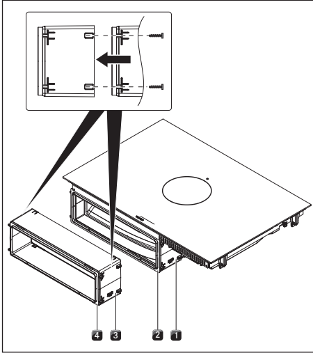
Kuva 10.34 Ulosvedettävän osan pidennys
