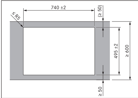
Kuva 10.12 Asennusaukkojen mitat pinta-asennusta varten
