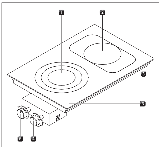
Kuva 4.2 Keittotaso PC3B
