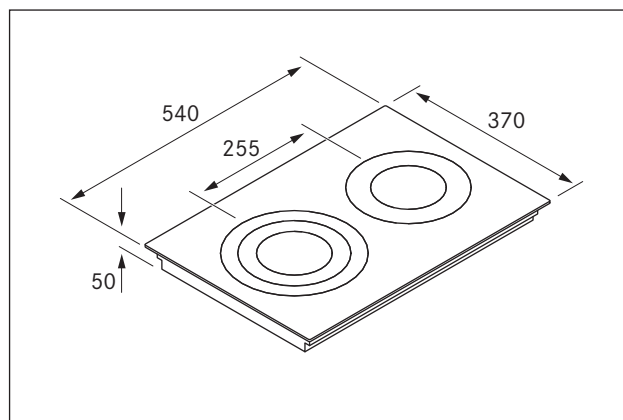
Kuva 3.1 Laitemitat PC32
