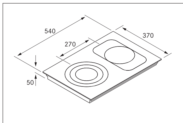
Kuva 3.2 Laitemitat PC3B
