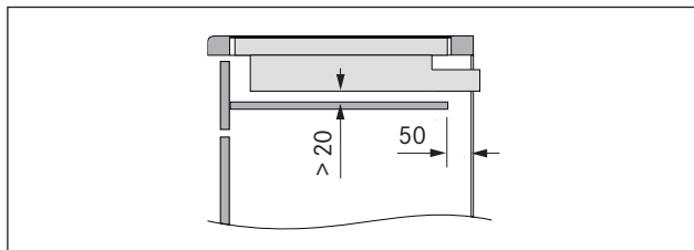
Ilustracja 5.2 Widok z boku: osłona kabla i wentylacja
