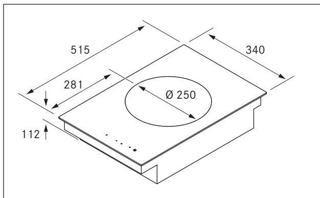
Ilustracja 3.1 Wymiar urządzenia
