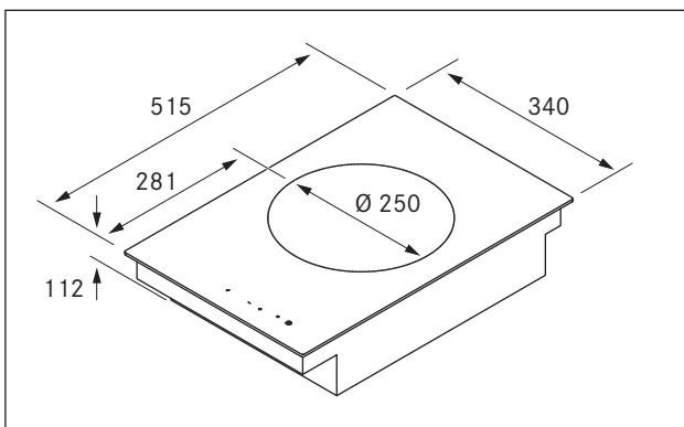
Afb. 3.1 Toestelafmetingen
