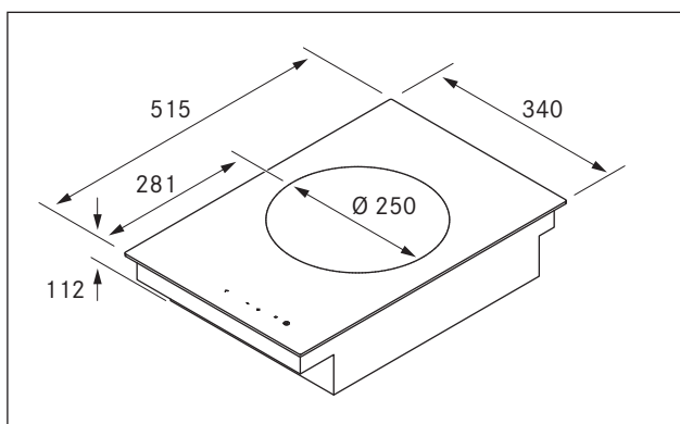
Fig. 3.1 Dimensioni dell'apparecchio
