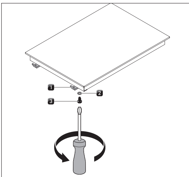
Obr. 5.11 Upevňovací svorky
