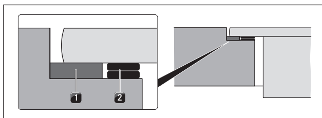
Fig. 6.30 Placas de compensación de altura
