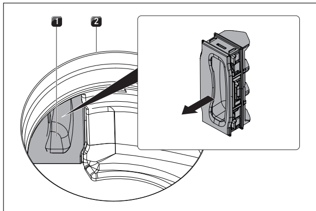
Fig. 8.4 Retirar la trampa para cambio del filtro
