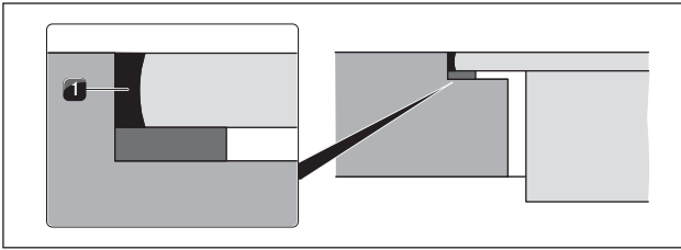
Fig. 6.41 Silicona de sellado para montaje enrasado
