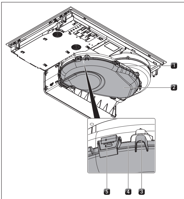
Fig. 8.3 Carcasa de conducción del aire
