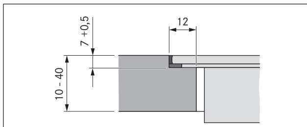
Fig. 6.5 Medida del pliegue para un montaje enrasado
