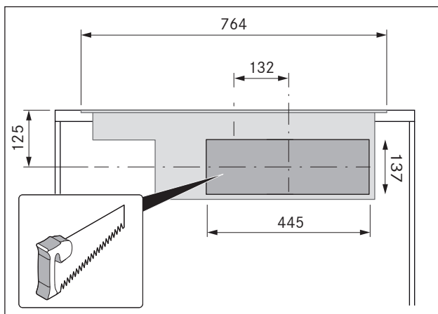
Fig. 6.11 Recorte para la abertura de flujo de retorno
