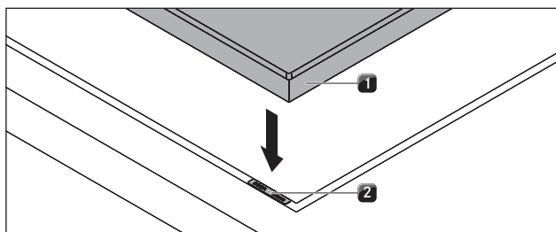
Fig. 6.29 Colocación de placas de compensación de altura
