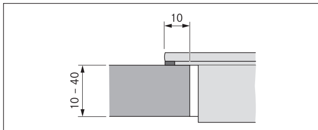
Fig. 6.7 Dimensiones para montaje superpuesto
