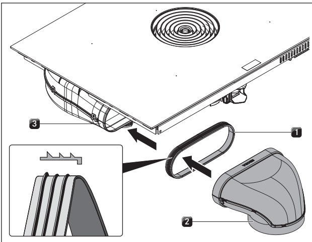
Fig. 6.32 Conexión al sistema de conductos
