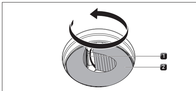
Fig. 8.5 Extracción del filtro de carbón activo de su carcasa
