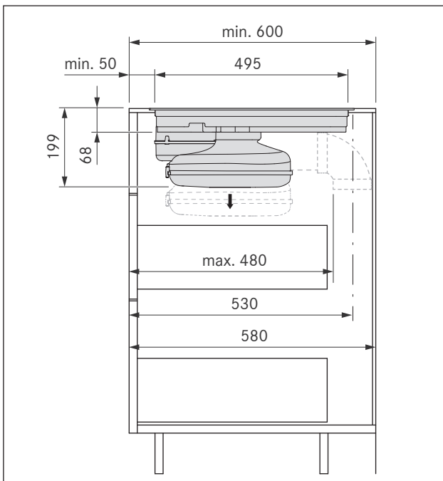
Fig. 6.26 Medidas de montaje para extracción al exterior, profundidad de la encimera 600 mm
