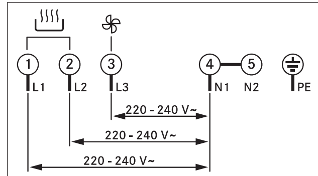
Fig. 6.33 Esquema de conexiones, conexión trifásica
