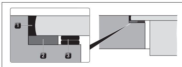
Fig. 6.9 Cinta selladora para montaje enrasado
