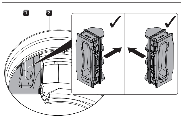
Fig. 6.23 Colocación de la trampilla para el cambio del filtro
