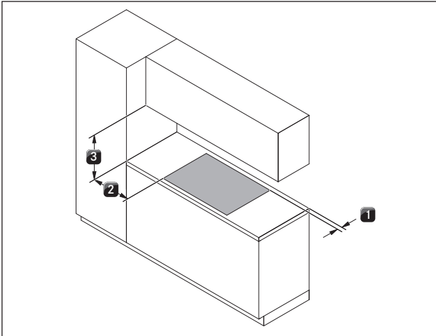
Fig. 6.1 Distancias mínimas recomendadas
