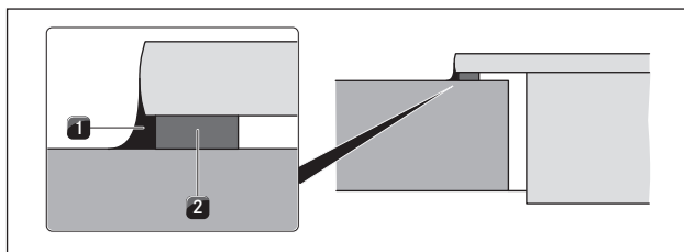
Fig. 6.8 Cinta selladora para montaje superpuesto
