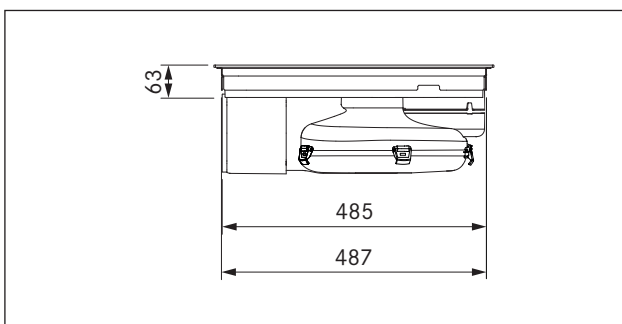
Fig. 3.6 PURU dimensiones, vista lateral
