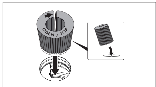
Fig. 6.21 Colocación del filtro de carbón activo en la abertura del extractor
