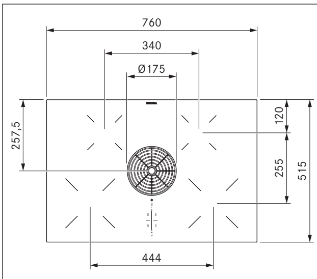
Fig. 3.4 PURU dimensiones, vista superior
