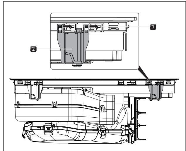
Fig. 6.27 Colocación de la placa de cocción
