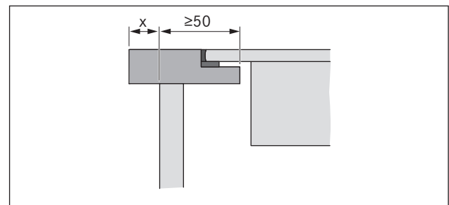
Fig. 6.3 Saliente de la encimera
