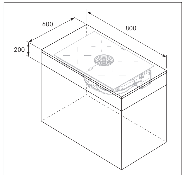
Fig. 6.2 Medidas mínimas de los muebles
