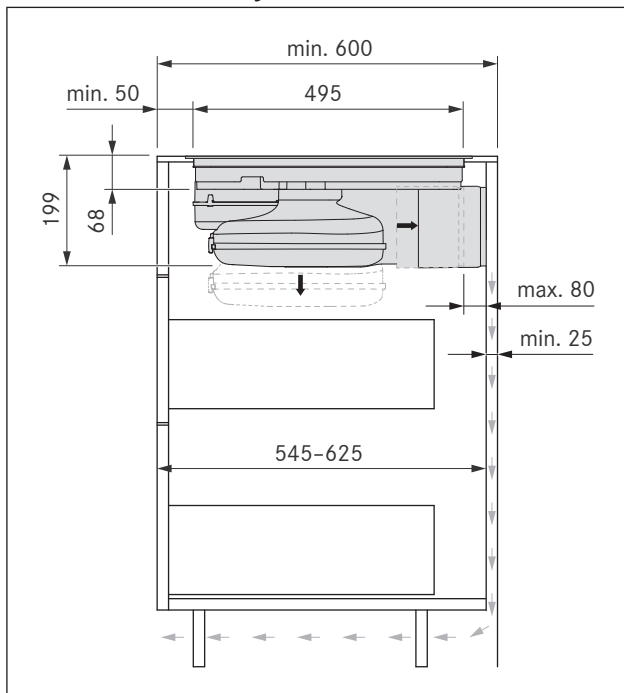
Fig. 6.10 Medidas de montaje para recirculación, profundidad de la encimera 600 mm
