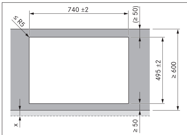
Fig. 6.6 Medidas del recorte para montaje superpuesto
