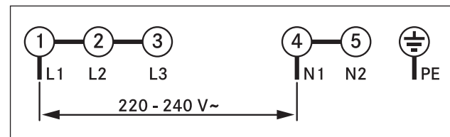
Fig. 6.35 Esquema de conexiones, conexión monofásica
