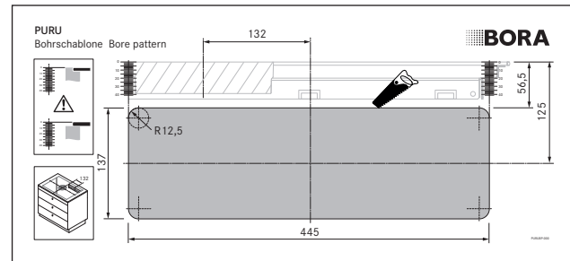
Fig. 6.12 Plantilla para el recorte del panel trasero
