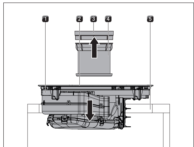
Fig. 6.28 Colocación de la placa de cocción
