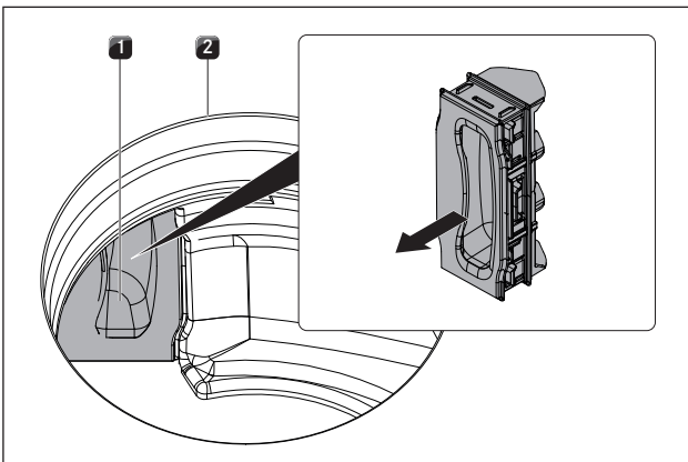
Fig. 6.19 Retirar la trampa para cambio del filtro
