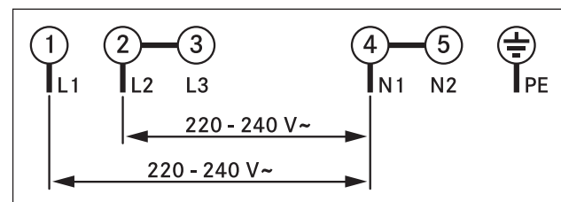
Fig. 6.34 Esquema de conexiones, conexión bifásica
