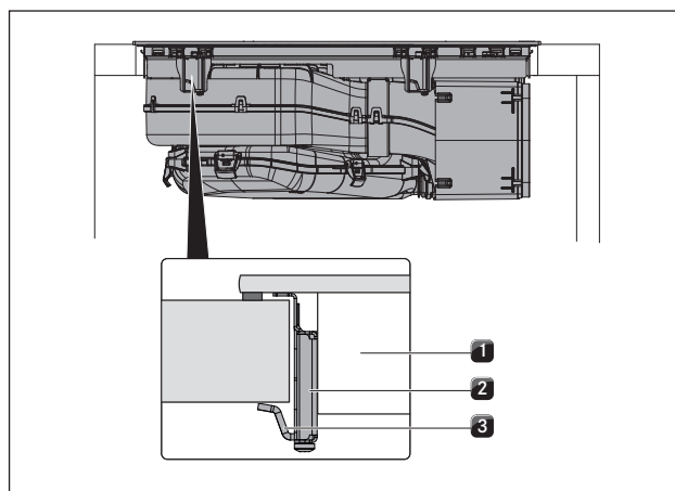
Fig. 6.31 Fijación de la placa de cocción en posición centrada
