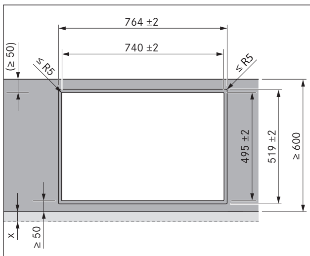
Fig. 6.4 Medidas del recorte para montaje enrasado
