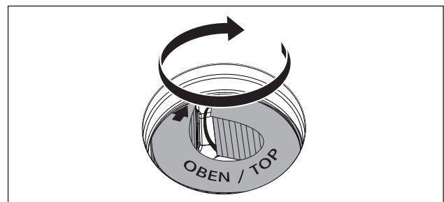
Fig. 6.22 Colocación del filtro de carbón activo en la posición final
