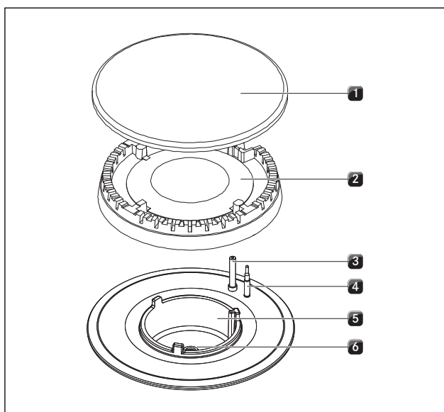
bild 5.26 Gasbrännare uppbyggnad
