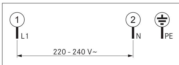
Sl. 5.25 1-fazna priključna shema
