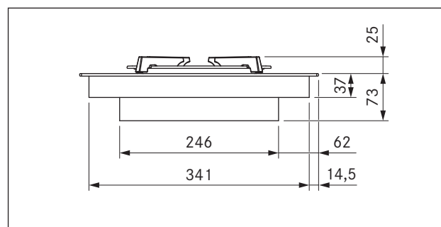
Fig. 3.3 PKG11 dimensões do aparelho vista frontal
