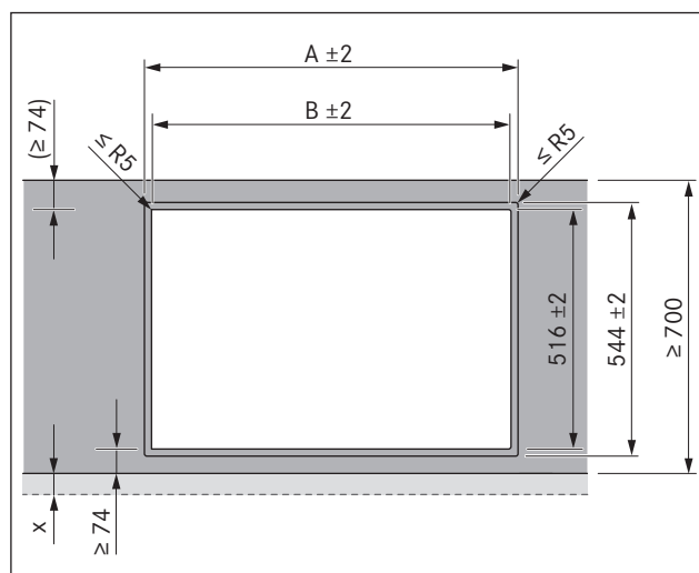
Fig. 5.6 Medidas de recorte para montagem à face
