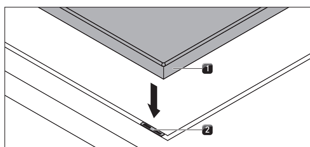
Fig. 5.16 Placa de cozinhar e placas de compensação de altura
