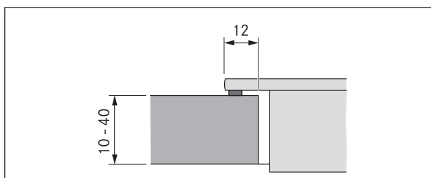
Fig. 5.9 Corte para montagem por sobreposição
