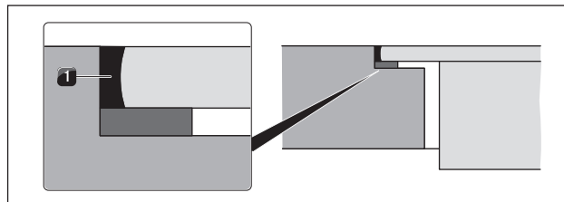
Fig. 5.18 Massa vedante de silicone na montagem à face
