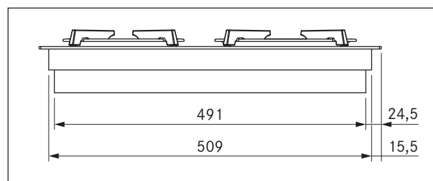
Fig. 3.4 PKG11 dimensões do aparelho vista lateral
