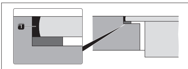
איור 5.29 חומר איטום מסיליקון בהתקנה מובנית
