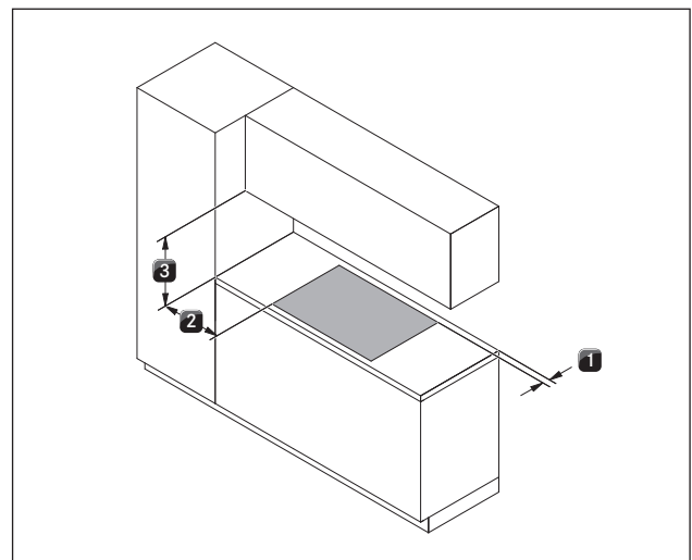
איור 5.1 מרווחים מינימליים
