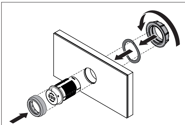
איור 5.13 התקנת כפתור הבקרה
