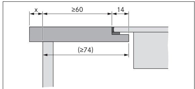
איור 5.5 בליטת משטח העבודה
