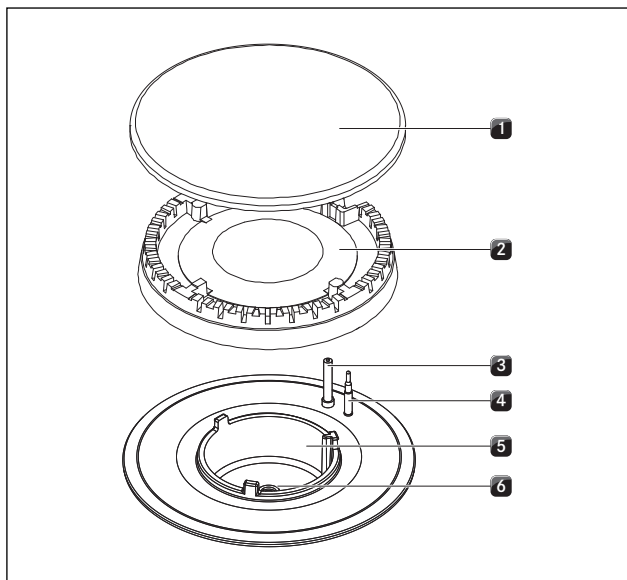
איור 7.2 פירוק מבער הגז
