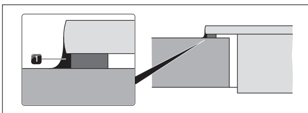
איור 5.30 חומר איטום מסיליקון בהתקנה עילית
