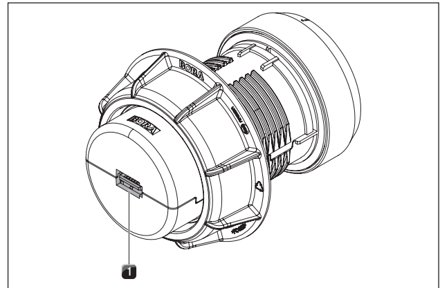
איור 5.20 חיבור כפתור הבקרה, צד אחורי
