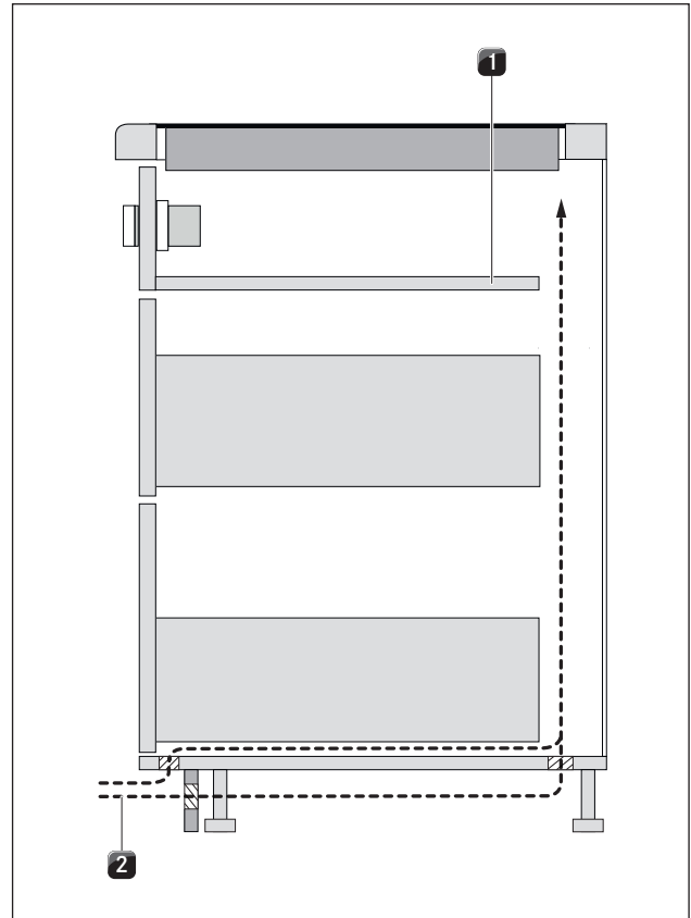
איור 5.3 הזרמת אוויר באזור הבסיס
