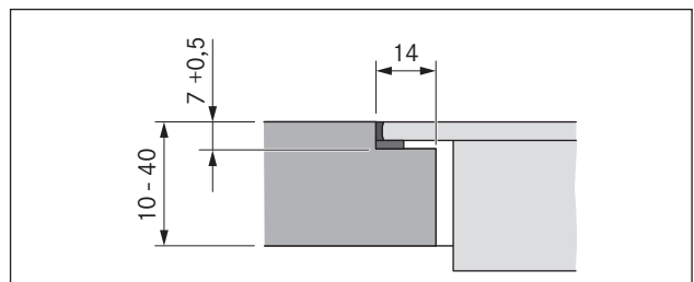
איור 5.7 מידות מופחתות עבור התקנה מובנית
