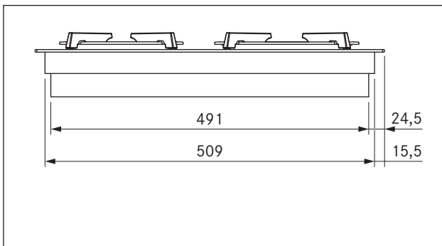
איור 3.4 מידות PKG11, מבט מהצד
