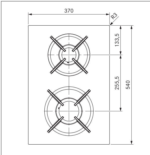
איור 3.2 מידות PKG11, מבט מלמעלה
