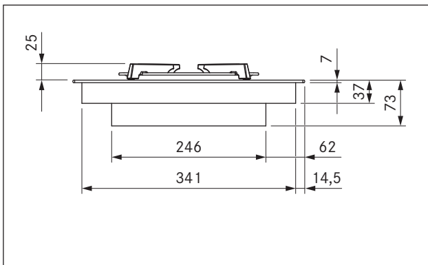
איור 3.3 מידות PKG11, מבט מלפנים
