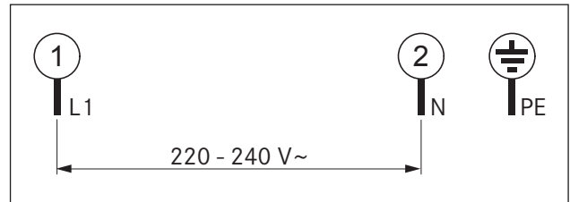
איור 5.25 תרשים חיבור חד-פאזי
