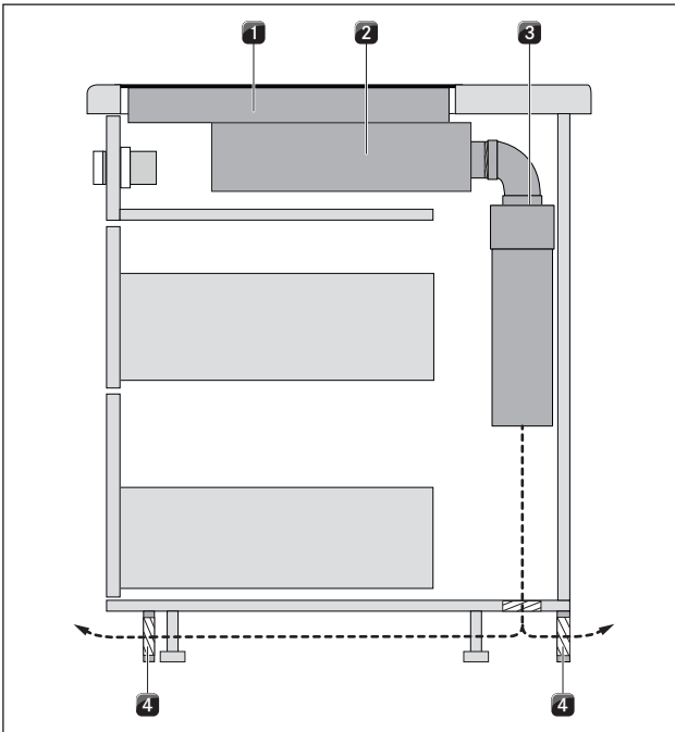
איור 5.4 דוגמה לתכנון הזרימה חוזרת של האוויר המסוחרר (אי מטבח + PKAS + PKG11-100 + יחידת ניקוי אוויר)
