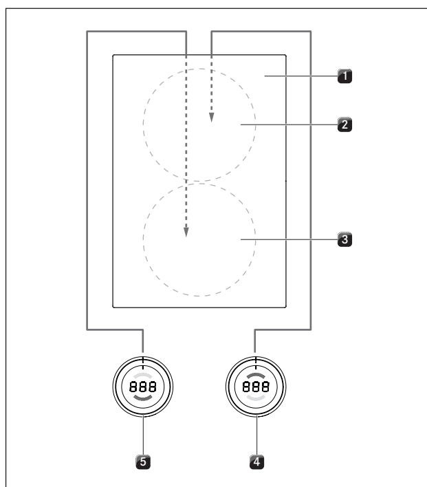
Fig. 5.23 Raccordement des zones de cuisson en montage à 180°
