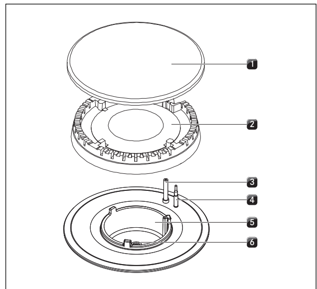
Fig. 7.2 Composition du brûleur à gaz
