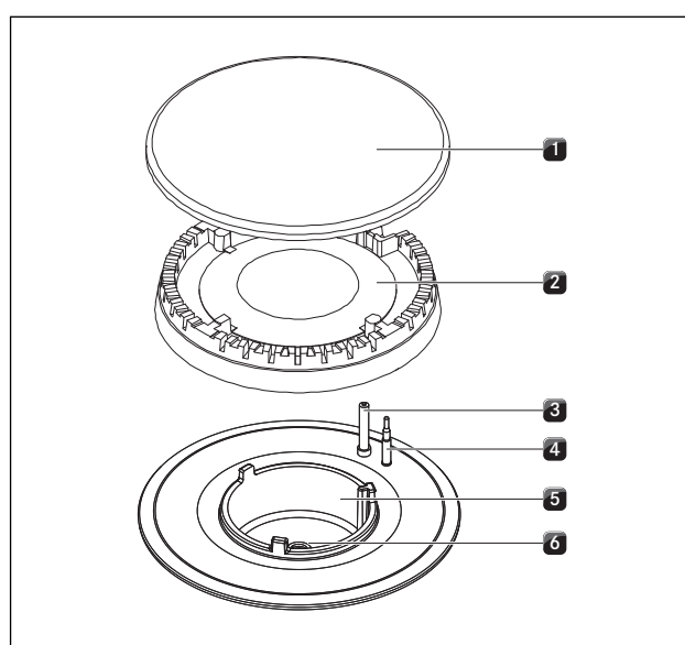
Fig. 5.25 Composition du brûleur à gaz
