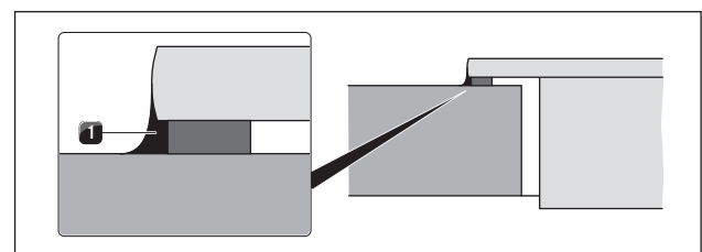
Kuva 5.30 Silikonitiivistysmassa pinta-asennuksessa
