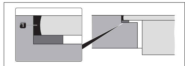
Kuva 5.29 Silikonitiivistysmassa uppoasennuksessa
