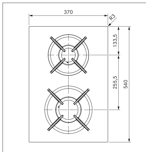
Kuva 3.2 Laitemitat PKG11, kuva ylhäältä
