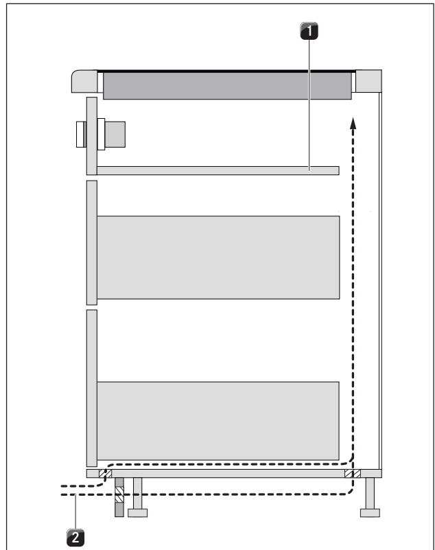
Kuva 5.3 Ilmansyöttö sokkelialueelta
