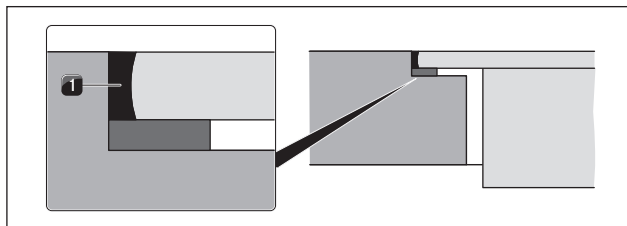
Obr. 5.29 Silikonová těsnicí hmota při plošně zarovnané montáži
