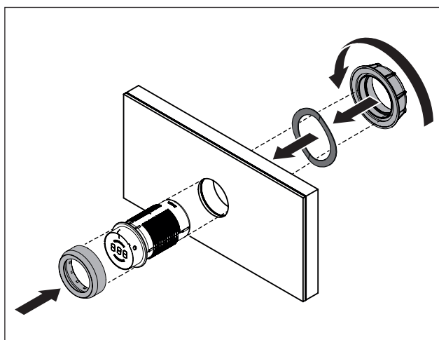
Obr. 5.13 Montáž ovládacích koleček
