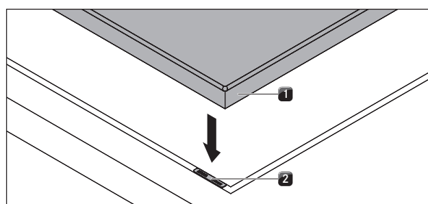
Obr. 5.18 Varná deska a podložky k nastavení výšky
