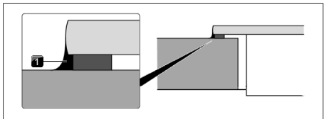
Fig. 11.35 Silicona de sellado para montaje superpuesto
