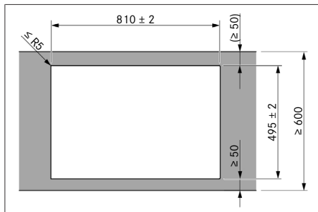
Fig. 11.7 Medidas del recorte para montaje superpuesto
