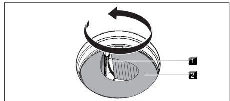
Fig. 9.5 Desenrosacar el filtro de carbón activo para extraerlo de su carcasa
