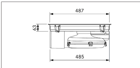
Fig. 3.6 PUXU2/R dimensiones, vista lateral
