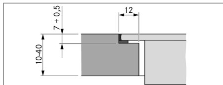
Fig. 11.6 Medida del rebaje para un montaje enrasado
