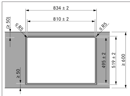
Fig. 11.5 Medidas del recorte para montaje enrasado
