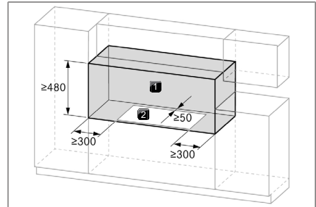
Fig. 11.3 Espacio libre requerido
