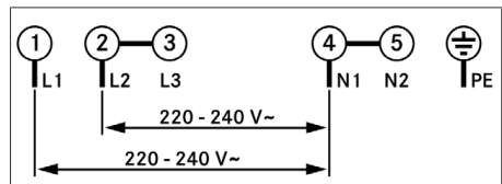
Fig. 11.29 Esquema de conexiones, conexión bifásica
