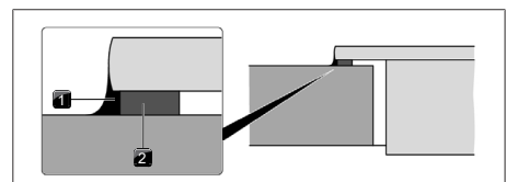
Fig. 11.17 Cinta selladora para montaje superpuesto
