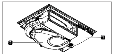
Fig. 4.3 Vista posterior variante de recirculación
