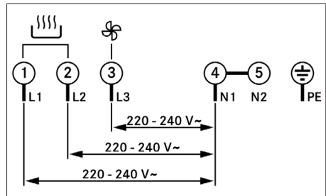
Fig. 11.27 Esquema de conexiones, conexión trifásica
