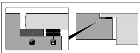
Fig. 11.22 Placas de compensación de altura
