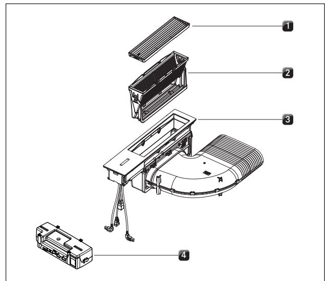
Afb. 4.5 BORA Classic kookveldafzuiging CKA2
