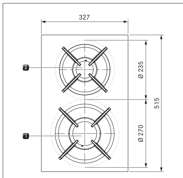
Afb. 4.17 Afmetingen kookzones
