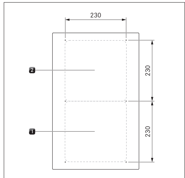
Afb. 4.7 Afmetingen kookzones
