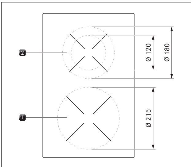
Afb. 4.13 Afmetingen kookzones
