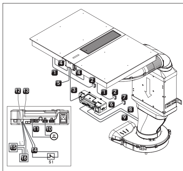
Afb. 4.37 Aansluitschema kookveldafzuiging CKA2
