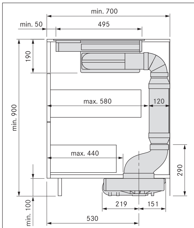
Afb. 4.14 Inbouwmaten toestel met vlakke geluidsdemper USDF bij corpusdiepte 700 mm
