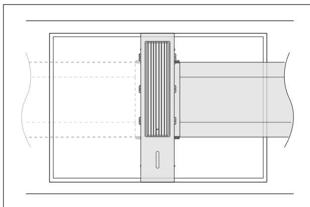
Afb. 4.17 Luchtgeleiding zijwaarts recht (rechts of links)
