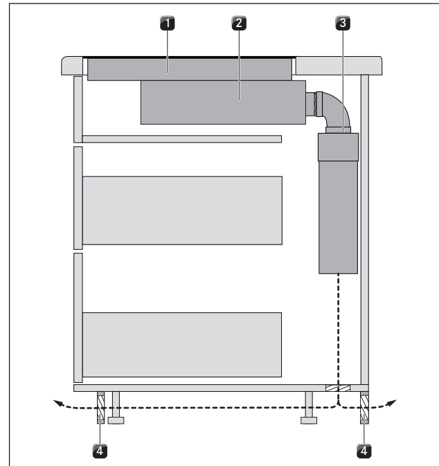
Afb. 4.20 Ontwerpvoorbeeld terugloop bij recirculatie (keukeneiland + kookveld + CKA2 + luchtreinigingsunit)
