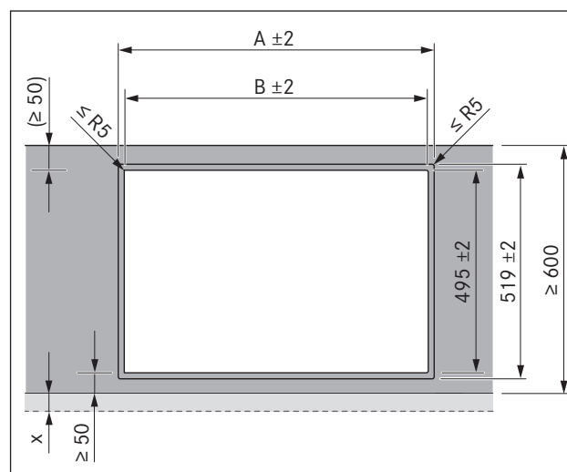
Afb. 4.7 Maten van de uitsparingen voor vlainbouw
