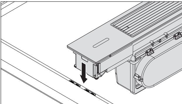
Afb. 4.22 Vulplaatjes bij vlakbouw
