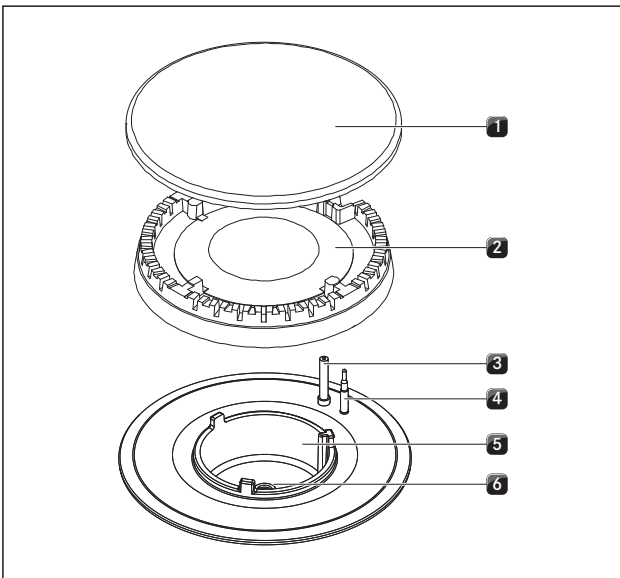
Afb. 4.44 Opbouw gasbrander
