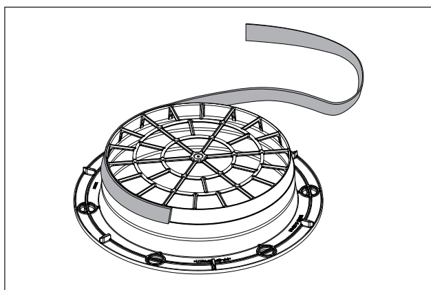
Afb. 4.24 Positie van de afdichtingsband voor montage met ronde buis
