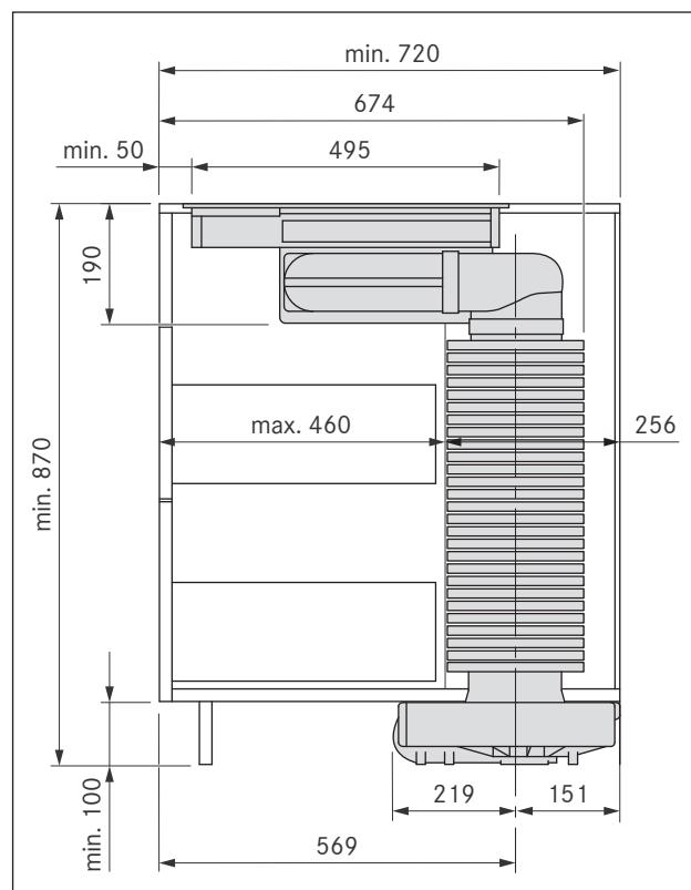
Afb. 4.15 Inbouwmaten toestel met ronde geluidsdemper USDR50
