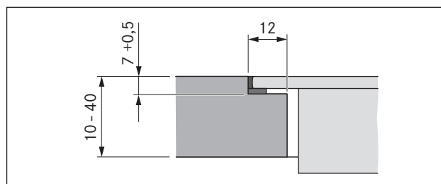
Afb. 4.8 Voegmaat voor vlainbouw
