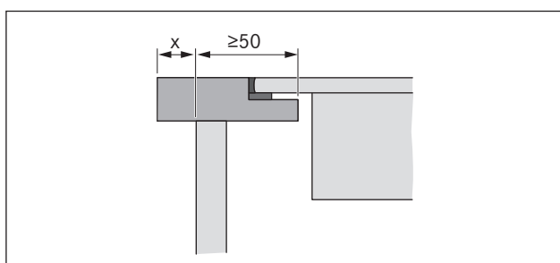
Afb. 4.6 Uitstekend deel van het werkblad
