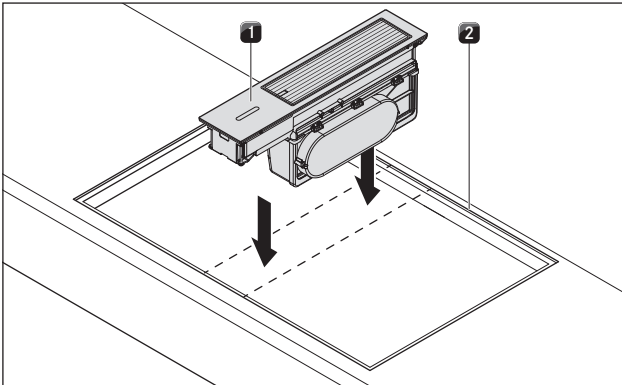
Afb. 4.21 Kookveldafzuiging in werkbladuitsparing plaatsen
