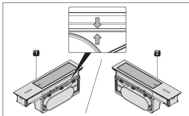
Afb. 4.18 Geassembleerde kookveldafzuiging CKA2
