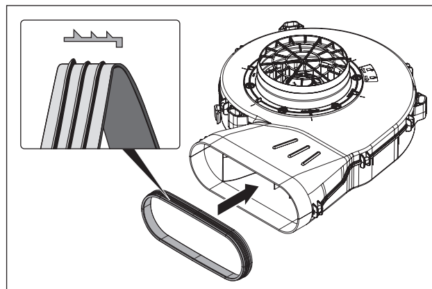
Afb. 4.25 Afdichting aanbrengen aan het uitloopsteunpunt van de plintmotor
