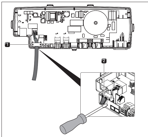
Afb. 4.36 Contact Home Out met trekontlasting
