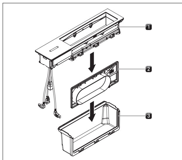
Afb. 4.19 Assemblage van de afzonderlijke componenten bij kookveldafzuiging CKA2
