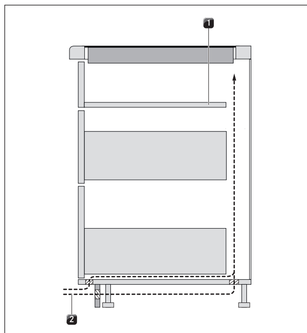
Afb. 4.5 Luchttoevoer in plintgedeelte
