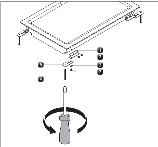
Afb. 4.32 Bevestigen van het Tepan kookveld
