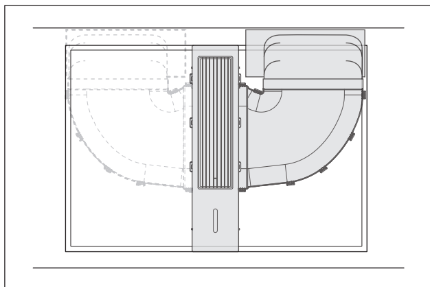
Afb. 4.16 Luchtgeleiding naar achteren (rechts of links)
