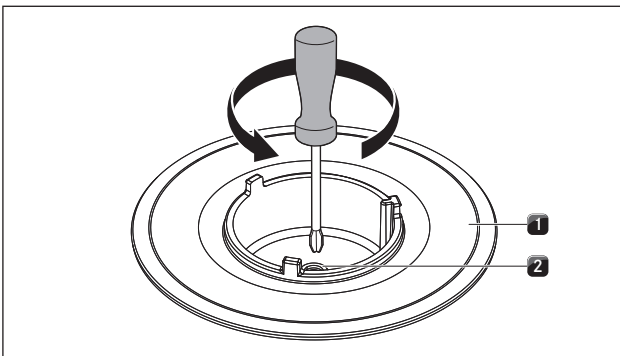
Afb. 4.45 Kookplaatbrander met gassproeier
