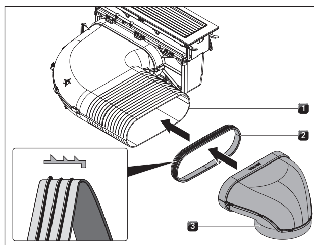
Afb. 4.26 Aansluiting op het kanaalsysteem
