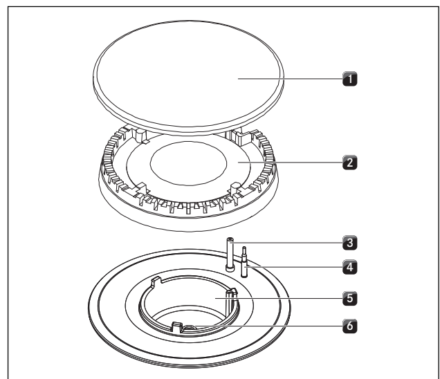
Abb. 9.5 Gas-Brenner Aufbau
