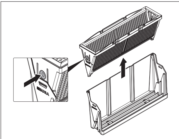
Abb. 9.3 Fettfilter entnehmen
