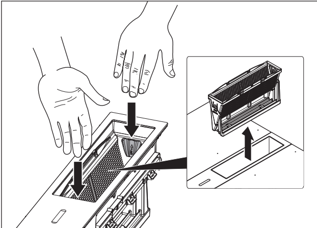
Abb. 9.2 Fettfiltereinheit entnehmen
