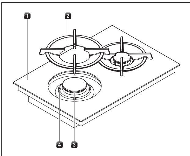
Abb. 9.4 Gas-Brenner Aufbau
