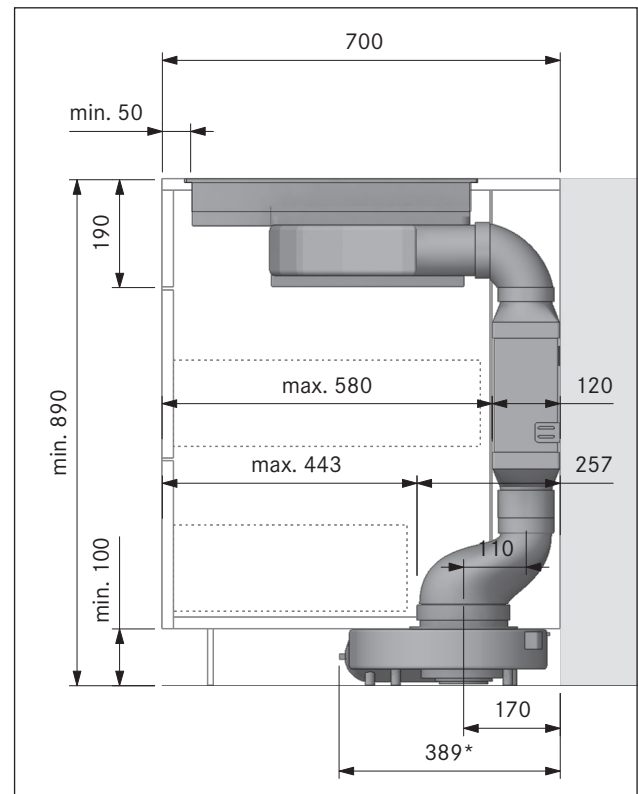
Fig. 4.14 Dimensions de montage de l'appareil avec silencieux plat USDF et raccord EFV
