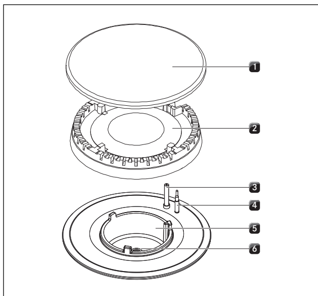
Fig. 4.41 Composition du brûleur à gaz
