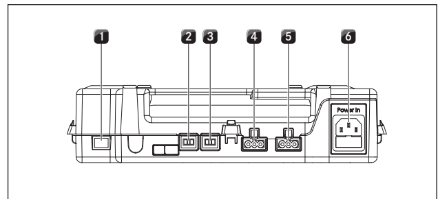
Fig. 4.38 Connecteurs de l'unité de régulation
