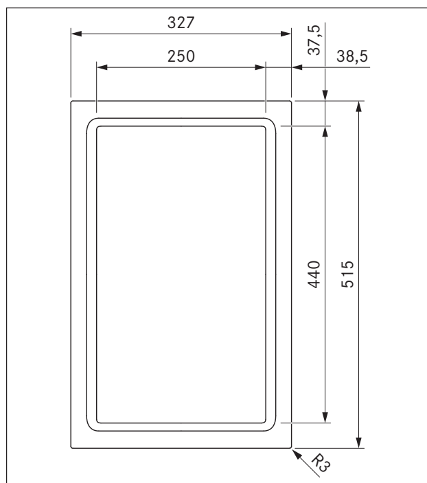
Fig. 3.23 Dimensions CKT - Vue de dessus
