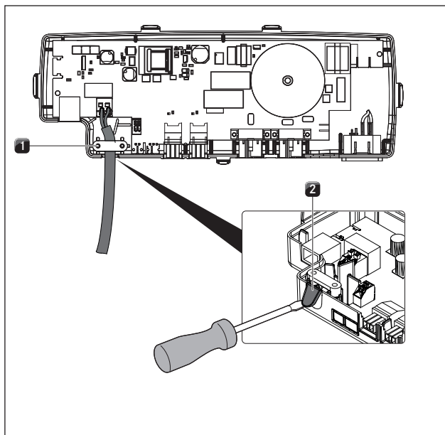
Fig. 4.33 Connexion sur Home Out avec serre-câble
