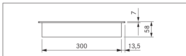
Fig. 3.6 Dimensions CKFI - Vue de devant
