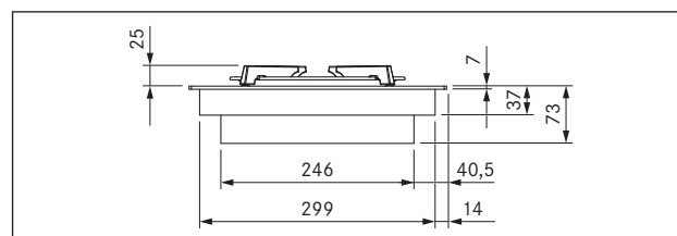
Fig. 3.21 Dimensions CKG - Vue de devant
