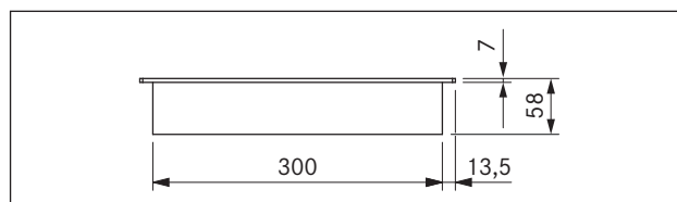
Fig. 3.9 Dimensions CKI - Vue de devant
