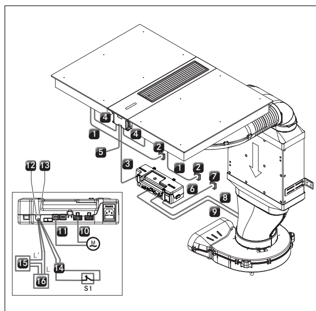
Fig. 4.34 Schéma de raccordement du dispositif aspirant CKA2/CKA2AB
