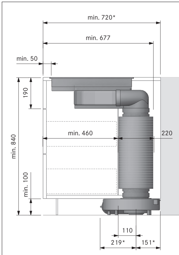
Fig. 4.15 Dimensions de montage de l'appareil avec silencieux rond USDR50
