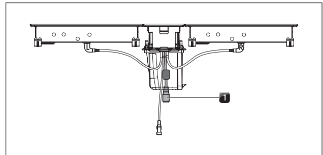
Fig. 4.37 Connecteur pour câble de communication CAT 5e sur l'unité de commande
