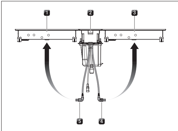
Fig. 4.35 Raccordement des câbles de commande à la table de cuisson
