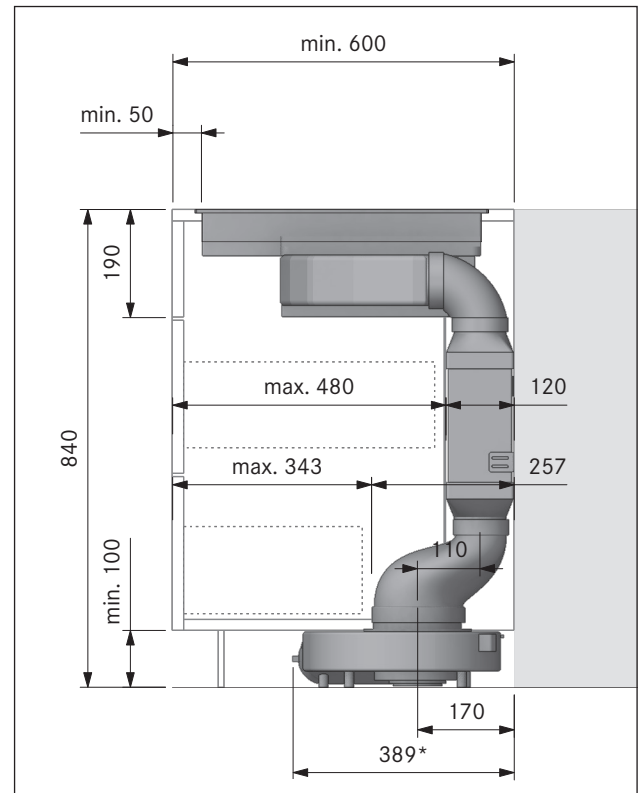
Fig. 4.13 Dimensions de montage de l'appareil avec silencieux plat USDF
