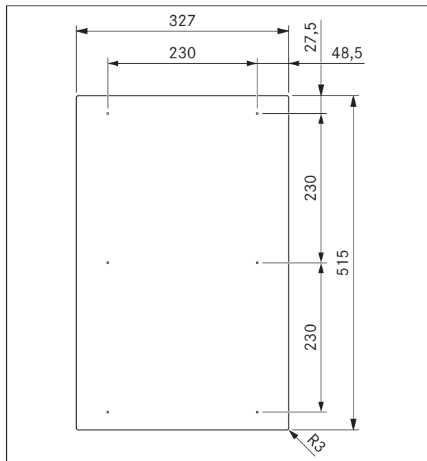
Fig. 3.5 Dimensions CKFI - Vue de dessus
