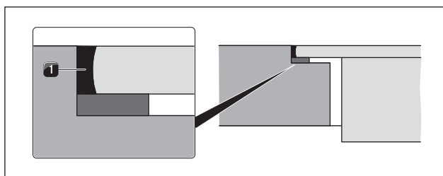
Fig. 4.44 Joint en silicone en montage affleurant
