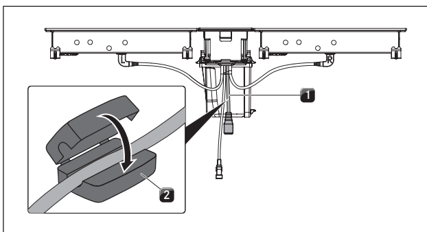
Fig. 4.36 Pose du noyau de ferrite
