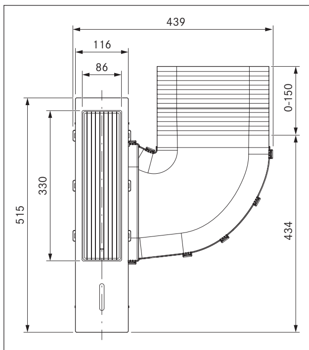
Fig. 3.1 Dimensions CKA2/CKA2AB - Vue de dessus
