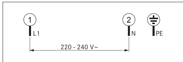
Fig. 4.40 Schéma de raccordement monophasé de la table de cuisson
