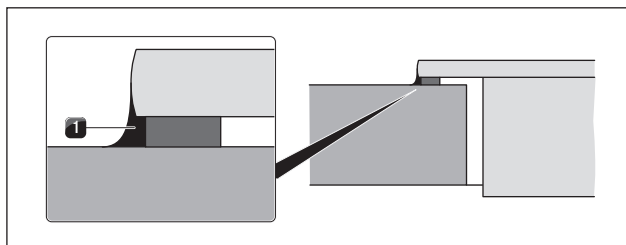
Fig. 4.45 Joint en silicone en montage en saillie
