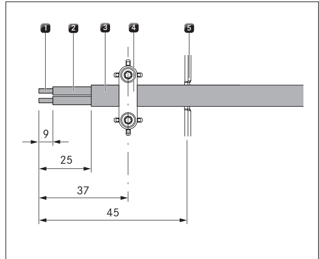
Fig. 4.31 Longueurs de dénudage et position de montage du câble de raccordement
