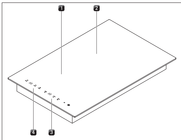
Kuva 4.1 Keittotaso
