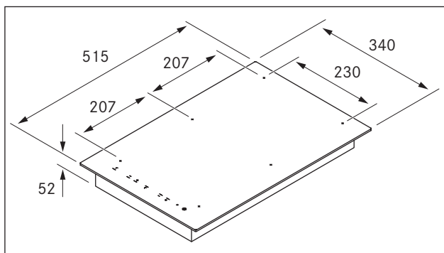
Kuva 3.1 Laitemitat
