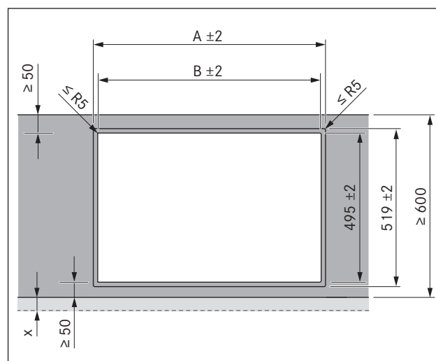
Ilustracja 5.3 Montaż zlicowany
