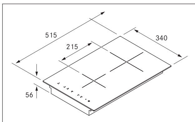
Ilustracja 3.1 Wymiary urządzenia
