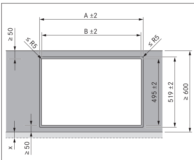
Afb. 5.3 Vlakinbouw
