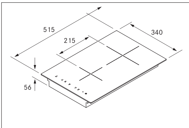
Afb. 3.1 Toestelafmetingen
