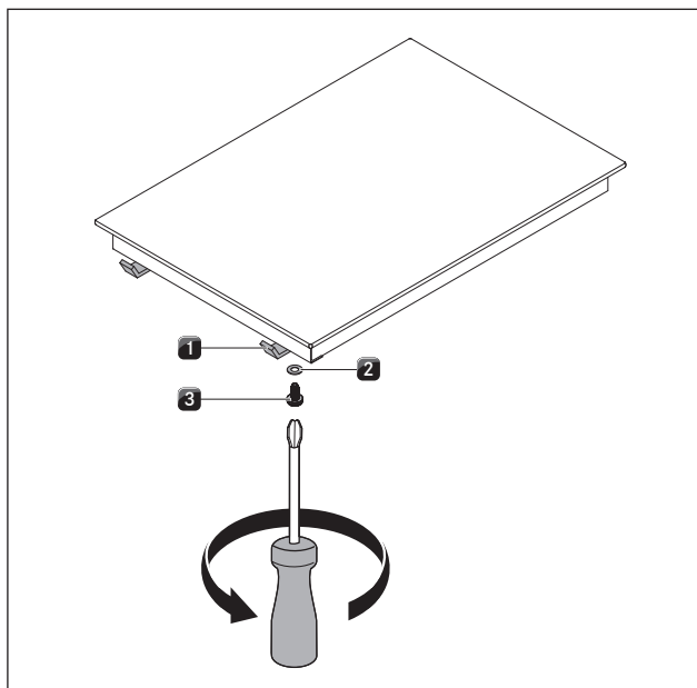
Prikaz 5.11 Montažni nosači
