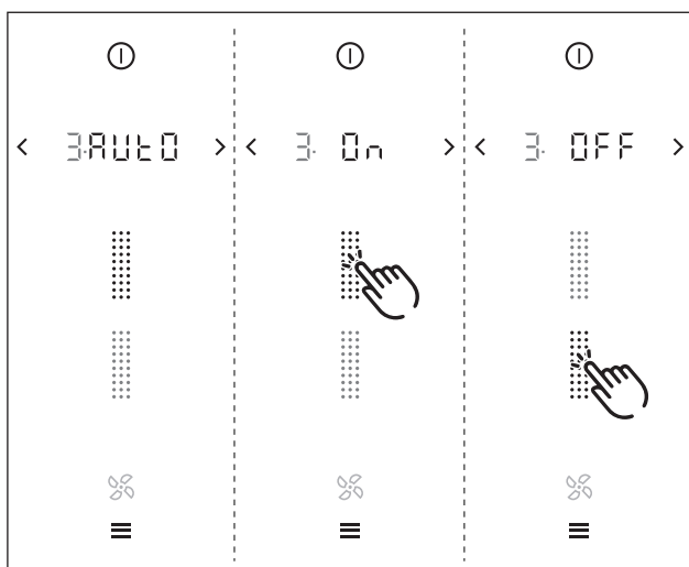
Fig. 7.4 Option de menu 3 : Système d'aspiration automatique
