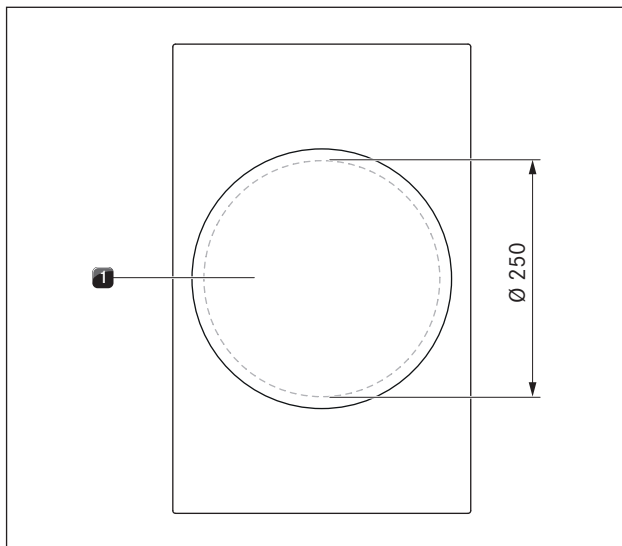
Fig. 4.11 Dimensions de la zone de cuisson
