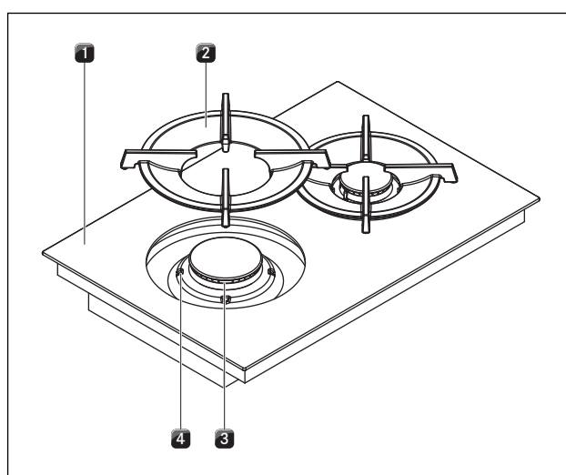
Fig. 9.1 Composition du brûleur à gaz
