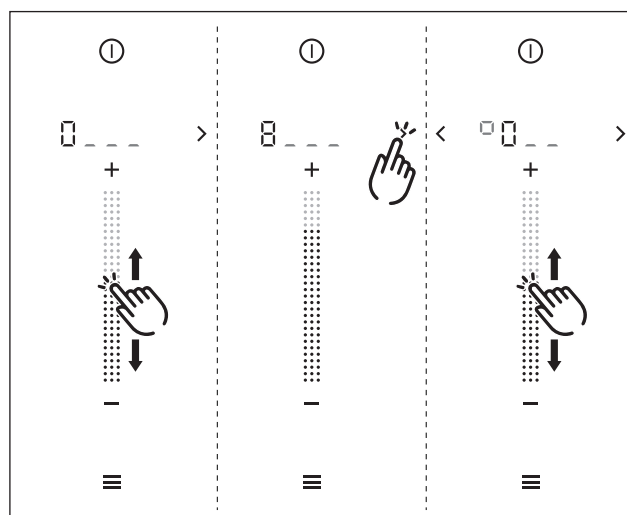
Fig. 8.1 Entrée du code
