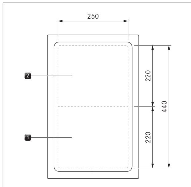
Fig. 4.19 Dimensions des zones de cuisson
