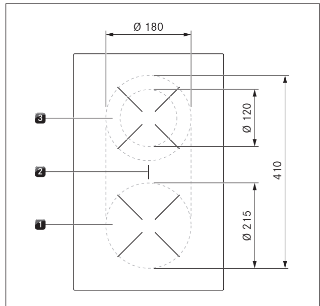
Fig. 4.15 Dimensions des zones de cuisson
