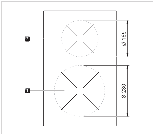
Fig. 4.9 Dimensions des zones de cuisson
