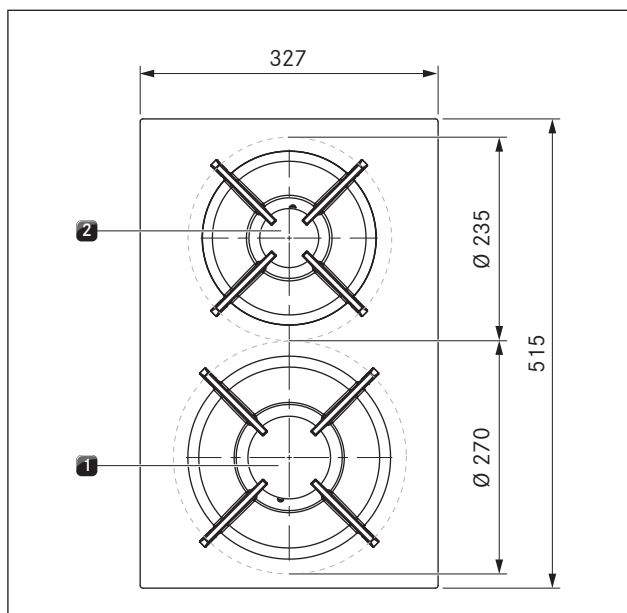
Fig. 4.17 Dimensions des zones de cuisson
