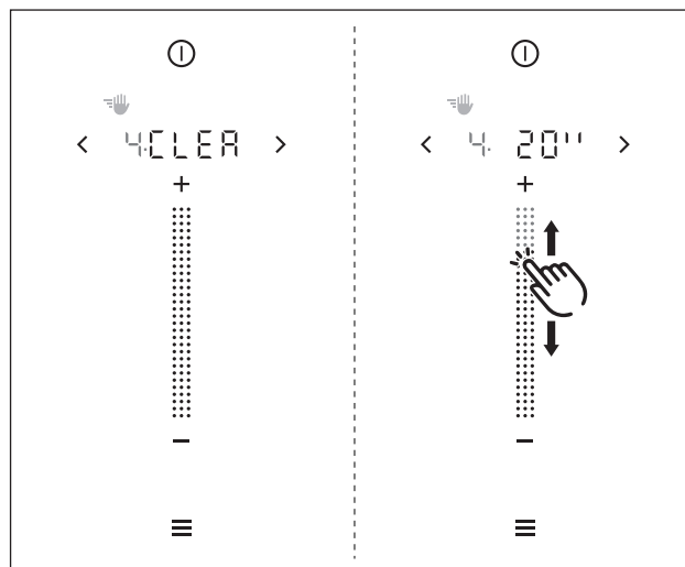
Fig. 7.5 Option de menu 4 : Durée du verrouillage au nettoyage
