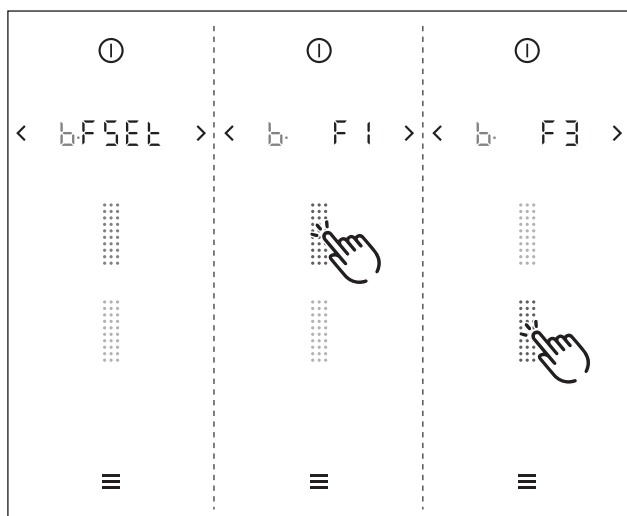
Fig. 7.13 Menupunkt B: Visning af filtertype, omskiftning af filtertype og nulstilling af filterets levetid
