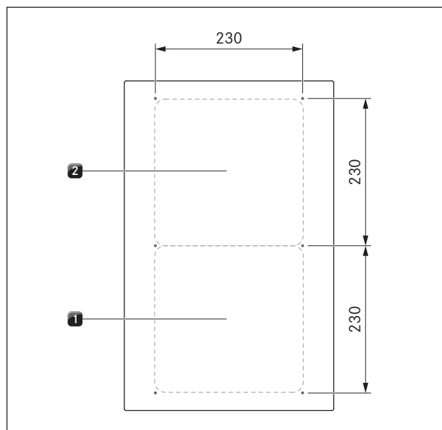
Fig. 4.7 Kogezonernes mål
