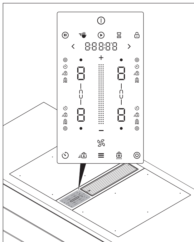
Fig. 4.1 Centralt touch-/skydebetjeningspanel
