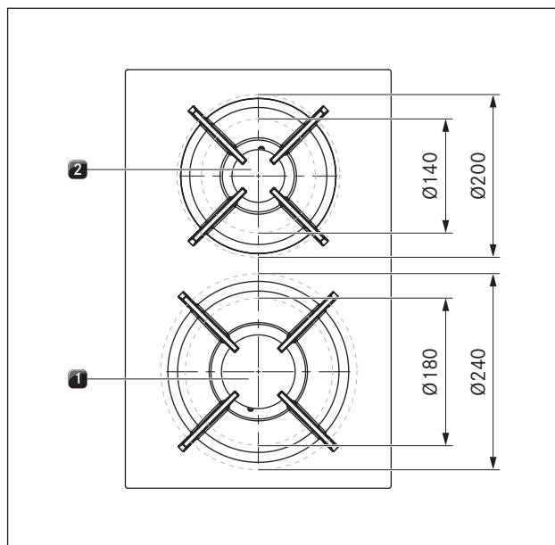
Fig. 4.17 Kogezonernes mål
