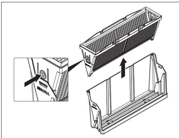
Fig. 9.3 Udtagning af fedtfilter
