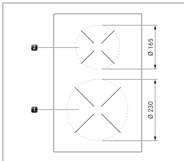
Fig. 4.9 Kogezonernes mål
