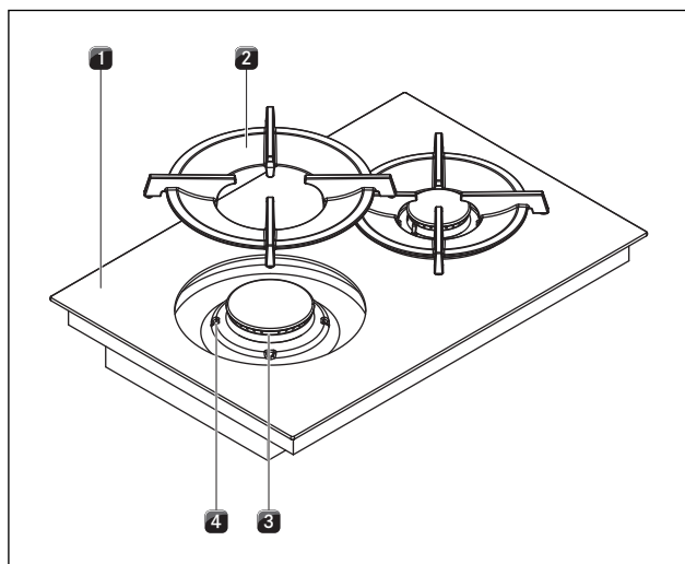
Fig. 9.4 Gasbrænder, opbygning
