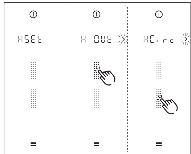
Fig. 5.1 Visning af aftrækssystemets konfiguration
