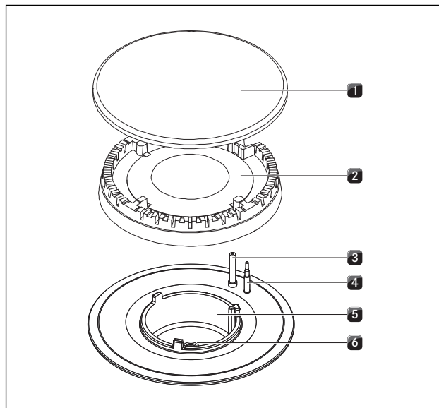
Fig. 9.5 Gasbrænder, opbygning
