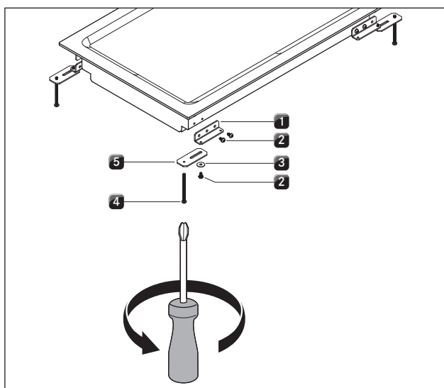
Ilustracja 4.33 Mocowanie grilla Tepan ze stali szlachetnej
