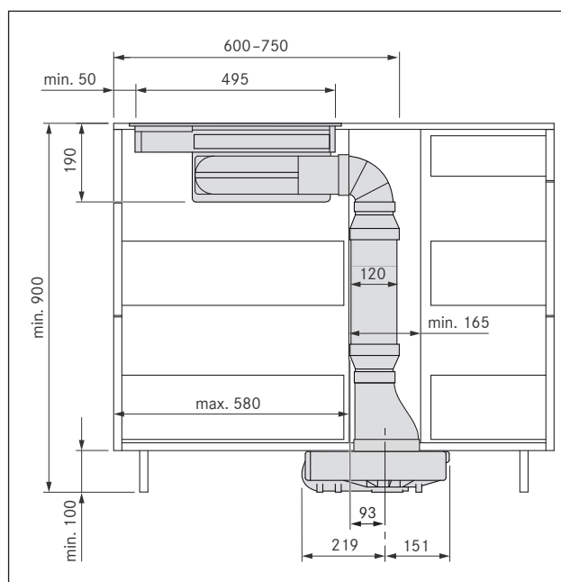
Ilustracja 4.16 Wymiary zabudowy urządzeń z płaskim tłumikiem hałasu USDF przy montażu na wyspie kuchennej
