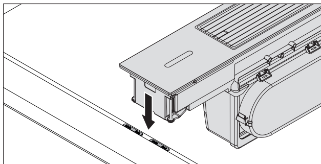
Ilustracja 4.23 Płytki wyrównujące wysokość do montażu z zachowaniem równej powierzchni
