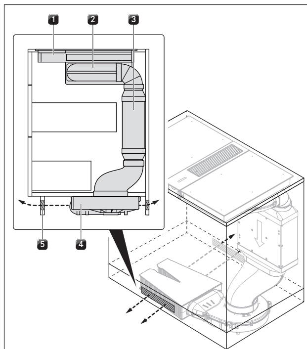
Ilustracja 4.4 Przykład rozplanowania dla powietrza odprowadzanego w obwodzie zamkniętym (wyspa kuchenna + płyta grzewcza + CKA2 + jednostka oczyszczająca powietrze)
