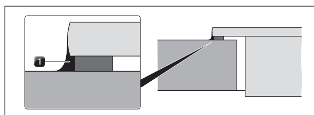
Ilustracja 4.49 Masa silikonowa przy montażu elementu z uskokiem
