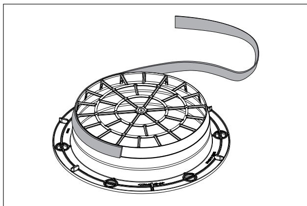
Ilustracja 4.25 Położenie taśmy uszczelniającej do montażu z rurą okrągłą
