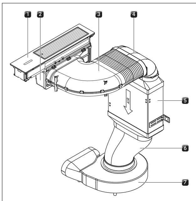
Ilustracja 4.28 Wyciąg oparów CKA2 – budowa standardowa
