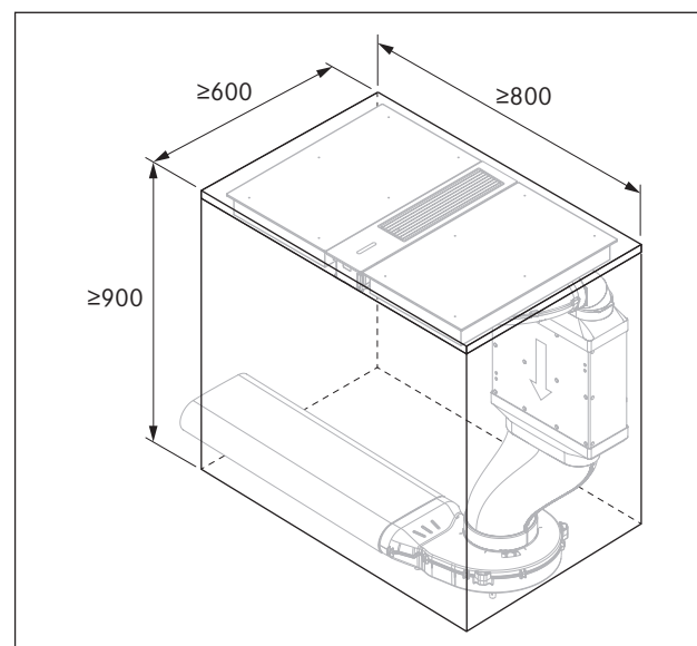
Ilustracja 4.12 Minimalne wymiary zabudowy z płaskim tłumikiem hałasu USDF
