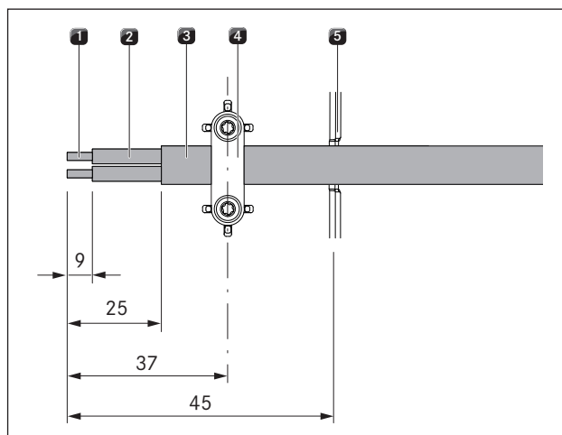
Ilustracja 4.35 Długości izolacji i pozycja montażowa kabla przyłączeniowego
