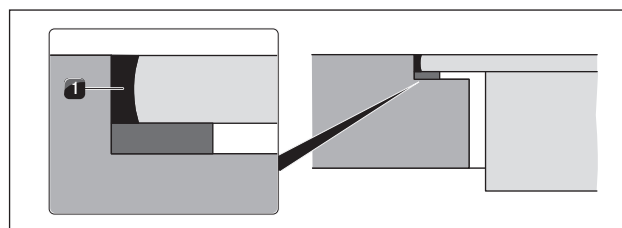
Ilustracja 4.48 Masa silikonowa przy montażu z zachowaniem równej powierzchni
