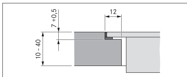
Ilustracja 4.9 Wielkość zakładki przy montażu z zachowaniem równej powierzchni
