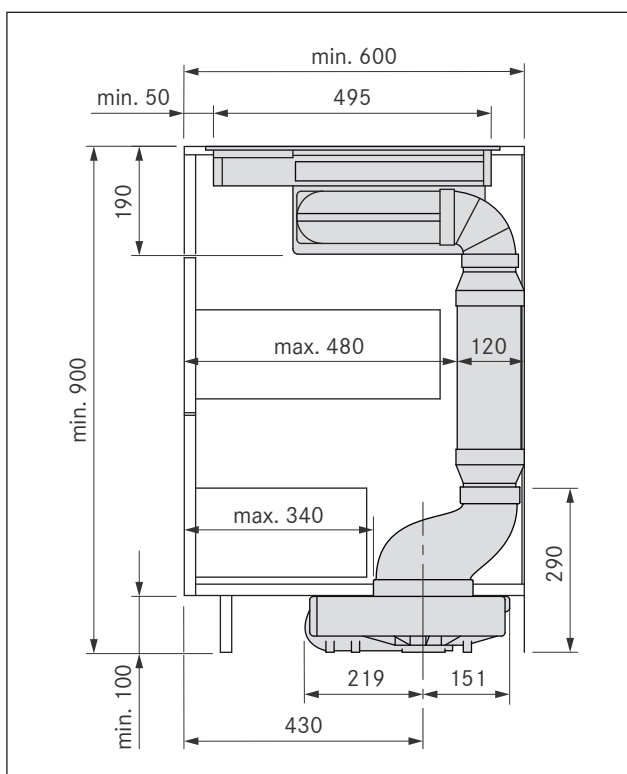
Ilustracja 4.14 Wymiary zabudowy urządzeń z płaskim tłumikiem hałasu USDF przy głębokości korpusu 600 mm
