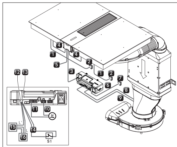
Ilustracja 4.38 Schemat podłączenia wyciągu oparów CKA2
