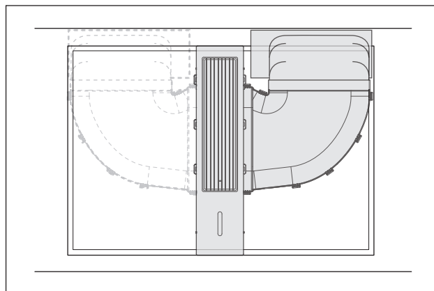
Ilustracja 4.18 Przepływ powietrza do tyłu (w prawo lub w lewo)
