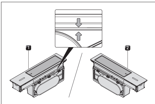
Ilustracja 4.20 Zmontowany wyciąg oparów CKA2
