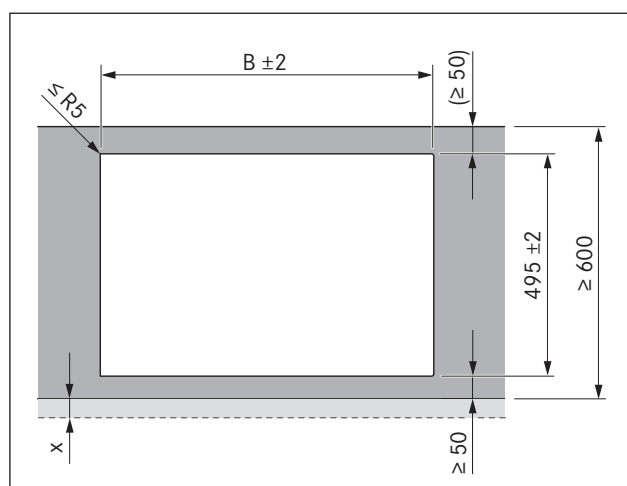
Ilustracja 4.10 Wymiary wycięcia dla montażu z elementu z uskokiem
