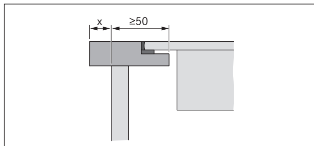
Ilustracja 4.7 Wystający na zewnątrz odcinek blatu
