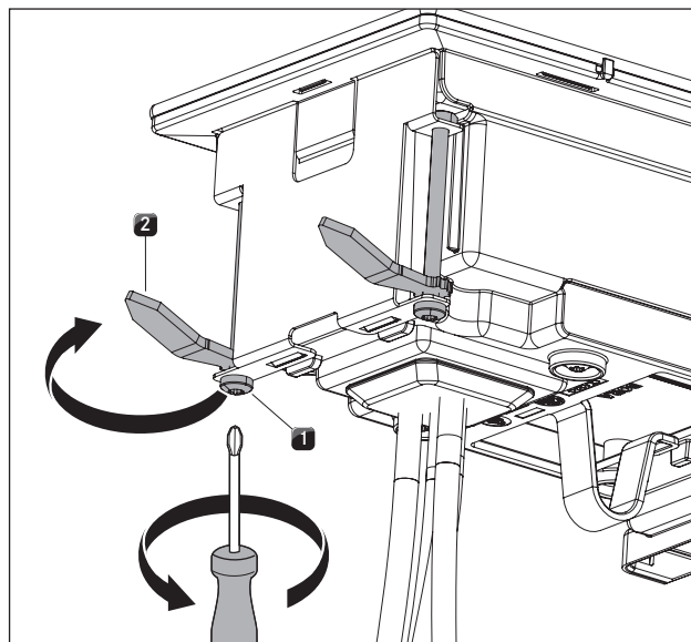
Ilustracja 4.31 Mocowanie wyciągu oparów
