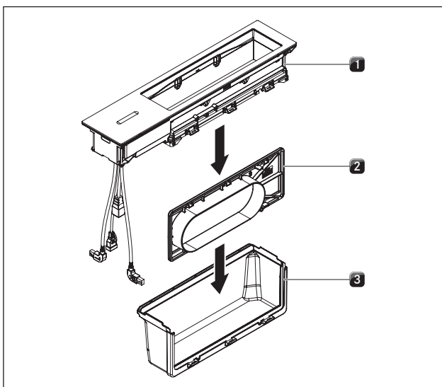
Ilustracja 4.21 Montaż poszczególnych elementów w przypadku wyciągu oparów CKA2
