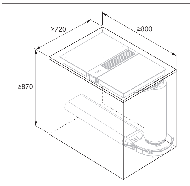
Ilustracja 4.13 Minimalne wymiary zabudowy z okrągłym tłumikiem hałasu USDR50
