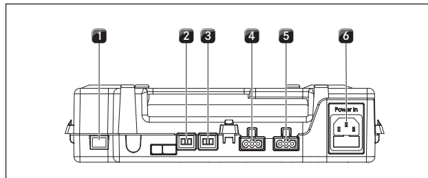
Ilustracja 4.42 Przyłącza jednostki sterującej
