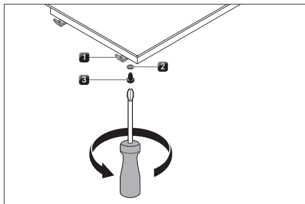
Ilustracja 4.32 Mocowanie płyt grzewczych
