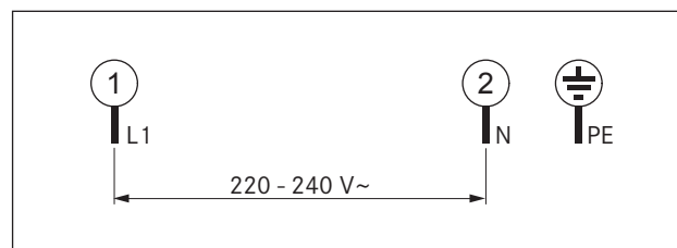
Ilustracja 4.44 Schemat podłączenia, przyłącze 1-fazowe płyty grzewczej
