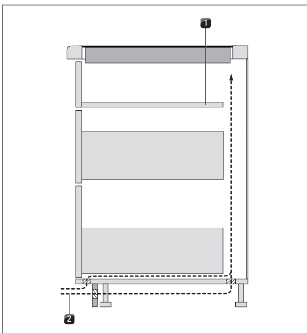
Ilustracja 4.6 Powietrze doprowadzane do obszaru cokołu
