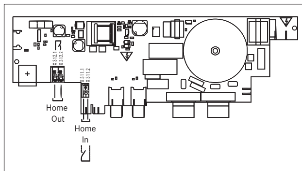
Ilustracja 4.36 Schemat połączeń dla zewnętrznych styków
