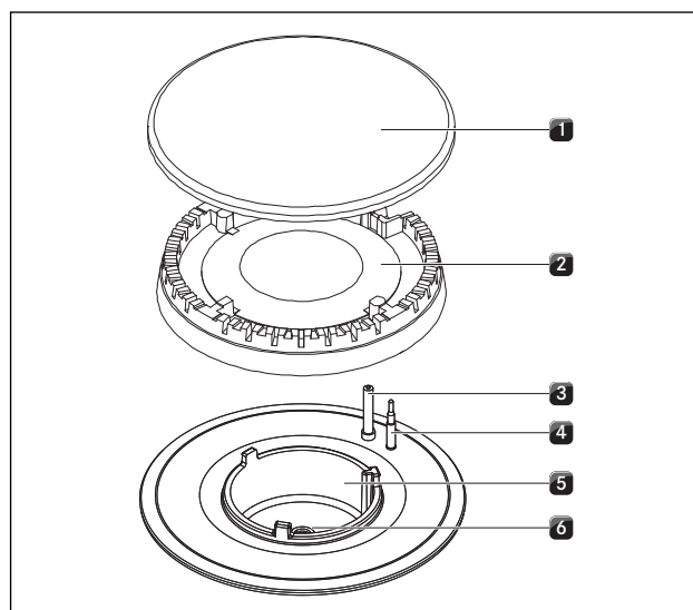
Ilustracja 4.45 Budowa palnika gazowego
