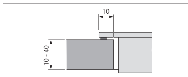
Ilustracja 4.11 Wymiar montażu elementu z uskokiem
