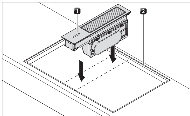
Ilustracja 4.22 Włożyć wyciąg oparów w wycięcie w blacie
