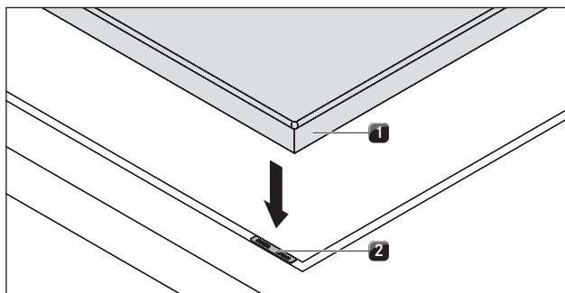
Ilustracja 4.30 Płyta grzewcza i podkładki wyrównujące
