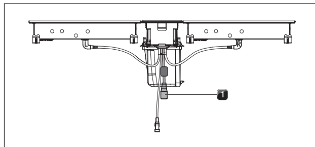
Ilustracja 4.41 Puszka przyłączeniowa dla przewodu komunikacyjnego CAT 5e na jednostce obsługi
