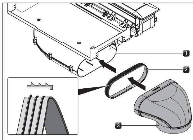
Ilustracja 4.27 Podłączenie do systemu kanałów
