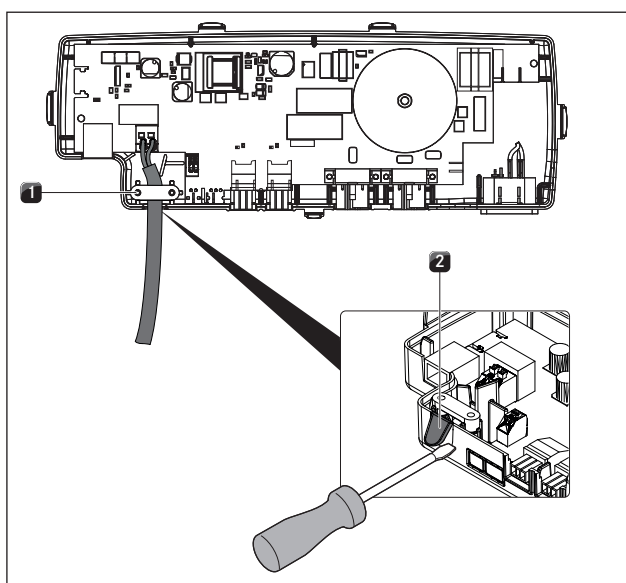
Ilustracja 4.37 Styk Home-Out z odciążeniem
