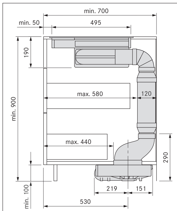
Ilustracja 4.15 Wymiary zabudowy urządzeń z płaskim tłumikiem hałasu USDF przy głębokości korpusu 700 mm
