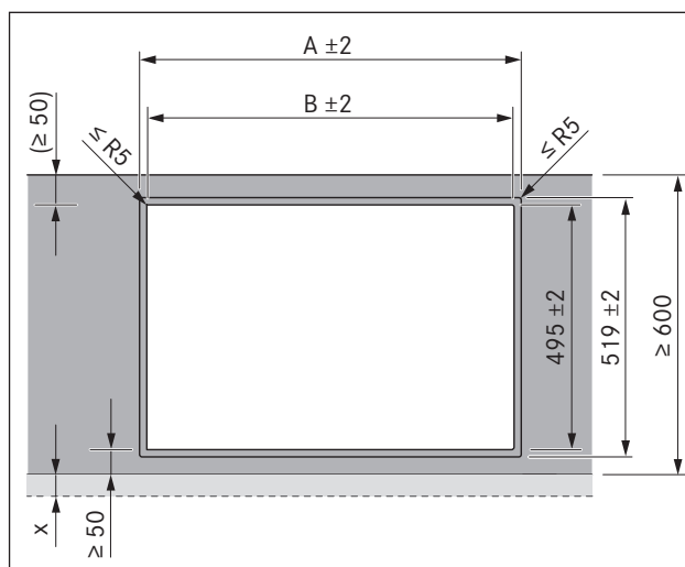
Ilustracja 4.8 Wymiary wycięcia dla montażu z zachowaniem równej powierzchni
