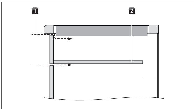
Ilustracja 4.5 Powietrze doprowadzane do korpusu z przodu
